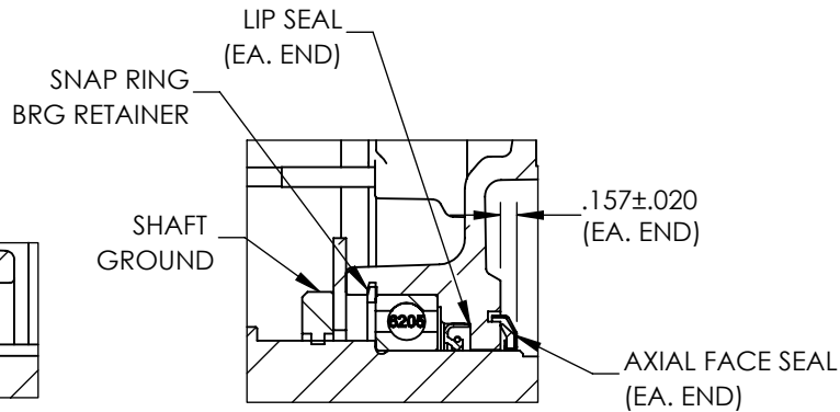
PU END DETAIL
