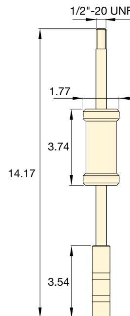
Dimensiones del martillo deslizante (pulg)
