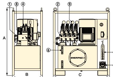
Serie SFP con depósito de 40 galones (mostrado aquí con 4 salidas de flujo dividido)
