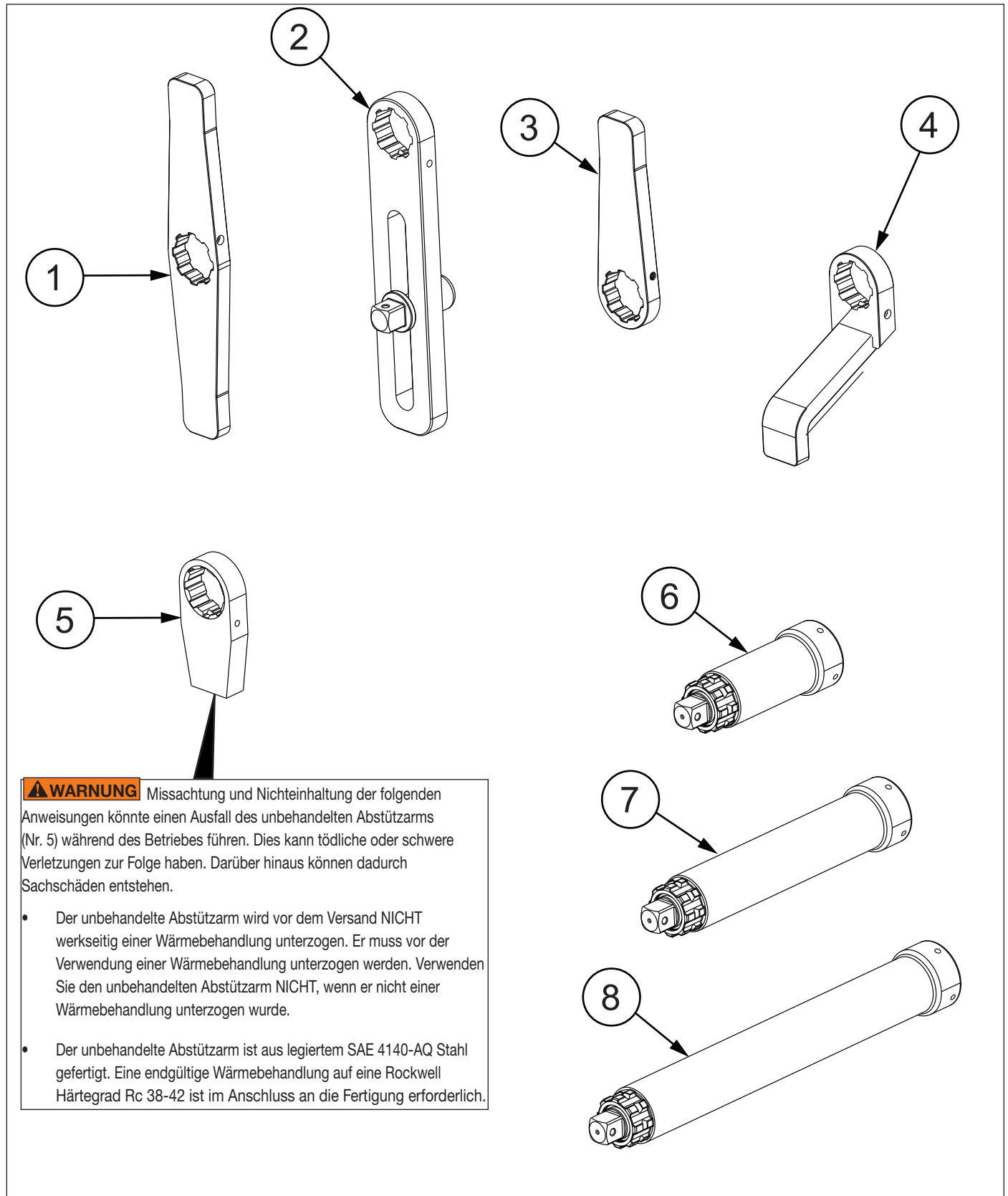
Abbildung 14: Zubehör
