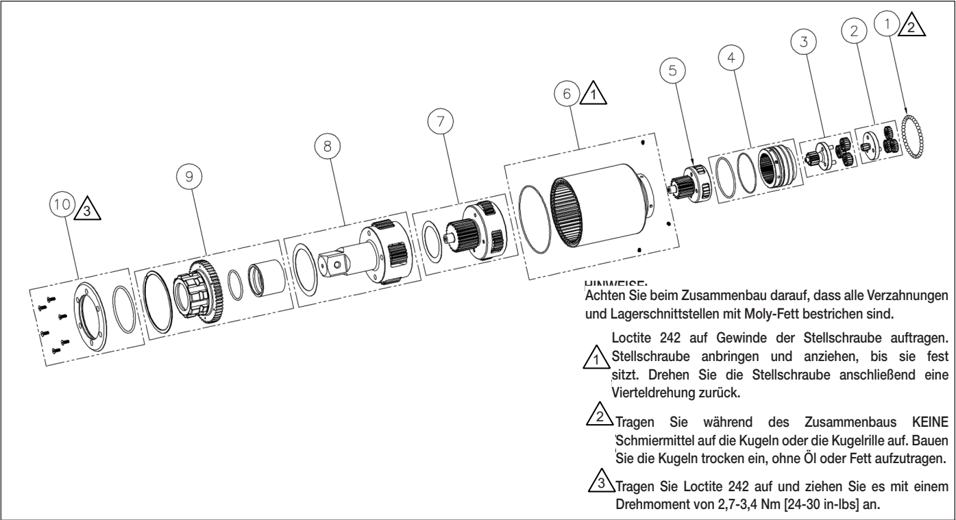
Abbildung 13: TW6000SR Getriebe-Baugruppe
