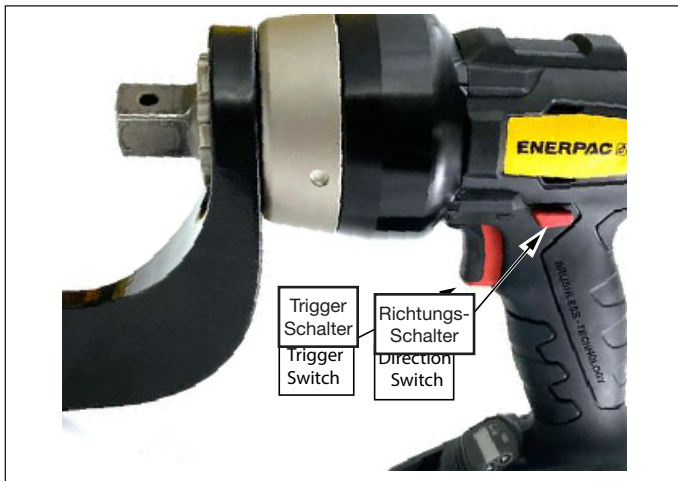
Abbildung 5: Trigger Schalter
