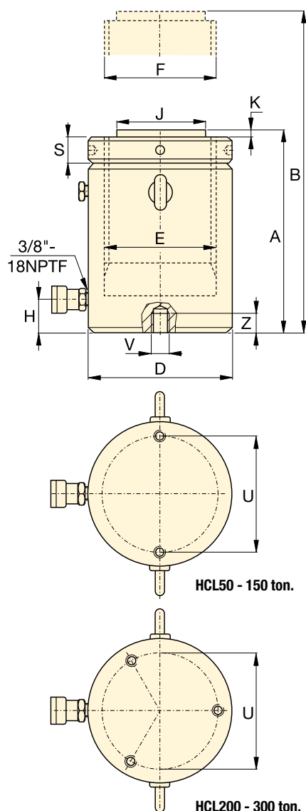
HCL200 - 300 ton.
