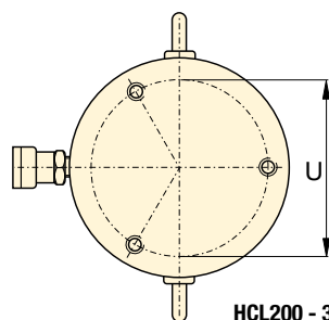
HCL200 - 300 tonnes
