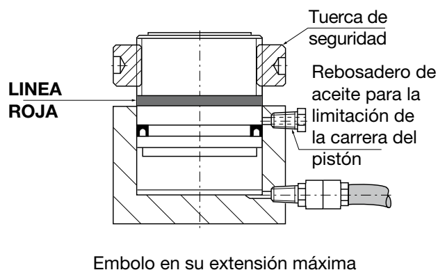
Ilustración 1 - Cilindros CLP
