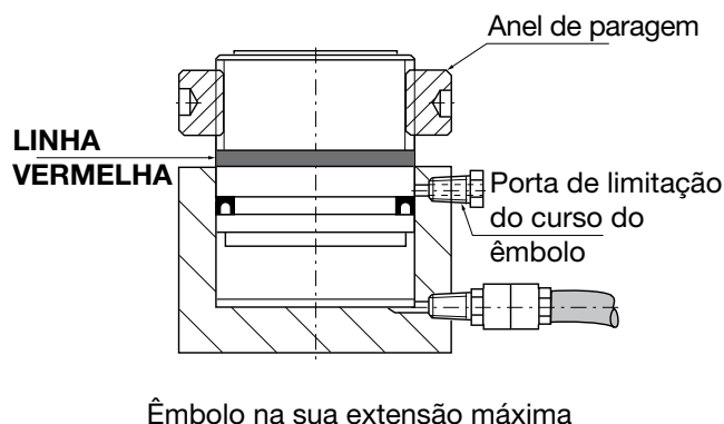
Figura 1 - Cilindros CLP
