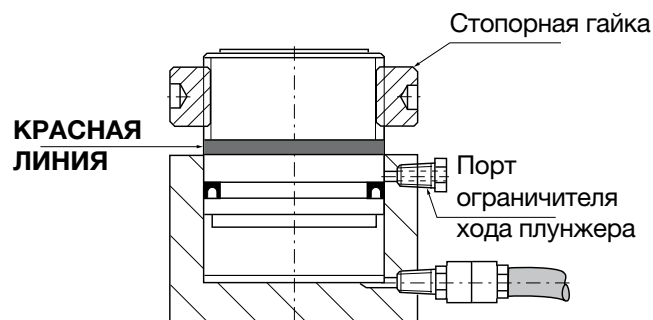
Рис. 1 - Цилиндры серии CLP
