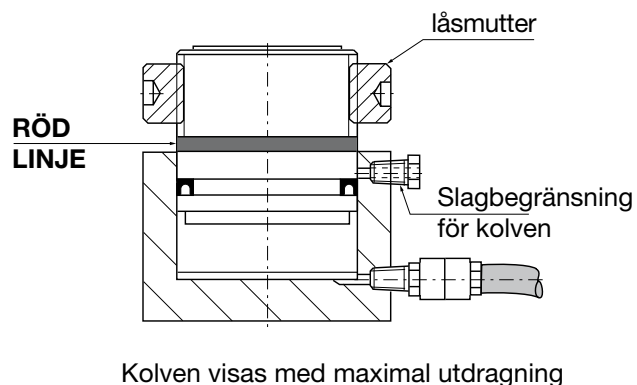
Bild 1 - CLP-cylindrar
