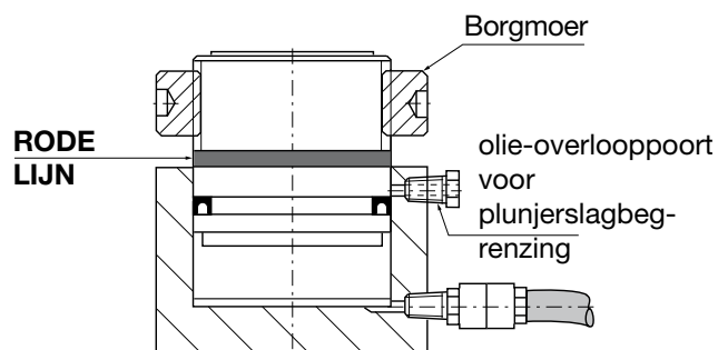
CLP cilinder, afgebeeld met maximale plunierslag
