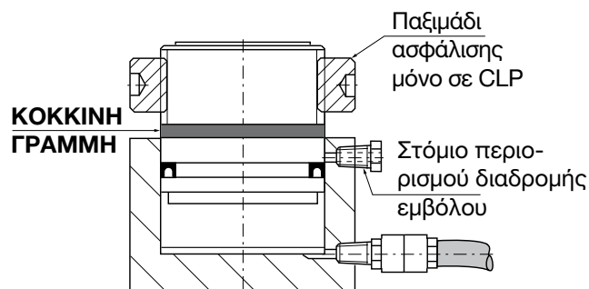
εικόνα 1 - Κύλινδροι CLP
