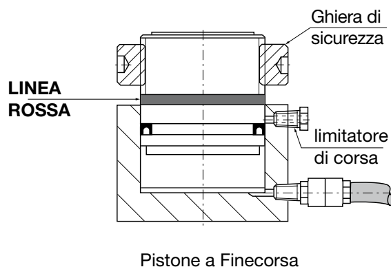
Illustrazione 1 - cilindri CLP
