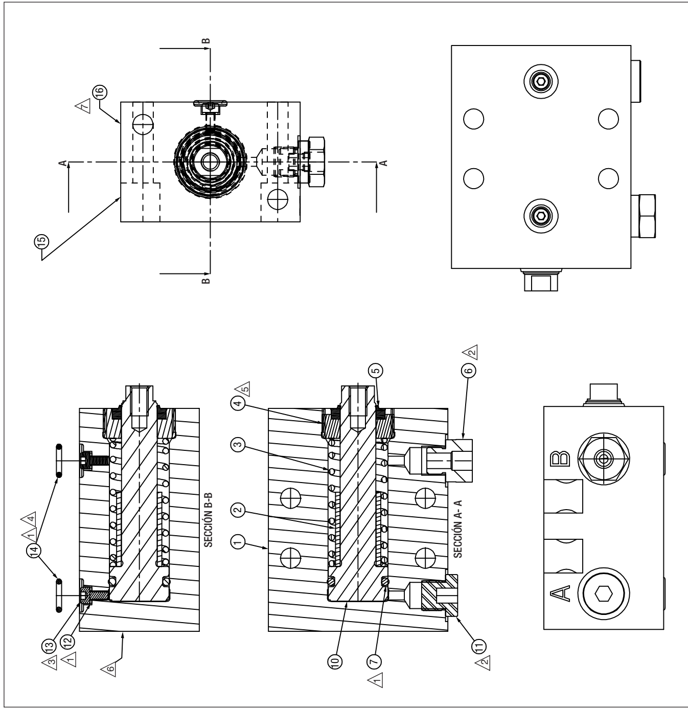
Figura 1: Conjunto del cilindro - Serie CSB
