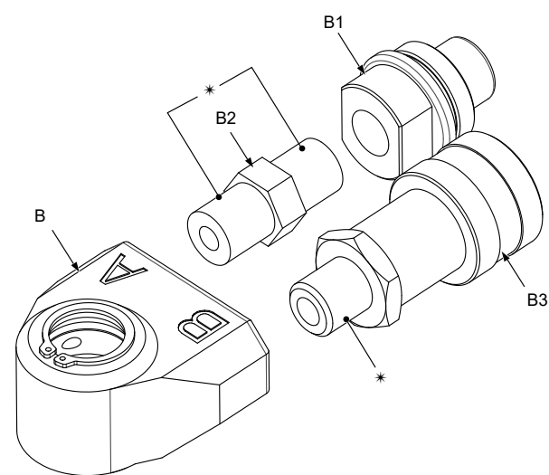
Figuur 12: Opengewerkte tekening van koppelsset
