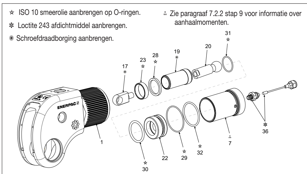
Figuur 13: Opengewerkte tekening van DSX1500, DSX3000, DSX5000 pluimers
