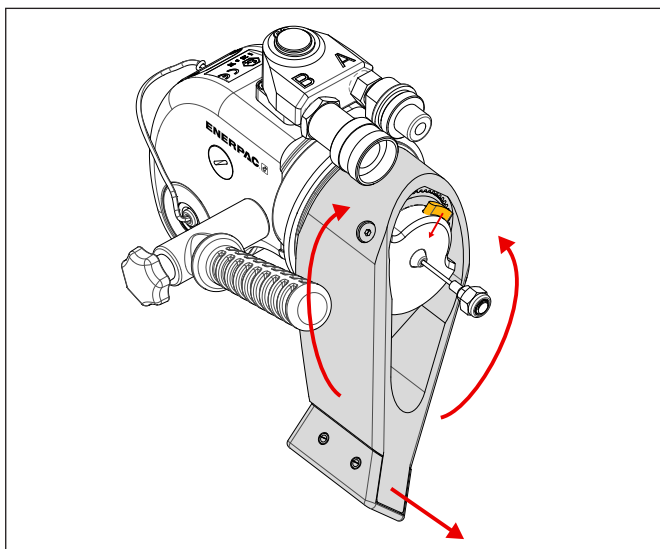
Figuur 4: Reactiearm positioneren
