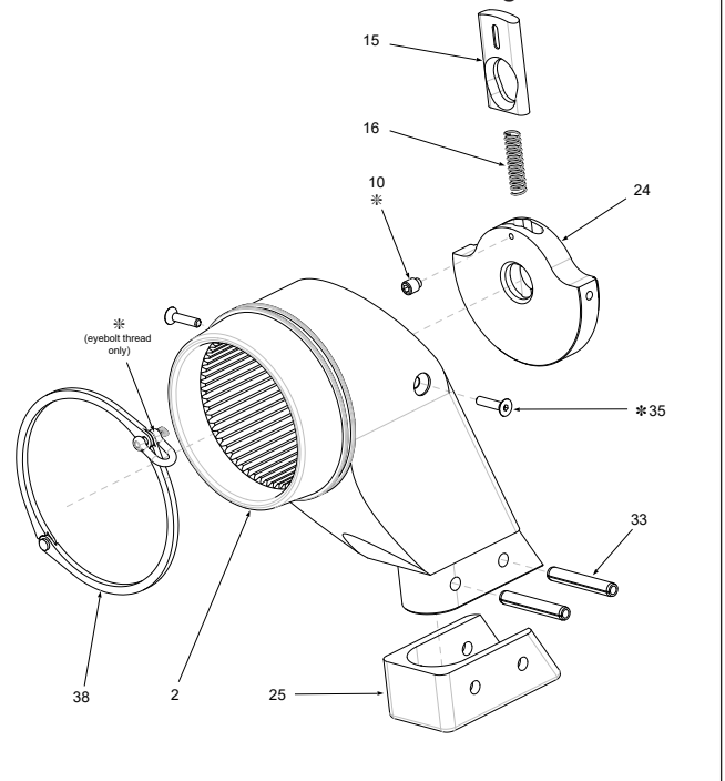
Figuur 16: Opengewerkte tekening van reactiearm
