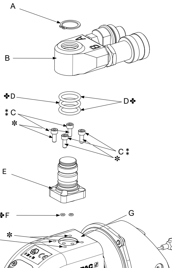
Figuur 11: Koppelsstang en koppelsset
