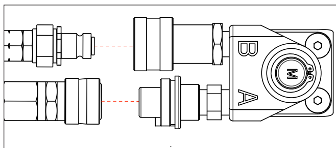
Figuur 6: Richting van aandrijving wijzigen
