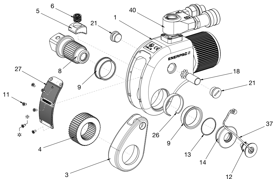
Figuur 9: Opengewerkte tekening van momentsleutelkop
