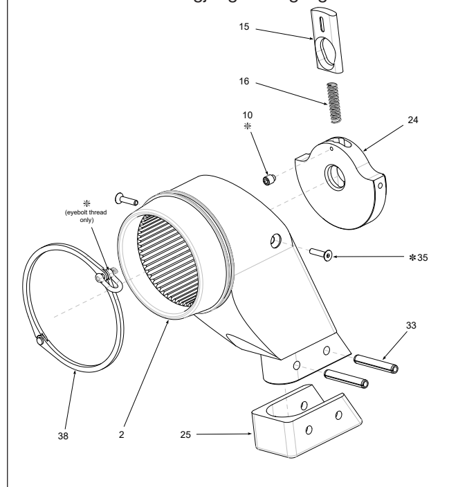
Figur 16: Oversiktstegning for reaksjonsarm
