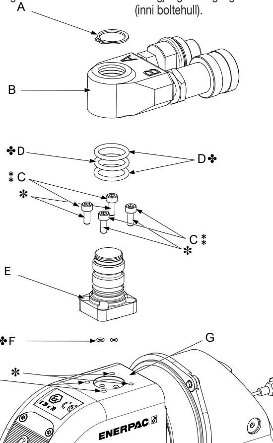
Figur 11: Montering av svingbolt og svivelenhet
