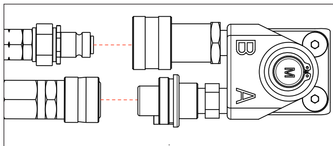
Figur 6: Endre drivretning
