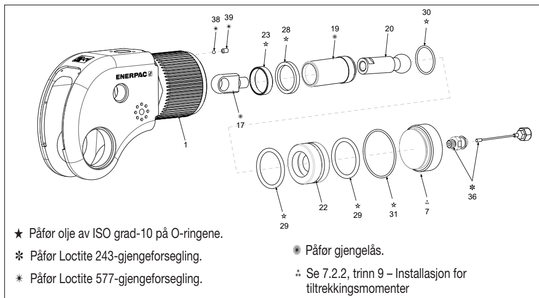
Figur 14: Oversiktstegning for DSX11000- og DSX25000-stempler
