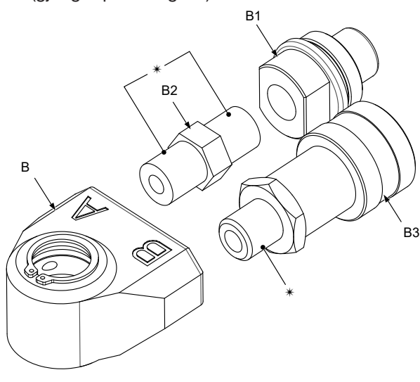
Figur 12: Oversiktstegning for svivelenhet
