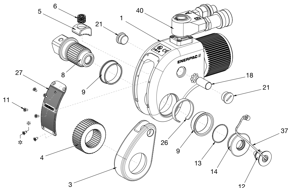
Figura 9: Cabeza de la llave dinamométrica en despiece
