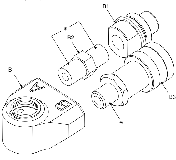
Figura 12: Despiece de la unidad giratoria
