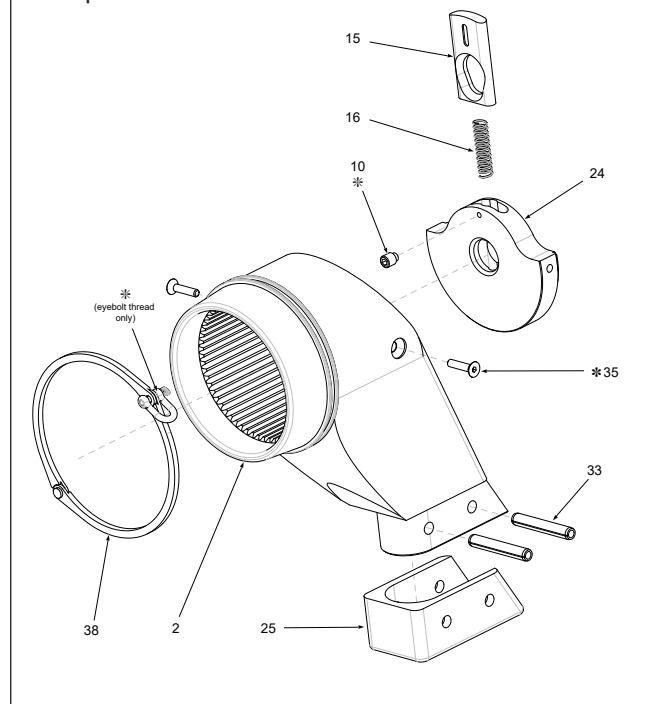
Figura 16: Brazo de reacción en despiece
