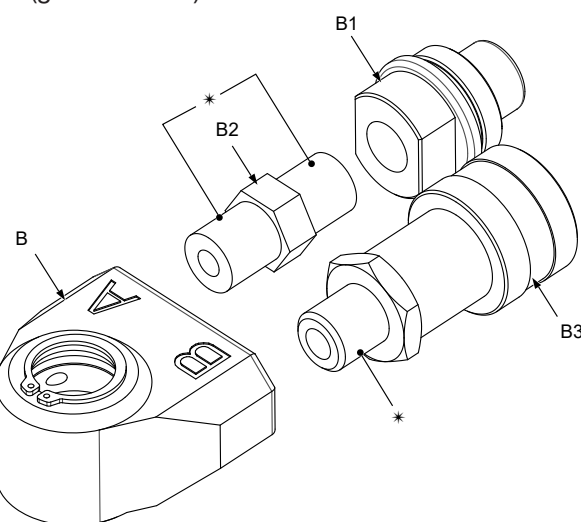
Rysunek 12: Rozłożony zespół przegubu
