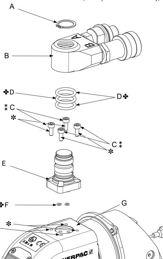
Rysunek 11: Podstawa przegubu i zespół przegubu
