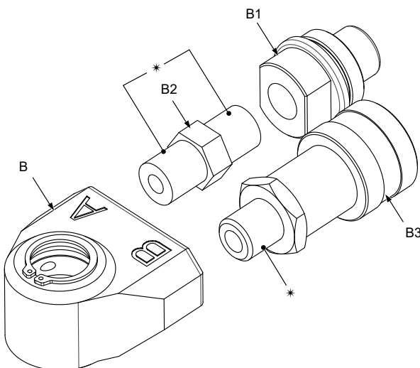
Figure 12 : vue éclatée du montage du raccord tournant
