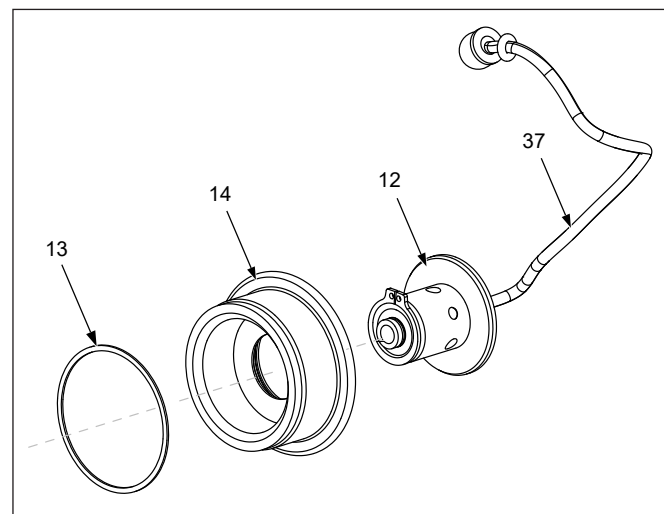
Figure 17 : Vue éclatée du carré conducteur
