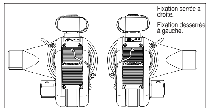
Figure 3 : sens du carré conducteur pour le desserrage/serrage
