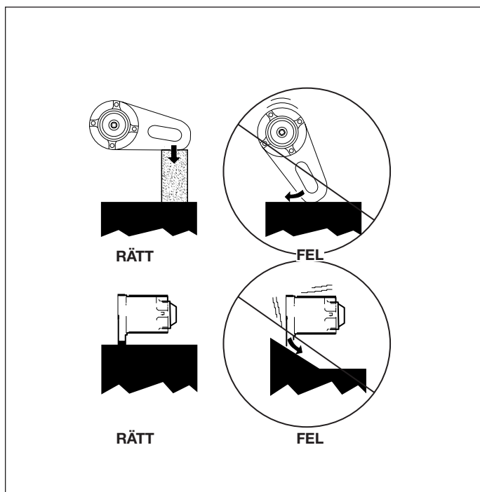
Fig. 7, Håll reaktionsankaret i rätt vinkel mot reaktionspunkten.
