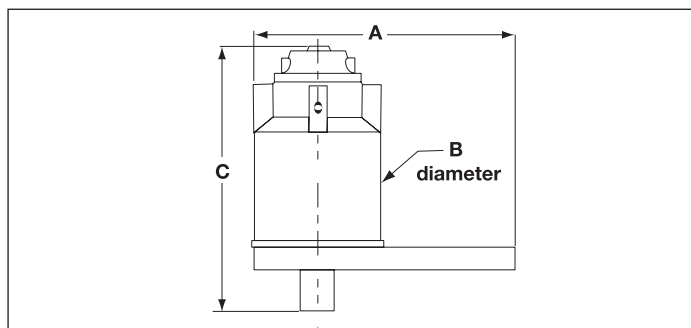
Figura 2, Dimensioni moltiplicatore di coppia
