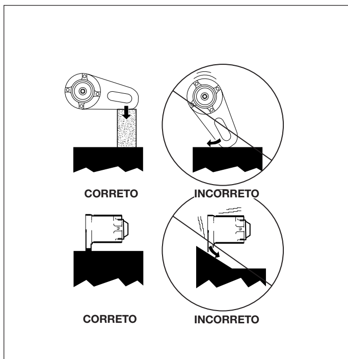
Fig. 7, Mantenha a âncora de reação perpendicular ao ponto de reação
