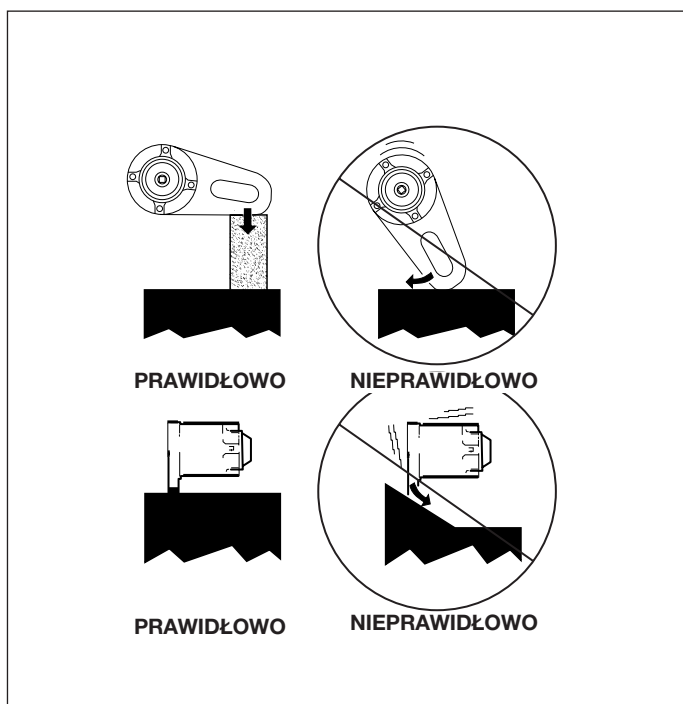
Rys. 7, Mocujący element reakcyjny należy utrzymywać w położeniu prostopadłym do punktu reakcyjnego.
