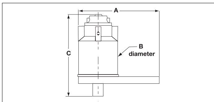
Fig. 2, Momentmultiplikatorns dimensioner
