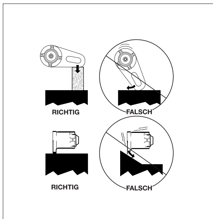
Abb. 7, Halten Sie den Reaktionsanker im rechten Winkel zum Reaktionspunkt.
