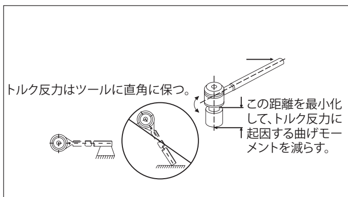
図6 - トルクマルチプライヤーの反力による曲げモーメントの最小化
