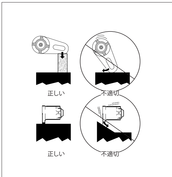
図7 - 反力支持部は、反力作用点に対して直角に配置する
