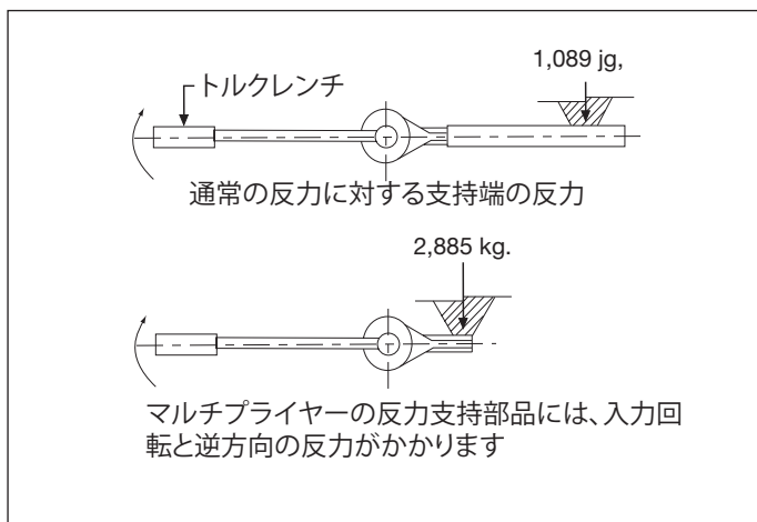
図5 - マルチプライヤーに近いほど反力は大きい
