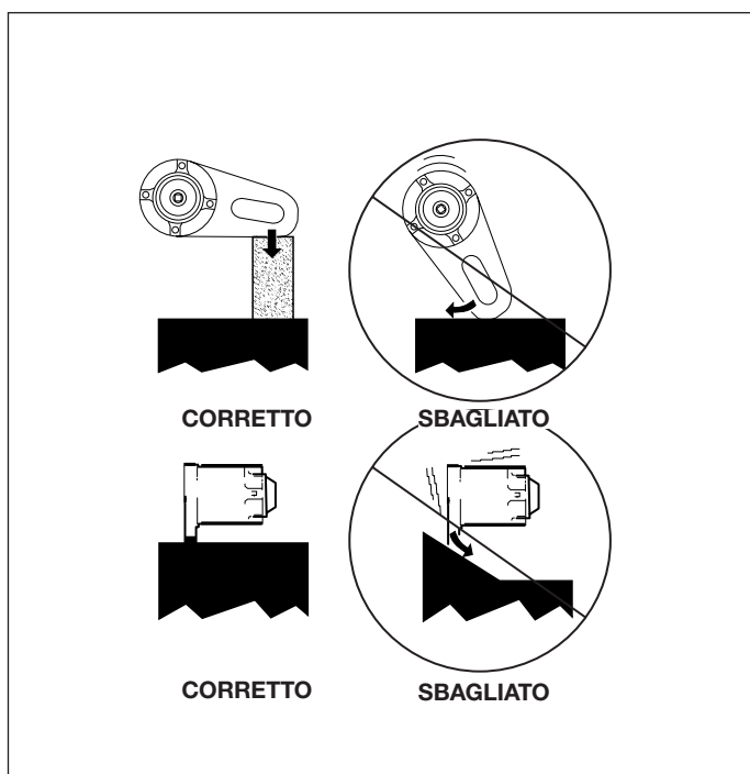
Figura 7, Mantenere l'ancora di reazione perpendicolare la punto di reazione
