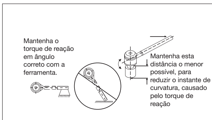
Fig. 6, Minimize os instantes de curvatura criados pelo torque de reação do multiplicador.
