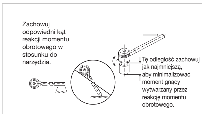
Rys. 6, Minimalizowanie momentów gnących wytworzonych wskutek działania wzmocniacza momentu obrotowego
