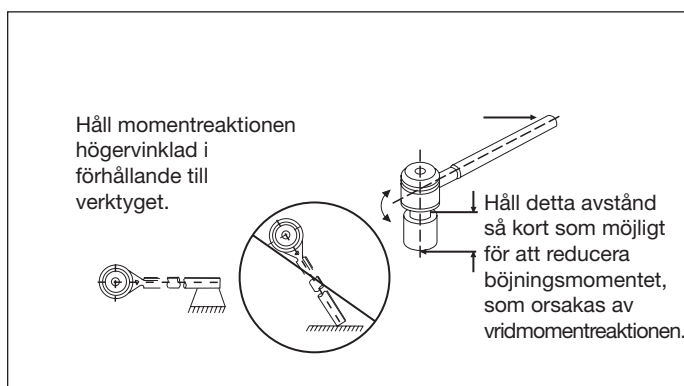
Fig. 6, Begränsa böjningsmomenten som skapas av momentmultiplikatorns reaktion
