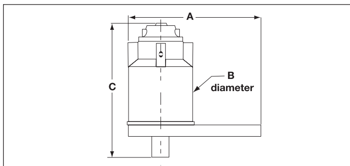
図2 - トルクマルチプライヤー寸法
