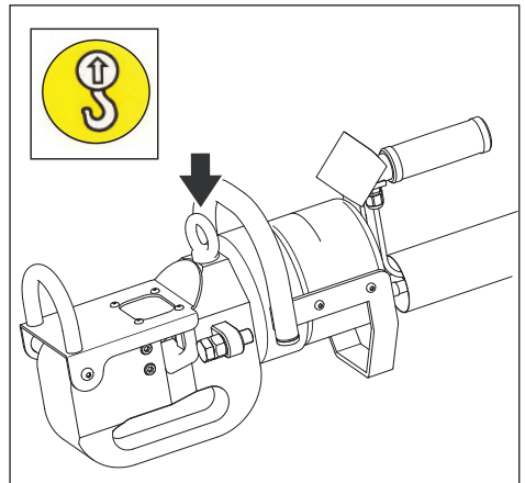
Figuur 7. Hijslocatie van knipper
