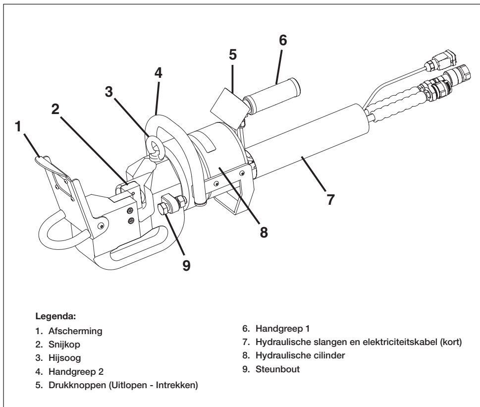
Figuur 1. Functies en onderdelen
