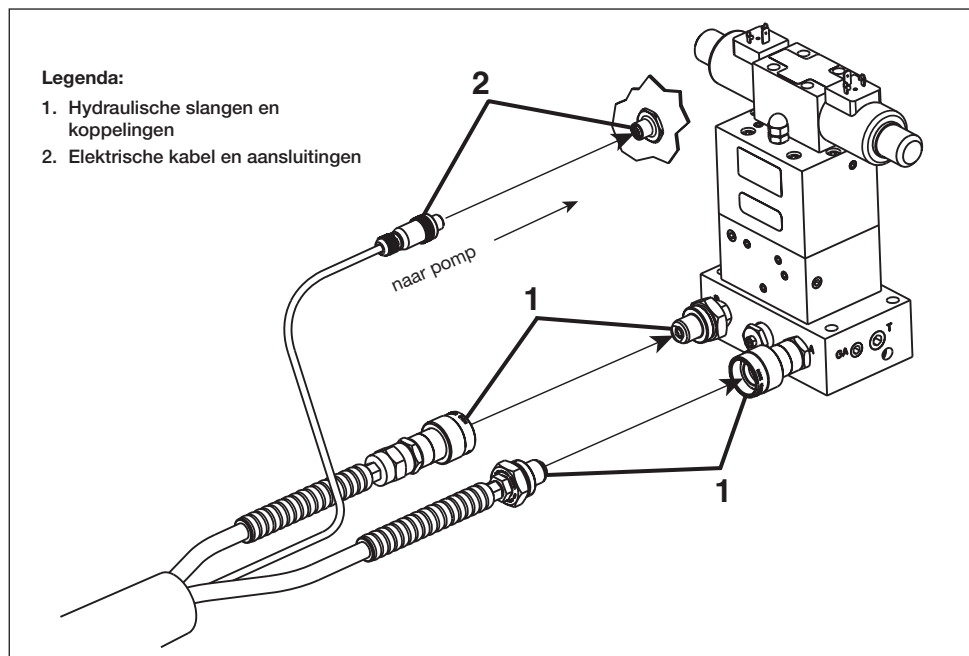
Figuur 3. Hydraulische en elektrische aansluitingen op pomp
