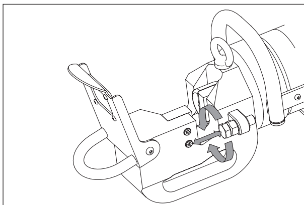
Figuur 10. De steunbout bijstellen
