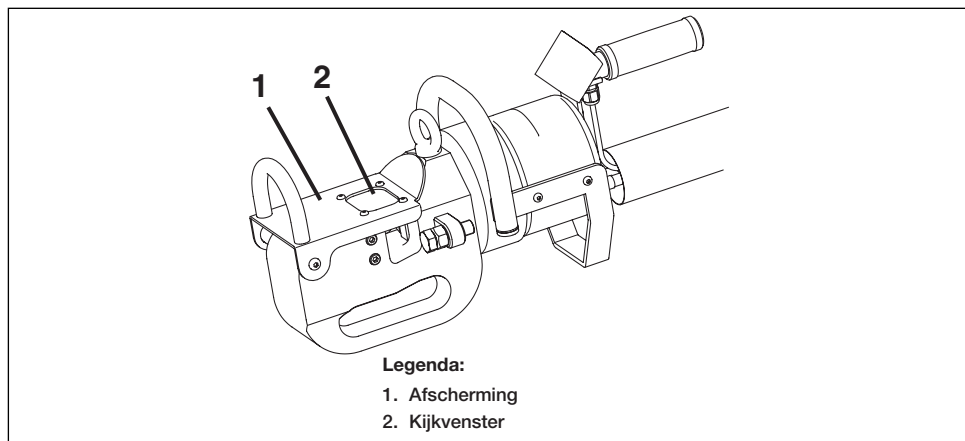
Figuur 4. Afscherming met kijkvenster
