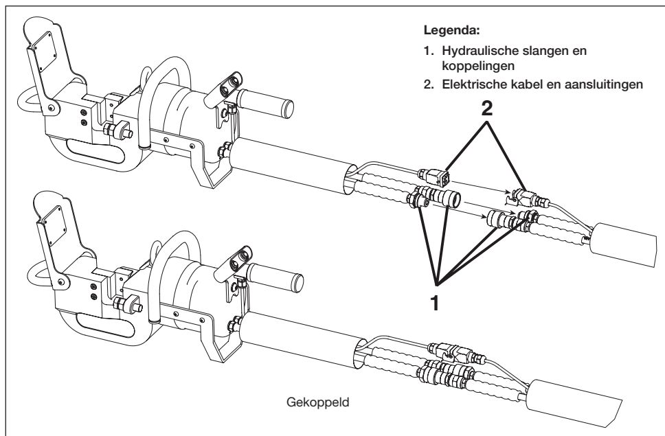
Figuur 2. Hydraulische en elektrische aansluitingen op knipper (voorbeeld)
