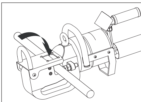
Figuur 6. Afscherming sluiten
