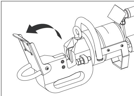
图 5，打开安全防护装置
