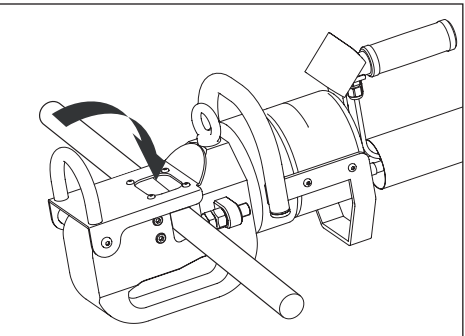
图 6，关闭安全防护装置
