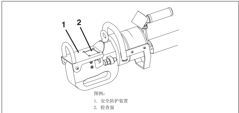
图 4，带检查窗的安全防护装置
