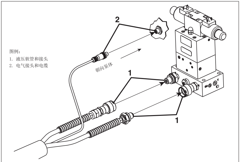
图 3，泵站处的液压和电气连接
