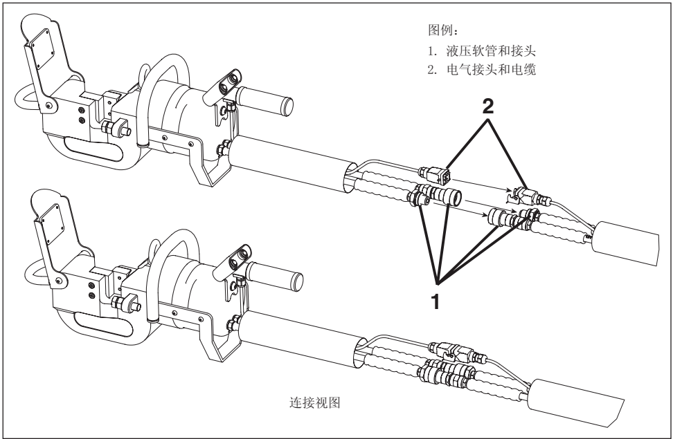
图 2，切断机处的液压和电气连接（典型）
