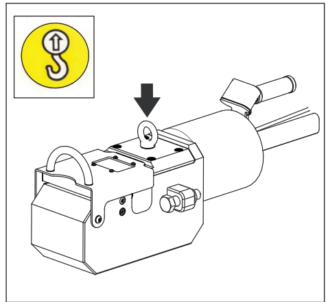
Abbildung 7, Anhebestelle
