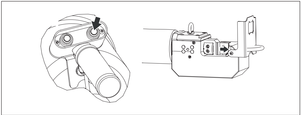
Abbildung 11, Betrieb - Ausfahren/Schneiden
