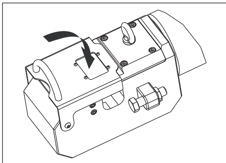
Abbildung 6, Schutzvorrichtung schließen
