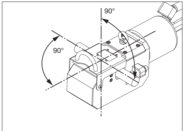
Abbildung 9, Positionierung des Materials im Schneidkopf
