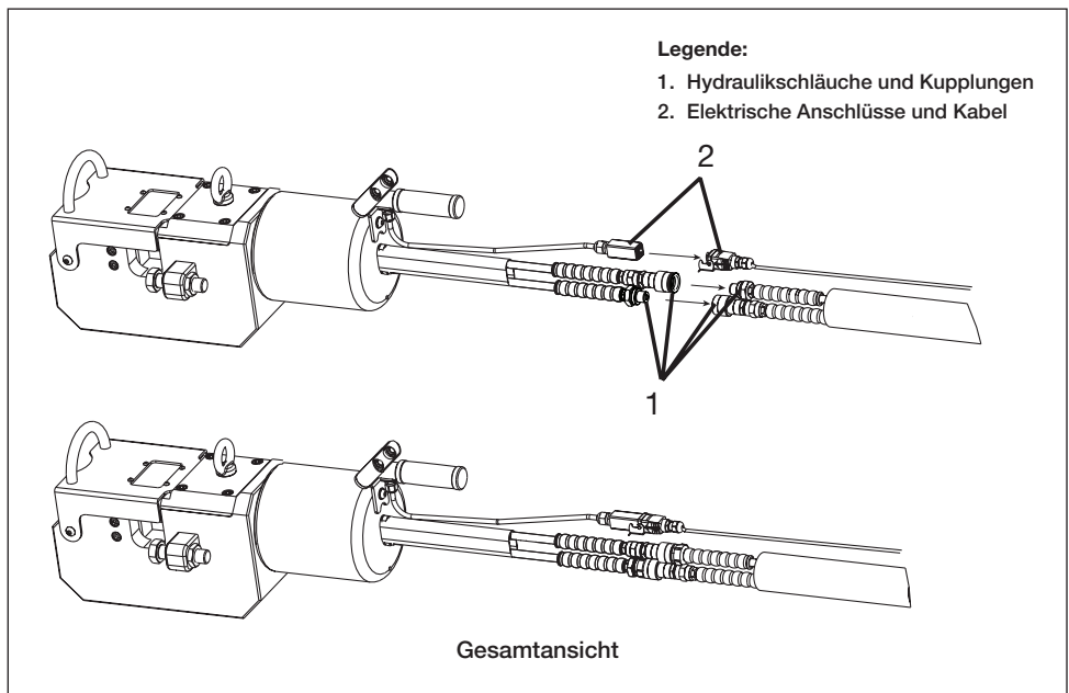
Abbildung 2, Hydraulik- und Elektroanschlüsse am Schneidgerät (typisch)
