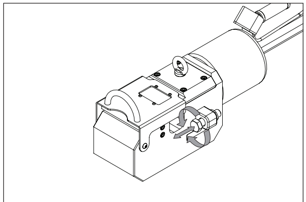
Abbildung 10, Einstellung des Stützbolzens
