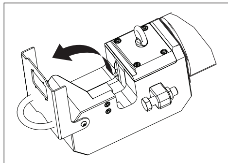
Abbildung 5, Schutzvorrichtung öffnen
