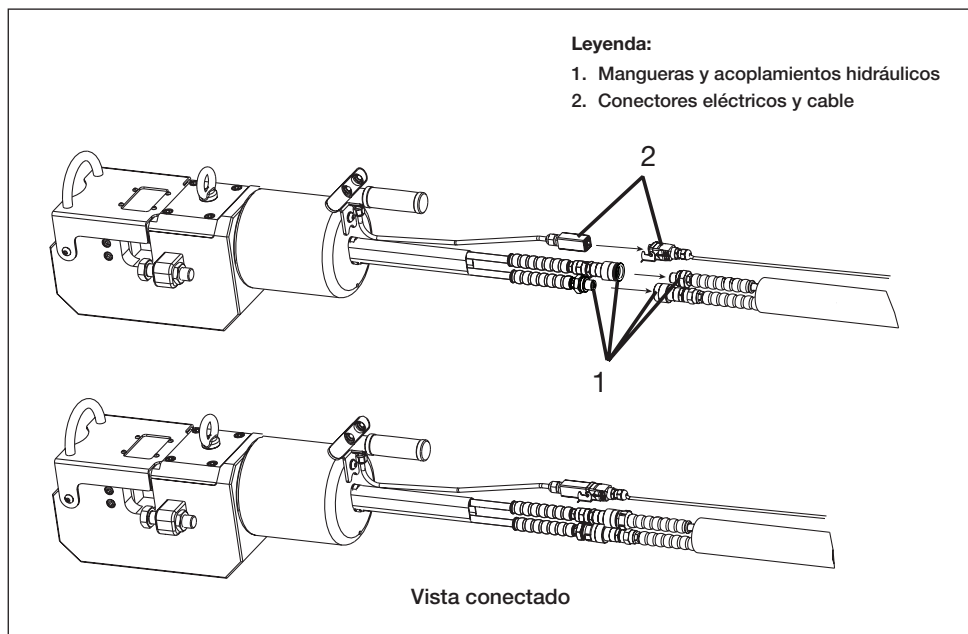
Figura 2, Conexiones hidráulicas y eléctricas en el cortabarras (típico)
