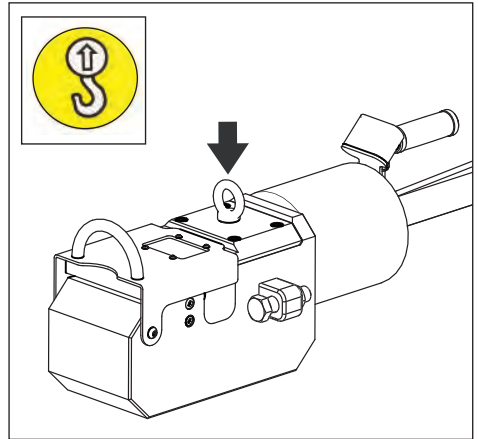
Figura 7, Ubicación del asa de elevación del cortabarras
