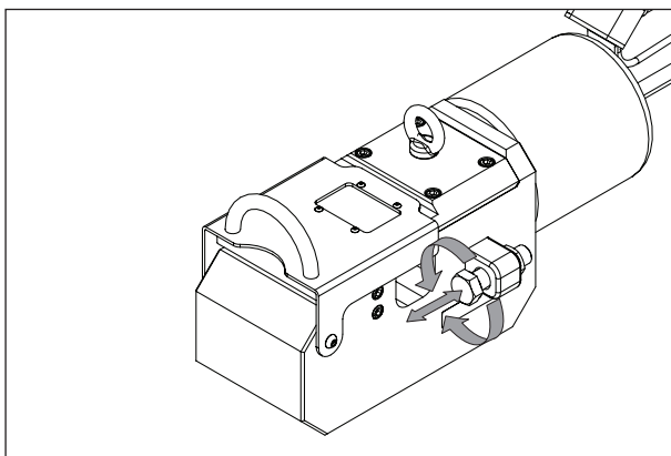
Figura 10, Ajustar el perno de soporte
