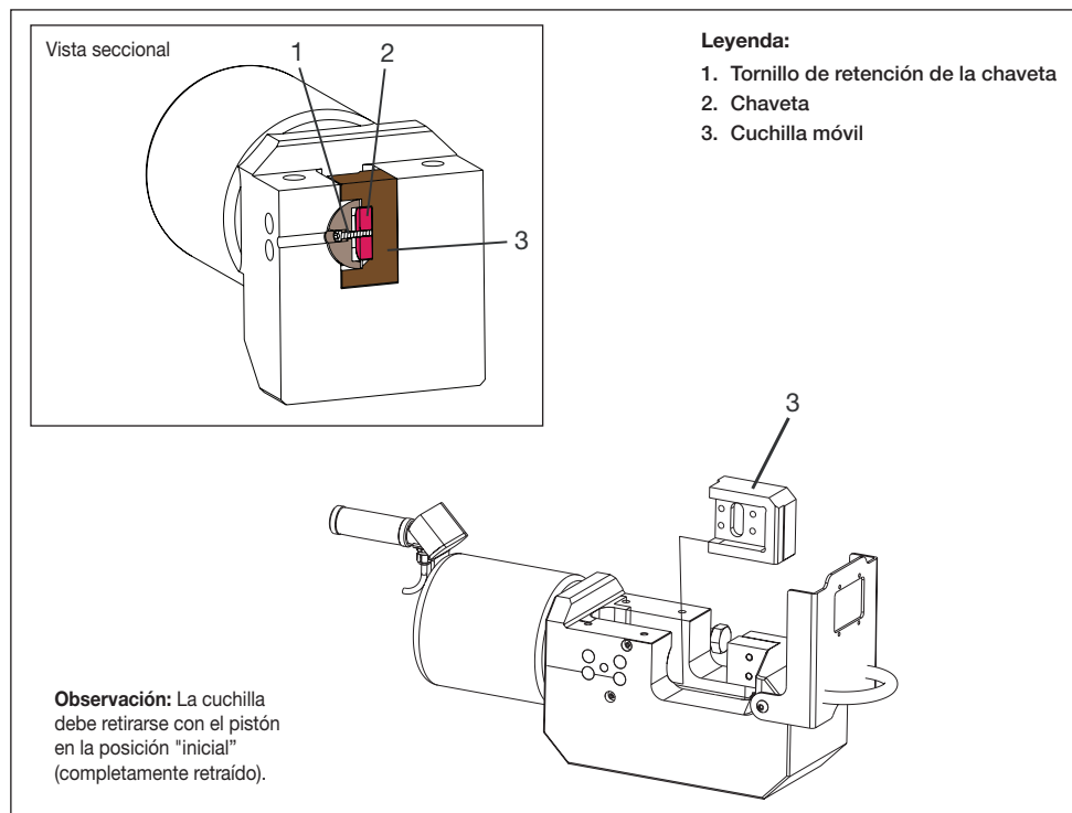
Figura 17, Sustitución de la cuchilla móvil (vista 2 de 2)
