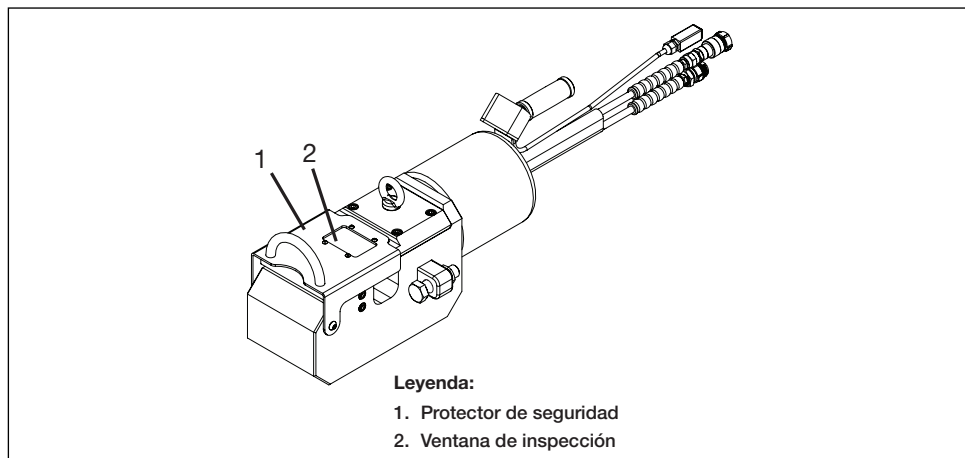
Figura 4, Protector de seguridad con ventana de inspección
