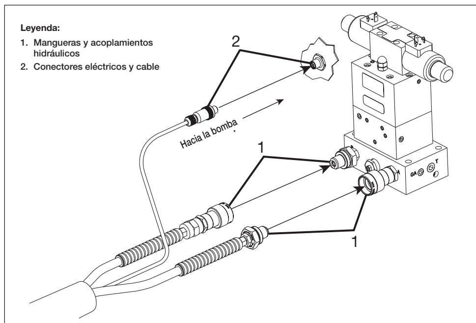
Figura 3, Conexiones hidráulicas y eléctricas en la bomba
