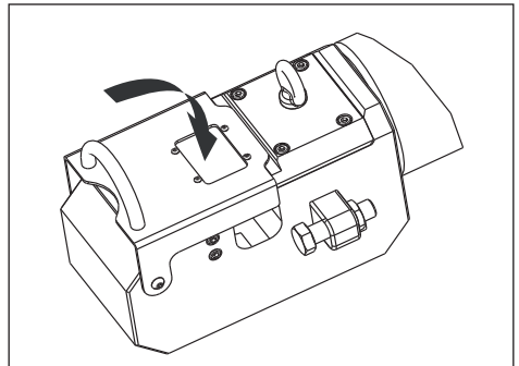
그림 6. 안전 가드 닫기
