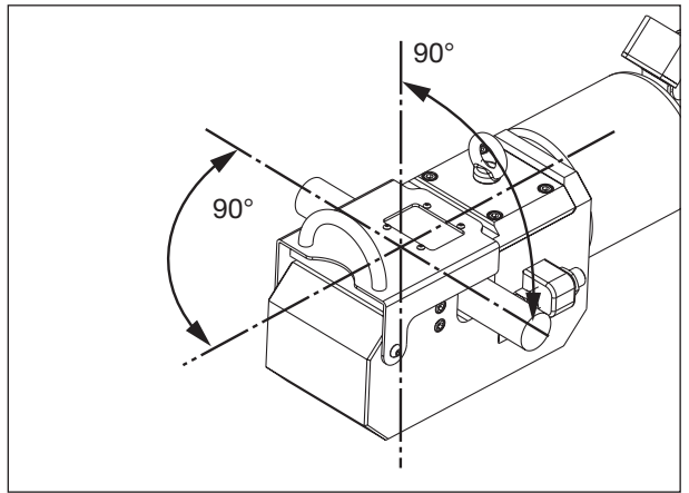
그림 9. 커팅 헤드의 재료 배치
