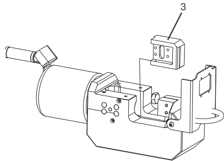
그림 17, 움직이는 날 교체 (보기 2 중 2)
