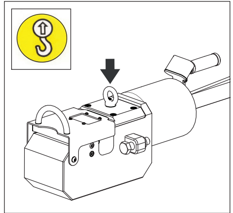
그림 7. 절단기 리프팅 위치
