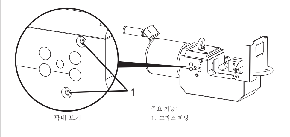
그림 14, 윤활
