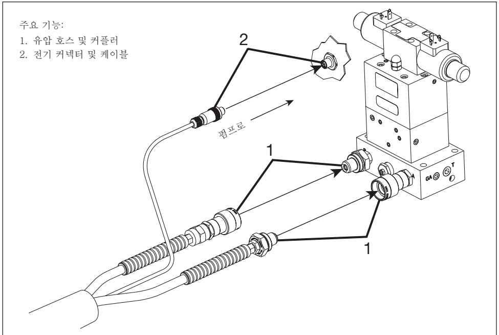
그림 3. 펌프의 유압 및 전기 연결
