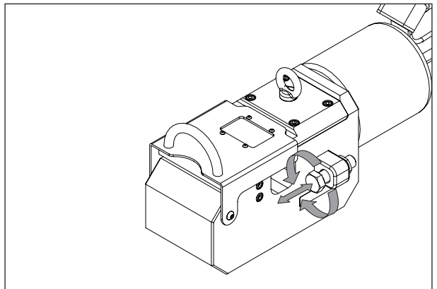
그림 10. 지지 볼트 조정
