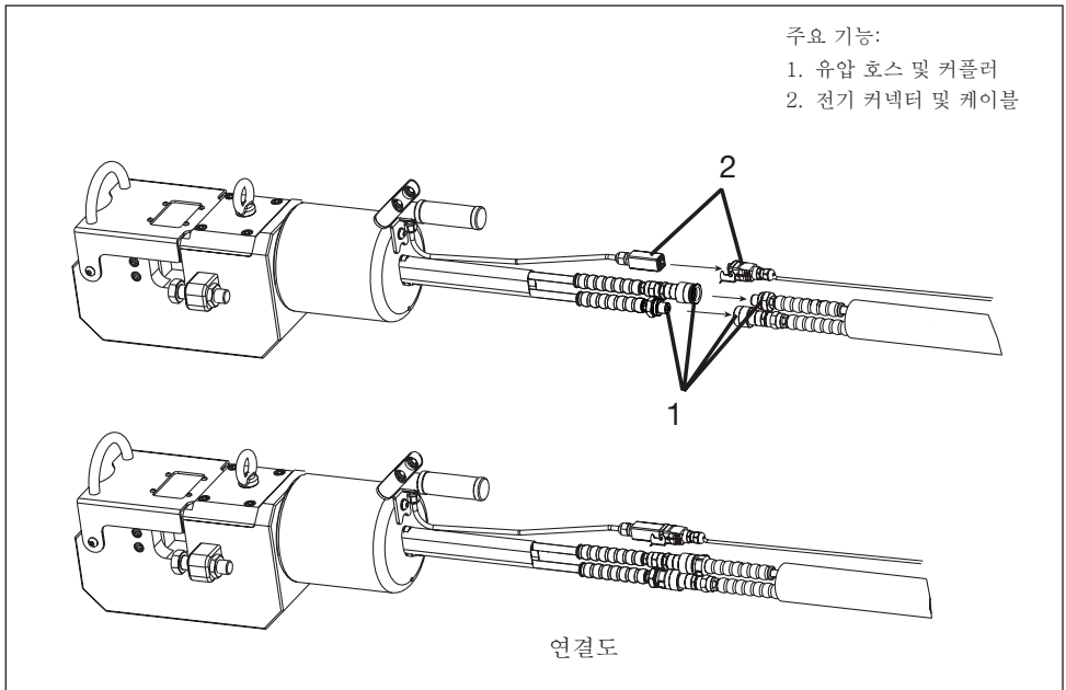
그림 2. 절단기의 유압 및 전기 연결(일반)
