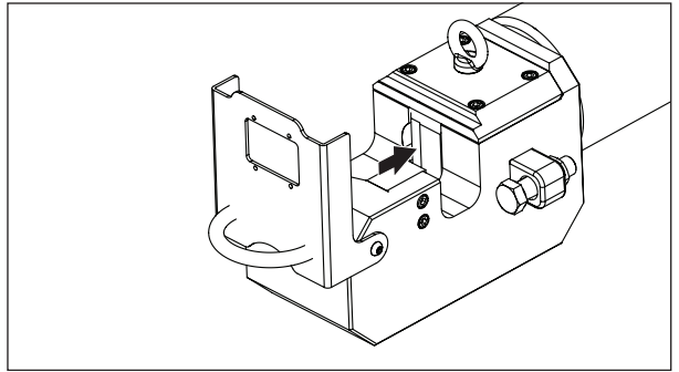
그림 8. 홈 위치의 피스톤과 날(완전히 후진한 상태)
