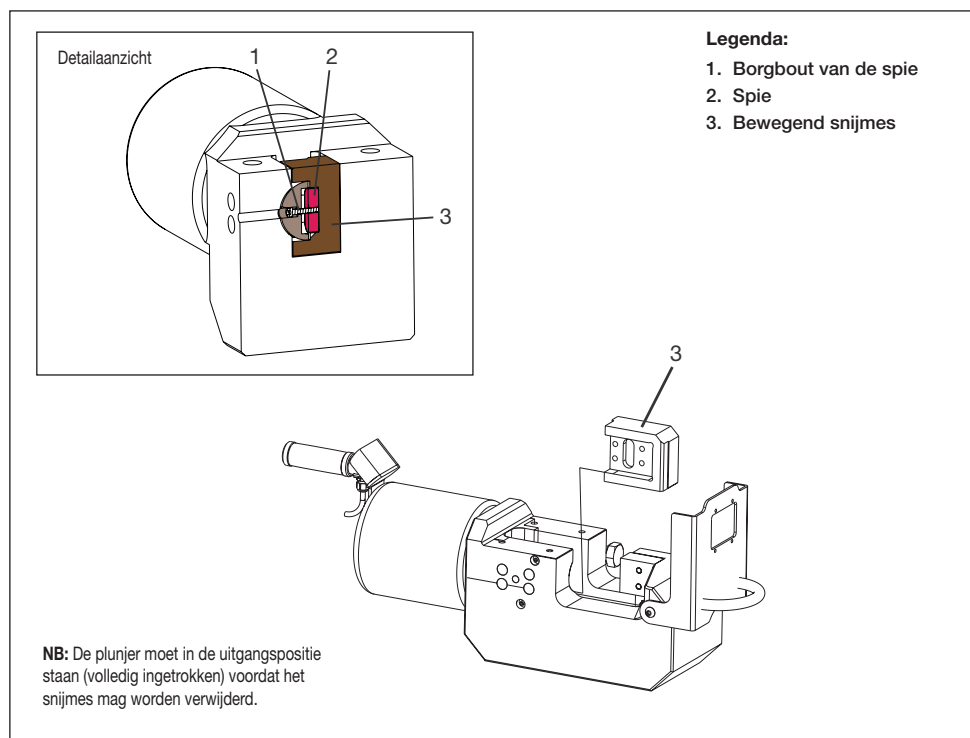
Figuur 17. Bewegend snijmes vervangen (weergave 2 van 2)
