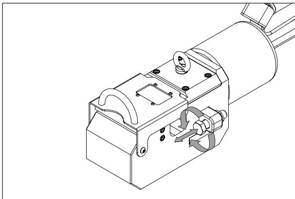
Figura 10, ajuste do parafuso de suporte
