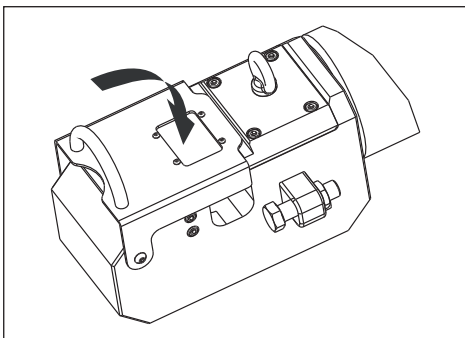
Figura 6, fechar a proteção de segurança
