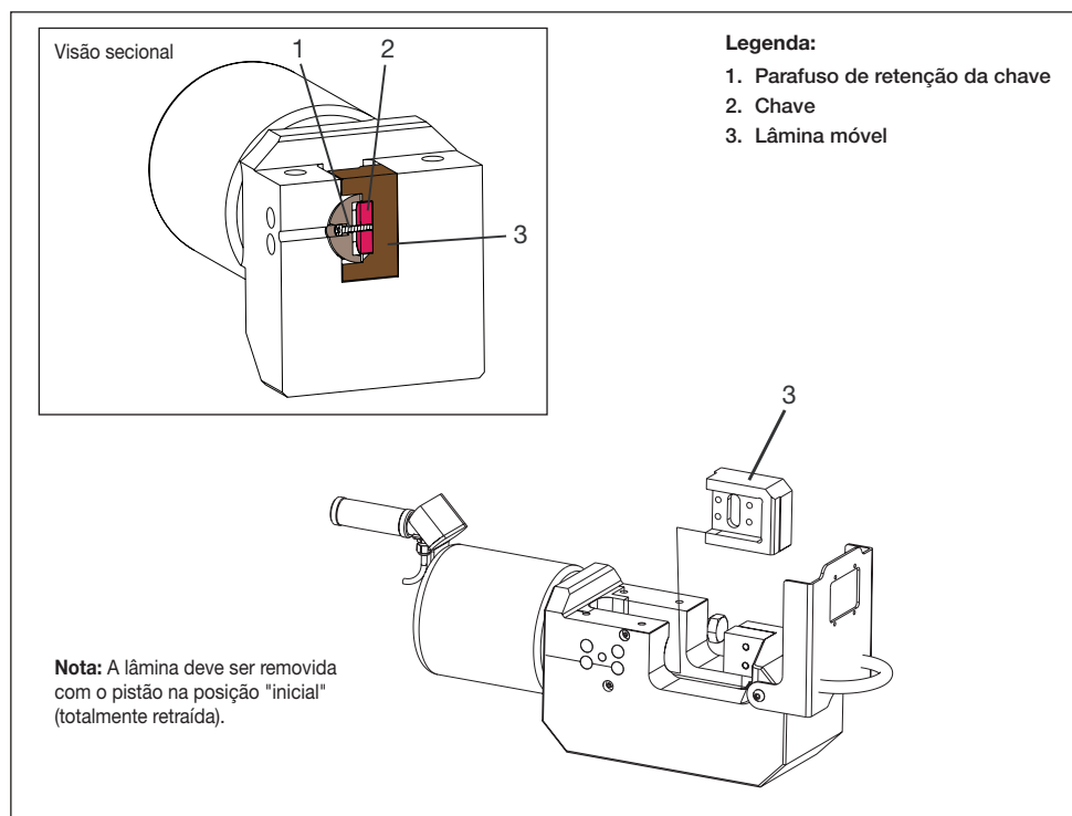
Figura 17, substituição da lâmina móvel (vista 2 de 2)
