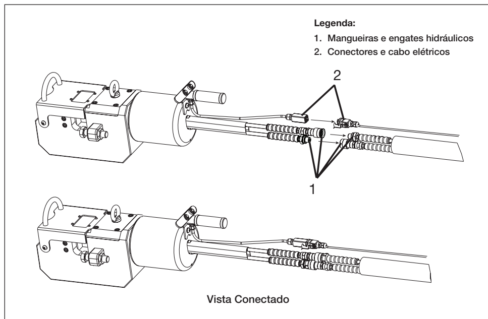
Figura 2, conexões hidráulicas e elétricas no cortador (típicas)
