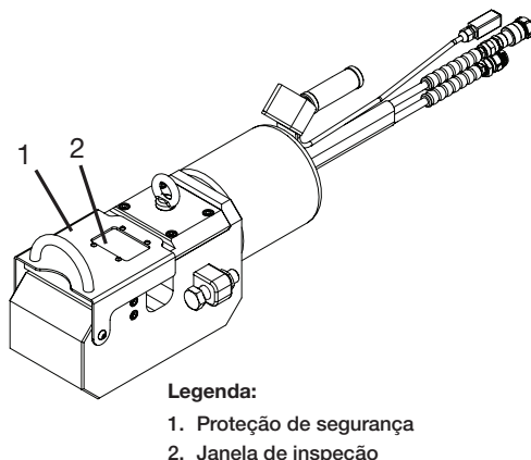
Figura 4, proteção de segurança com janela de inspeção
