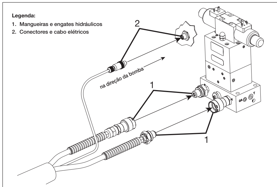
Figura 3, conexões hidráulicas e elétricas na bomba
