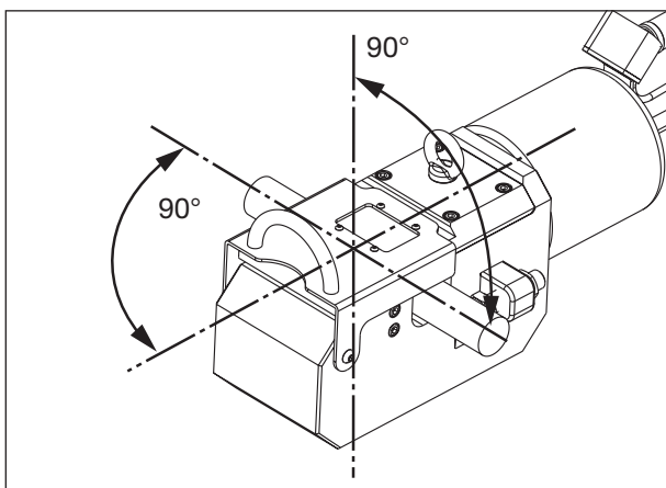
Figura 9, colocação do material no cabeçote de corte
