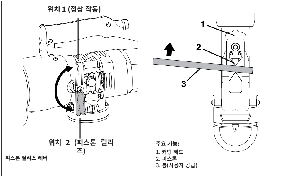
그림 17, 피스톤 수동 후진 절차
