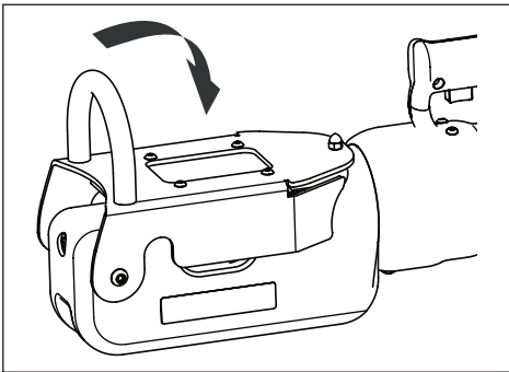
그림 4, 안전 가드 닫기
