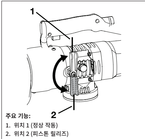
그림 8, 피스톤 릴리즈 나사
