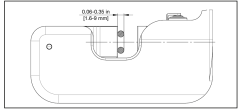
그림 12, 직경이 1.6~9mm인 링크 와이어의 위치
