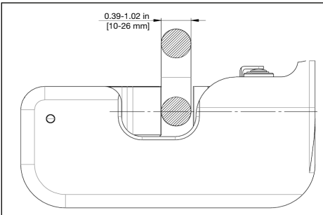
그림 11, 직경이 10~26mm인 링크 와이어의 위치
