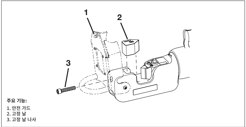
그림 15, 고정 날 교체
