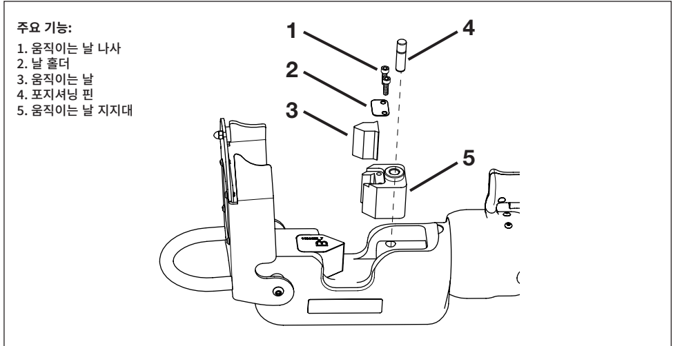
그림 16. 가동 날 교체
