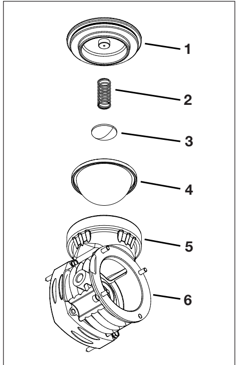
그림 14E, 다이어프램 커버 (1), 스프링 (2), 푸셔 디스크 (3), 다이어프램 (4), 다이어프램 입구 (5) 및 저장소 (6)
