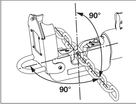
그림 10. 커팅 헤드 내 재료 위치
