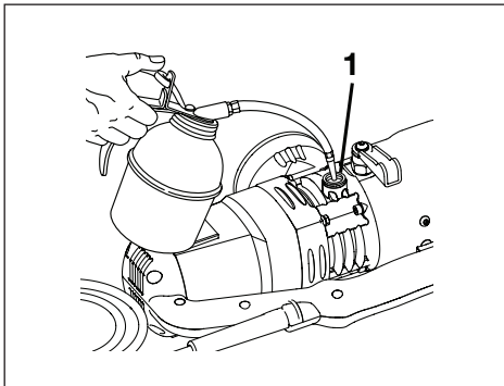
그림 14C, 저장소 보충 구멍에 오일 추가 (1)
