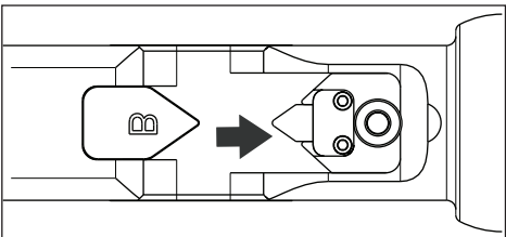
그림 7, 피스톤과 블레이드가 완전히 후진한 (“흠”) 위치
