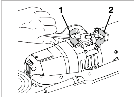
그림 14B, 오일 저장소 캡 - 풀림 (1) 및 조임 (2)
