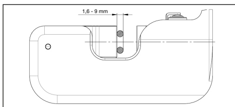
Figure 12, Emplacement pour un fil de maillon de 1,6 à 9 mm de diamètre
