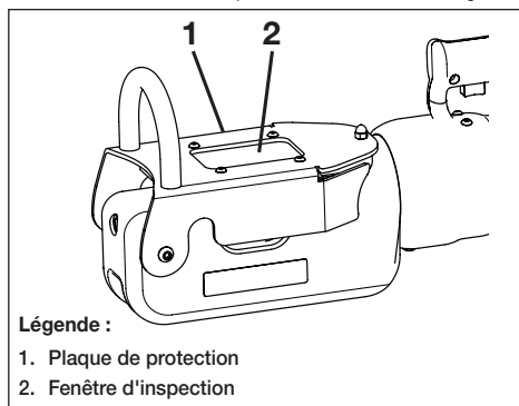
Figure 2, Plaque de protection avec fenêtre d'inspection
