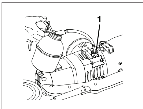
Figure 14C, Ajout d'huile via l'orifice de remplissage du réservoir (1)
