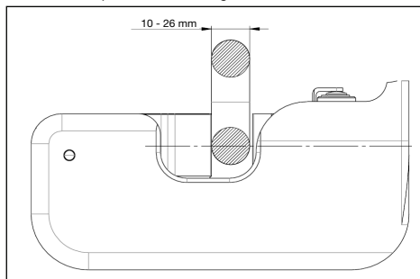
Figure 11, Emplacement pour un fil de maillon de 10 à 26 mm de diamètre
