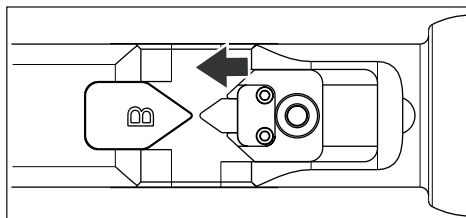
Figure 6, Piston et lame complètement sortis
