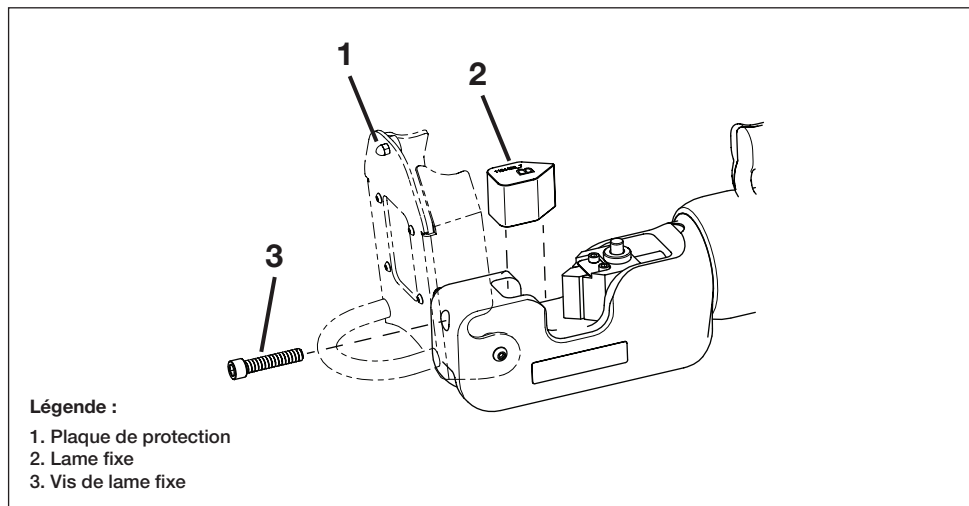
Figure 15, Remplacement de la lame fixe
