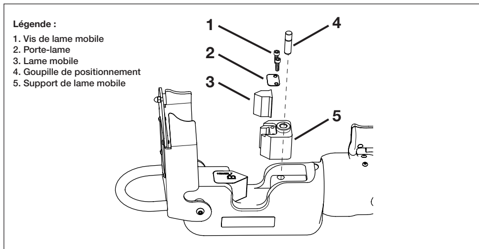
Figure 16, Remplacement de la lame mobile
