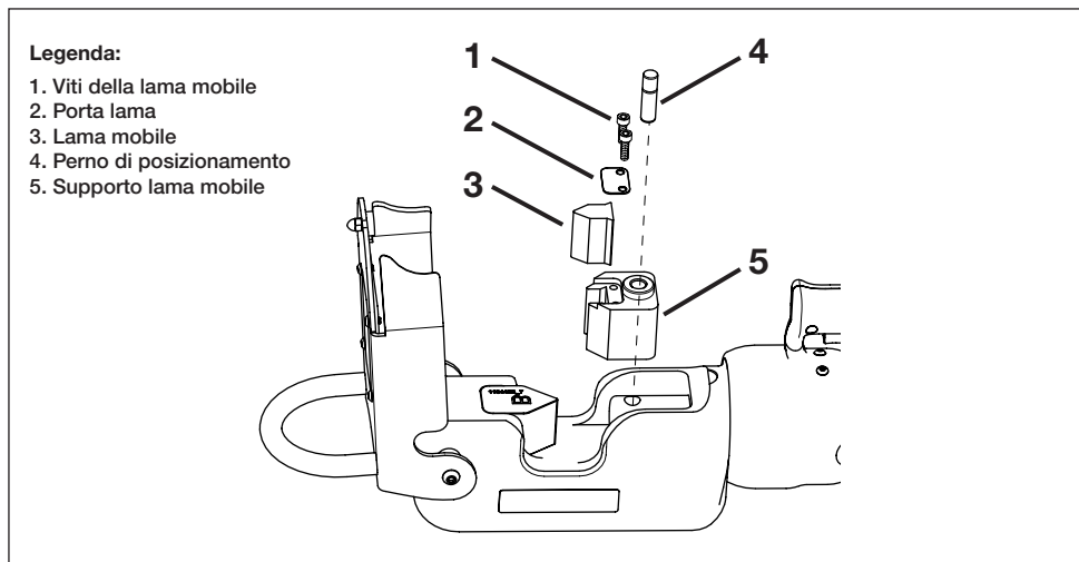
Figura 16, Sostituzione della lama mobile
