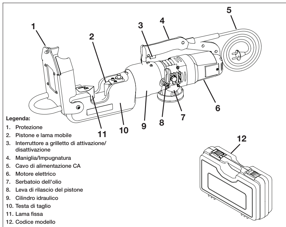
Figura 1, Caratteristiche e componenti
