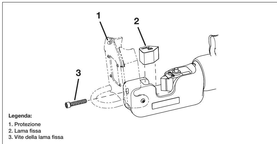
Figura 15, Sostituzione della lama fissa
