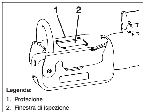
Figura 2, Protezione con finestra di ispezione
