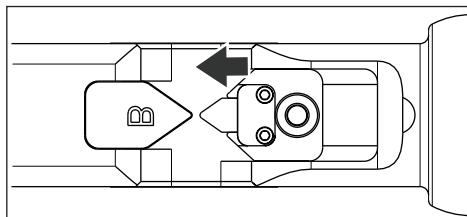
Figure 6, Pistone e lama completamente estesi
