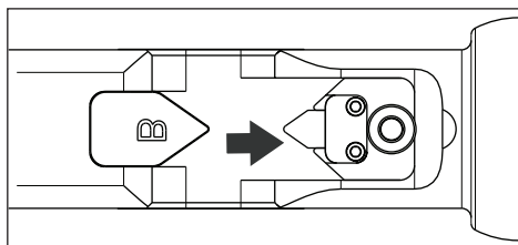
Figure 7, Pistone e lama completamente retratti (posizione "Home")
