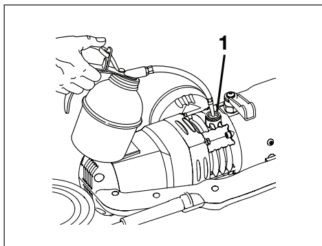
Figura 14C, Aggiunta di olio nel foro di riempimento del serbatoio (1)
