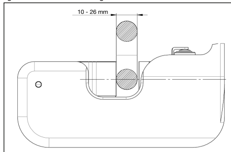
Figura 11, Posizione dell'anello con diametro da 10-26 mm
