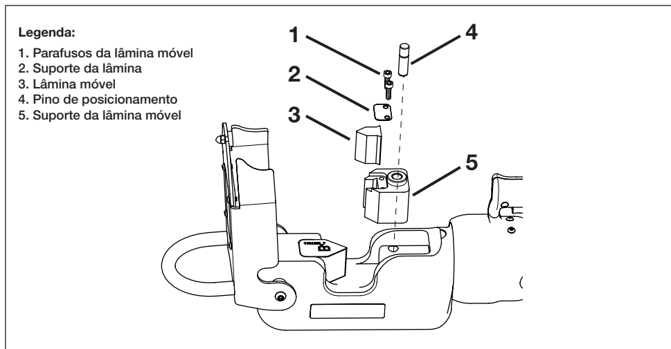
Figura 16, troca da lâmina móvel
