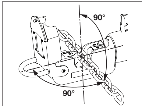
Figura 10, posicionamento do material no cabeçote de corte
