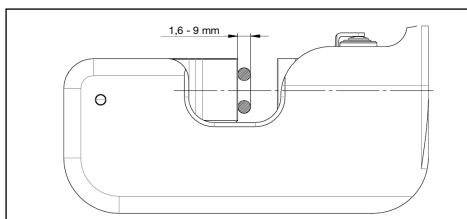
Figura 11, posição para correntes com diâmetro de 1,6-9 mm
