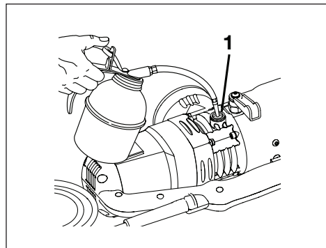
Figura 14C, adição de óleo ao orifício de preenchimento do reservatório (1)
