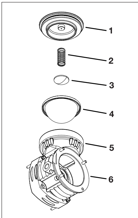
Figura 14E, tampa do diafragma (1), mola (2), disco impulsor (3), diafragma (4), abertura do diafragma (5) e reservatório (6)
