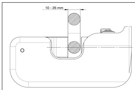
Figura 11, posição para correntes com diâmetro de 10-26 mm
