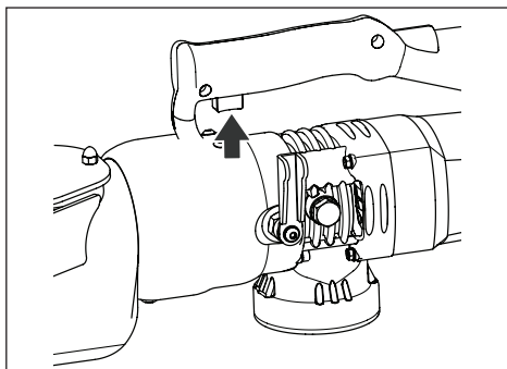
Figura 5, interruptor on/off (ligar/desligar) do gatilho
