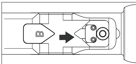
Figure 7, pistão e lâmina totalmente retraídos posição ("Inicial")
