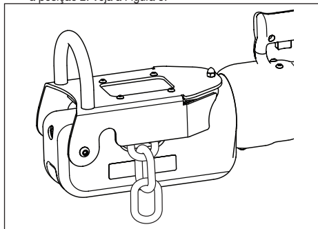
Figura 13, material sendo cortado (típico)
