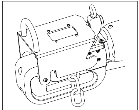
Abbildung 14, Zu durchtrennende Kette (typisch)
