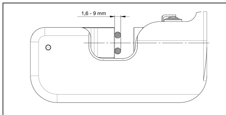
Abbildung 13, Position für Draht mit einem Durchmesser von 1,6-9 mm
