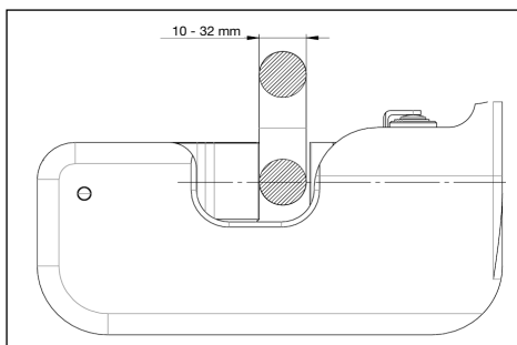
Abbildung 12, Position für Draht mit einem Durchmesser von 10-32 mm
