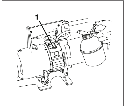
Abbildung 15D, Öl in Tanköffnung einfüllen (1)
