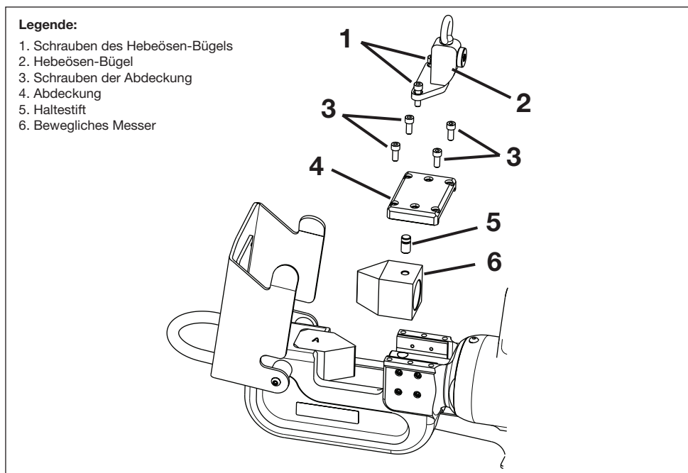
Abbildung 18, Austausch des beweglichen Messers
