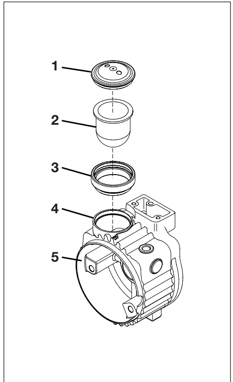
Abbildung 15E, Membranabdeckung (1), Membran (2), Verlängerung (3), Membranöffnung (4) und Öltank (5)
