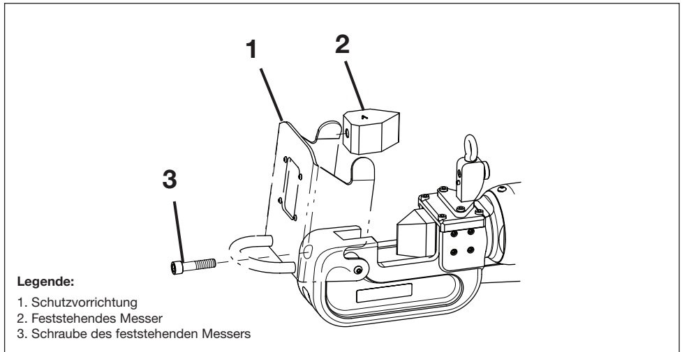
Abbildung 17, Austausch des feststehenden Messers
