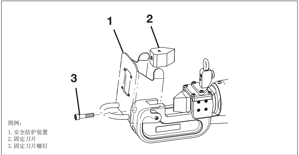
图 17，固定刀片更换
