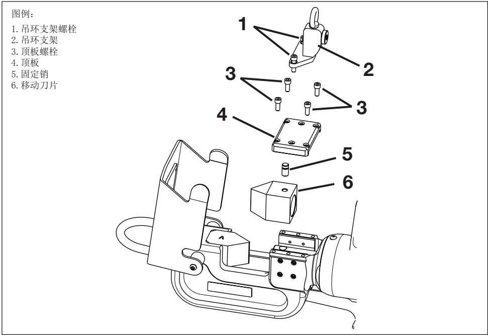
图 18，移动刀片更换
