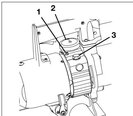
图 15A, 通气螺钉 (1), 隔膜盖 (2) 和油箱盖 (3)
