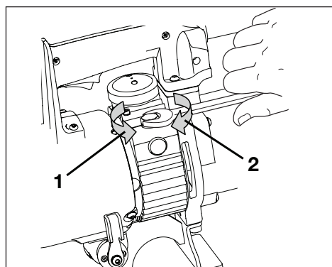
图 15C, 油箱盖 - 旋松 (1) 和旋紧 (2)
