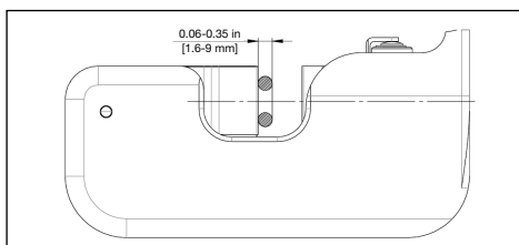
图 13, 1.6-9 mm 直径铁丝的位置
