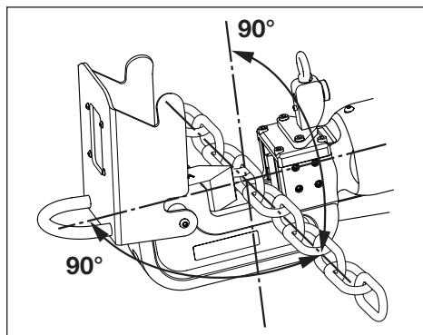
图 11, 在切割头中放置待切割链条
