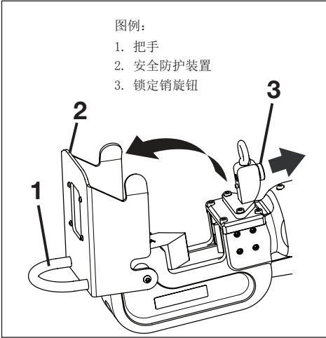
图 3，打开安全防护装置
