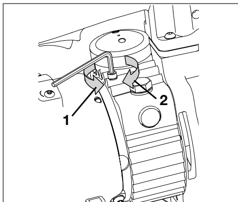
图 15B, 通气螺栓 - 旋松 (1) 和旋紧 (2)
