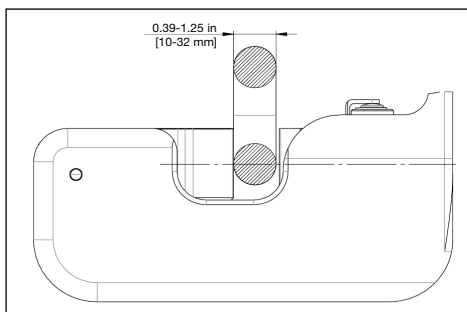
图 12, 10-32 mm 直径铁丝的位置
