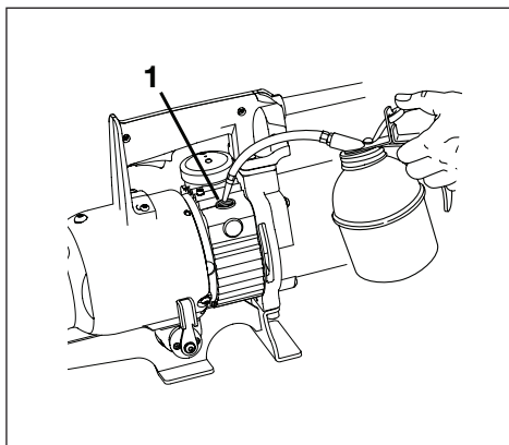
图 15D, 注油至油箱注油口 (1)
