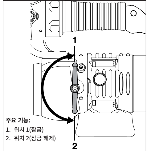
그림 2. 수동 릴리즈 나사
