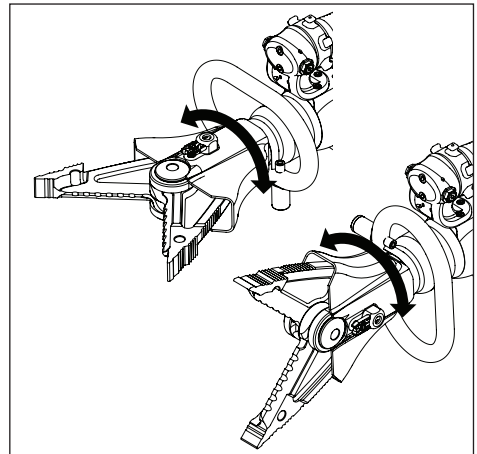
그림 3. 회전 커팅 헤드
