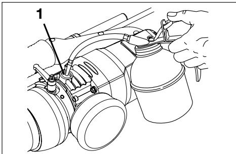
그림 9C. 저장소 보충 구멍에 오일 추가(1)
