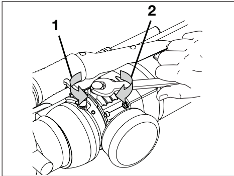
그림 9B. 오일 저장소 캡 - 풀림 (1) 및 조임 (2)
