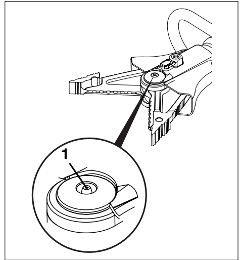
그림 10. 그리스 피팅, 중앙 핀(1)
