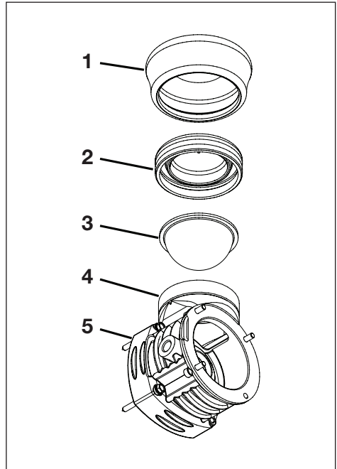
그림 9E. 고압 지지대(1), 다이어프램 하우징 커버(2), 다이어프램(3), 다이어프램 입구(4) 저장소(5)
