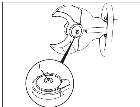
図8: グリースフィッティング、中央ピン (1)
