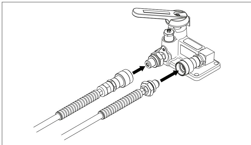
図3:ポンプ部の油圧接続部
