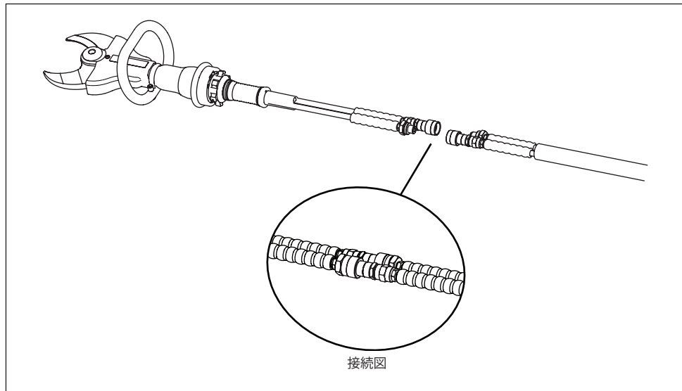
図2:カッター部の油圧接続部
