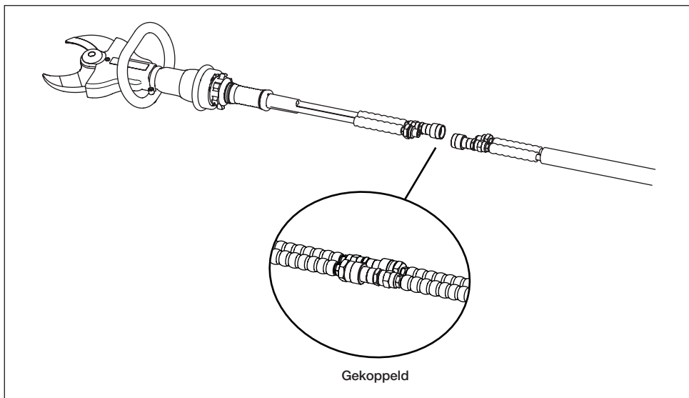
Figuur 2. Hydraulische aansluitingen op knipper
