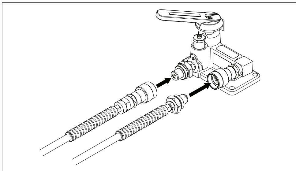
Figuur 3. Hydraulische aansluitingen op pomp
