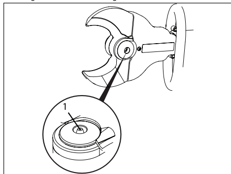
Figuur 8. Smeren van centrale pin (1)
