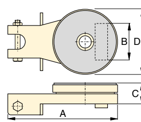
ES10, ES15, ES30 Prato giratório
