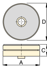
ES1, Prato giratório
