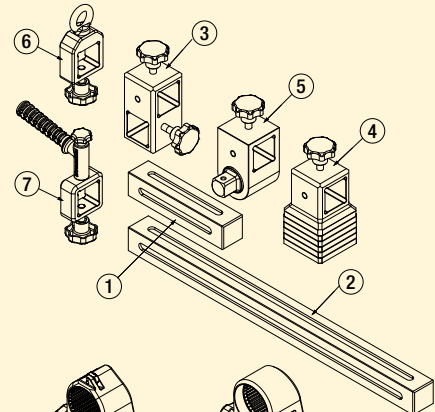
TWRAKRSL * RSL 시리즈용 렌치 어댑터 어셈블리
