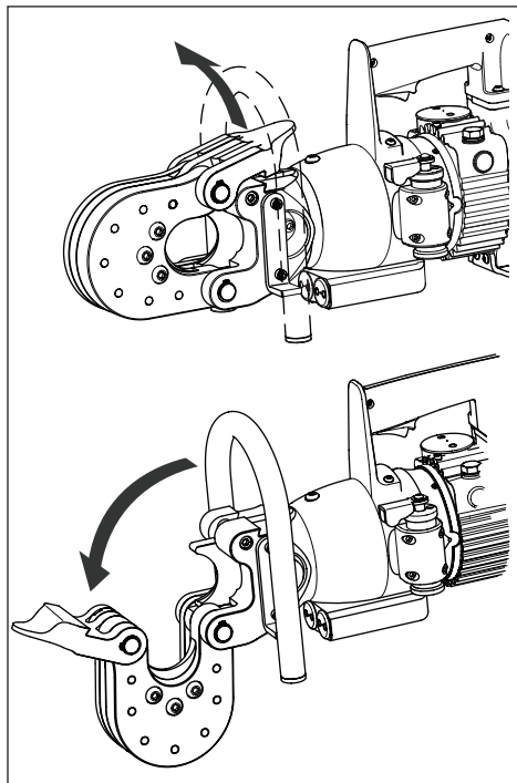
Figura 2, abrir o cabeçote de corte
