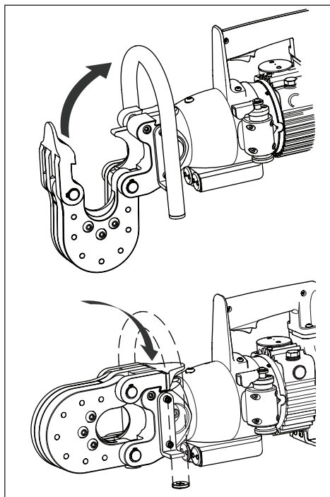
Figura 3, fechar o cabeçote de corte
