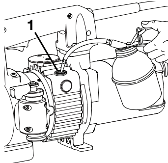
Figura 10D, adição de óleo ao orifício de preenchimento do reservatório (1)
