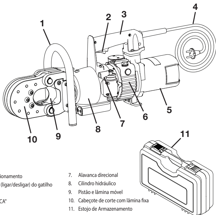
Figura 1, características e componentes
