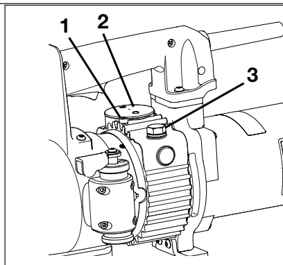
Figura 10A, parafuso de ventilação (1), tampa do diafragma (2) e tampa do reservatório de óleo (3)
