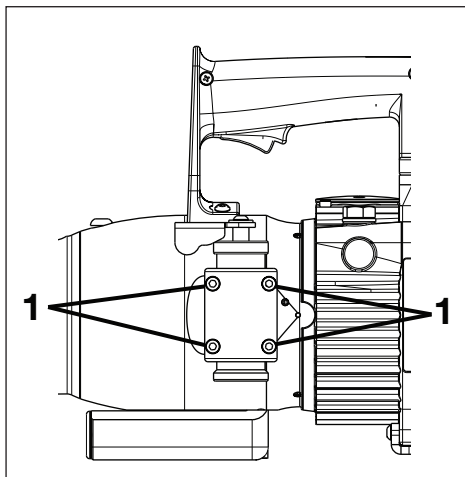
Figura 11, parafusos da válvula de controle direcional (1)
