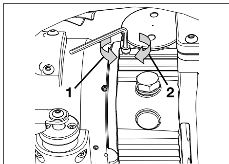
Figura 10B, parafuso de ventilação - solto (1) e apertado (2)
