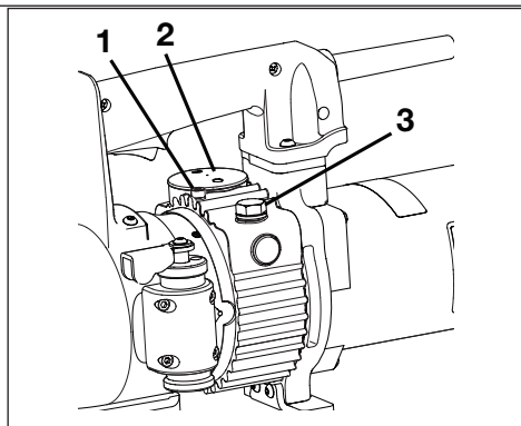
图 10A, 通气螺钉 (1), 隔膜盖 (2) 和油箱盖 (3)
