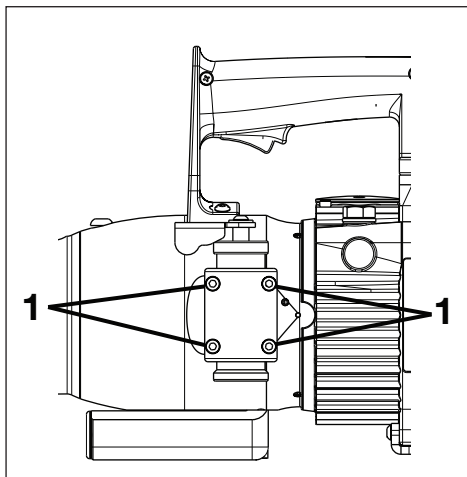
图 11，方向控制阀螺钉（1）
