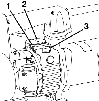
Abbildung 10A, Entlüftungsschraube (1), Membranabdeckung (2) und Tankdeckel (3)
