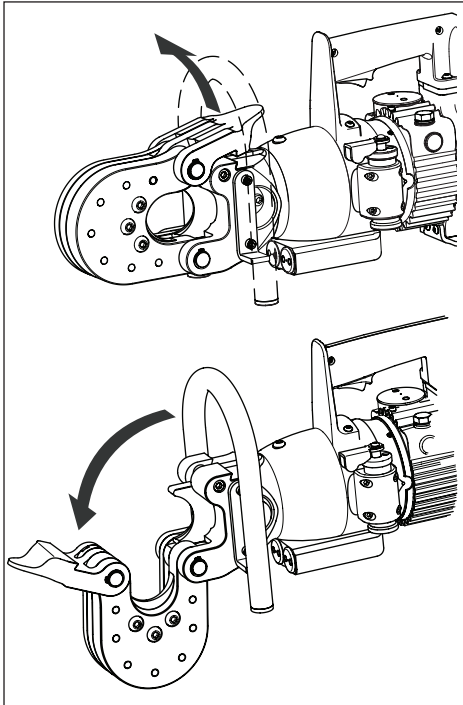
Abbildung 2, Schneidkopf öffnen
