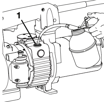
Abbildung 10D, Öl in Tanköffnung (1)
