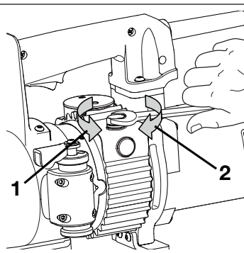
Abbildung 10C, Tankdeckel des Öltanks - lösen (1) und anziehen (2)
