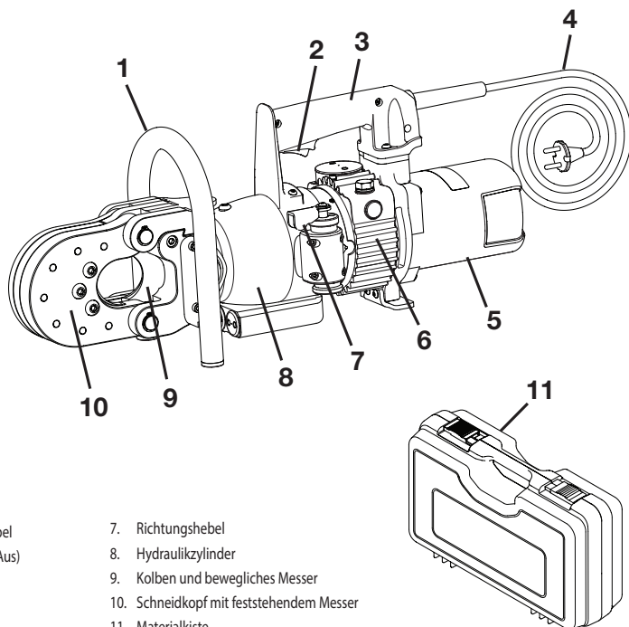
Abbildung 1, Funktionen und Komponenten
