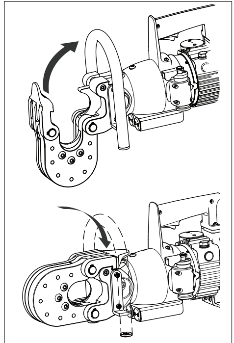
Abbildung 3, Schneidkopf schließen
