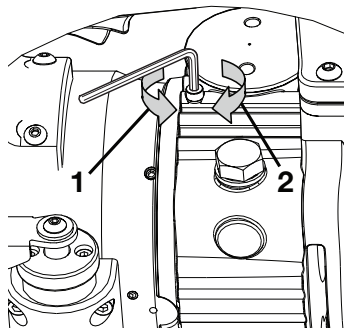
Abbildung 10B, Entlüftungsschraube - lösen (1) und anziehen (2)
