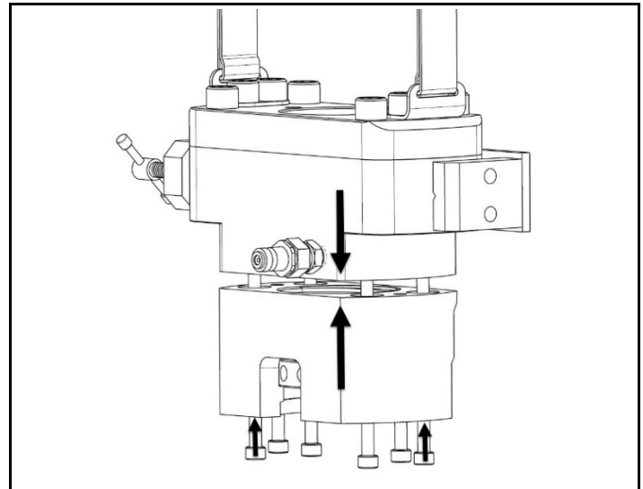
Kuva 4.15 Aseta pääkokoonpano siltakokoonpanon päälle, kiinnitä kuusiokoloruuveilla
