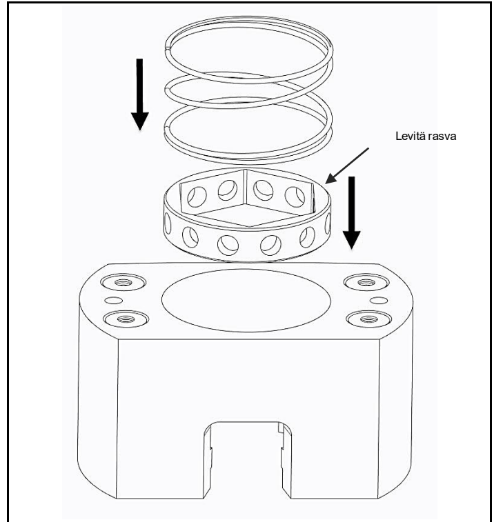
Kuva 4.13 Rasvaa ja aseta muhvi paikoilleen, aseta sen jälkeen puristusjousi
