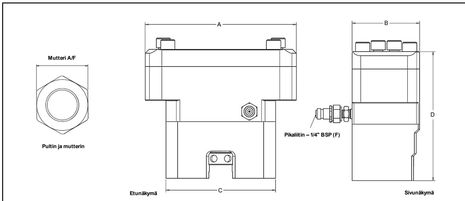
Taulukko 1, tekniset tiedot, FTE-sarjan elliptinen perustuskiristin
