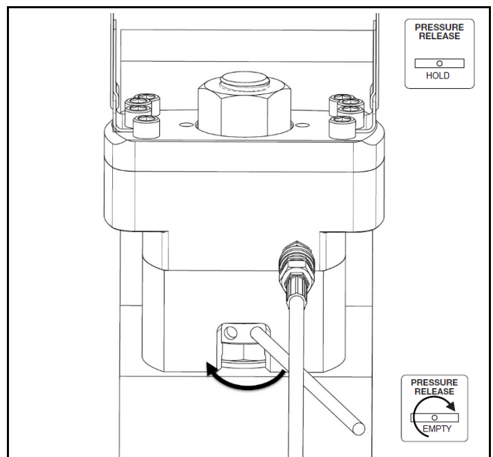
Kuva 2.6 Pidä paine mutterin kiristystä varten
