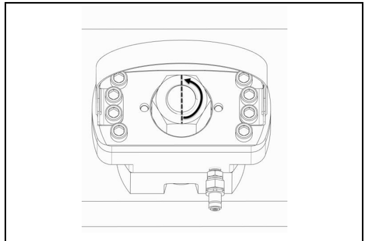
Kuva 3.1 Kiristä reaktiomutteria ja käännä takaisin ½ kierrosta
