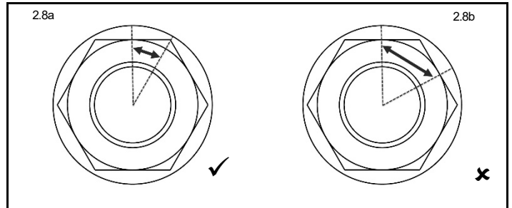
Kuva 2.8a Pultin kiristys valmis
