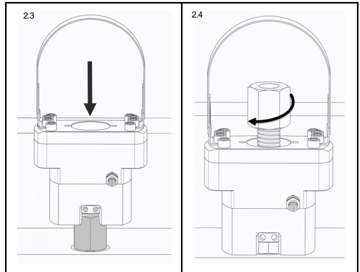
Kuva 2.3 Aseta kiristin käyttökohteeseen
