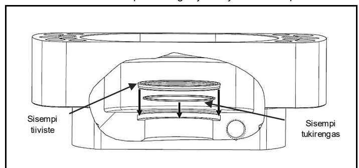
Kuva 4.8 Aseta sisempi tiiviste ja sen jälkeen sisempi tukirengas
