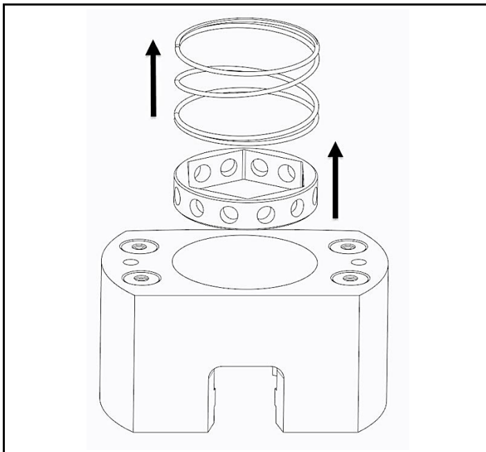
Kuva 4.12 Poista puristusjousi ja muhvi
