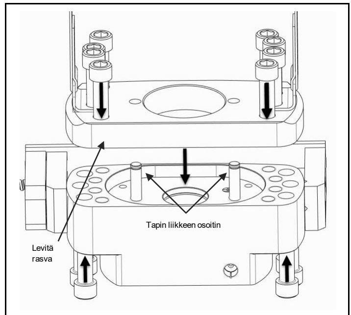
Kuva 4.11 Levitä rasva, aseta tapin liikkeen osoitin, kiinnitä rajoituslevy runkoon
