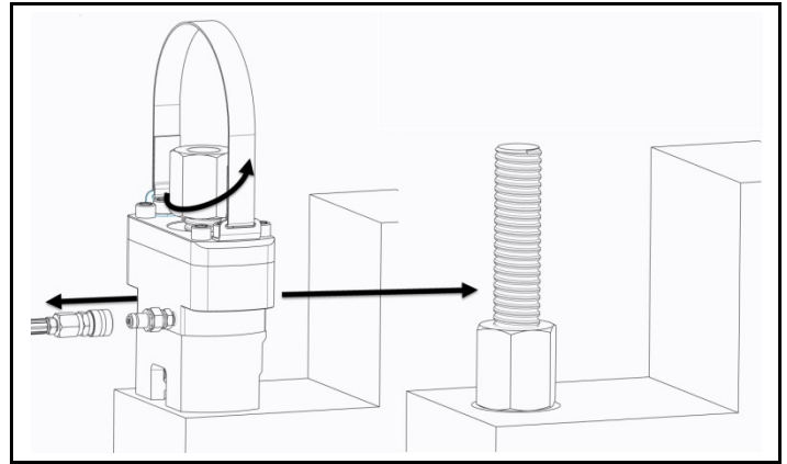
Kuva 2.7 Irrota letku, poista kiristin ja aseta se uudelleen
