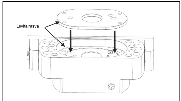
Kuva 4.10 Levitä rasva, aseta varoventtiilikokoontalo, kiinnitä jousipalautuslevyn alle
