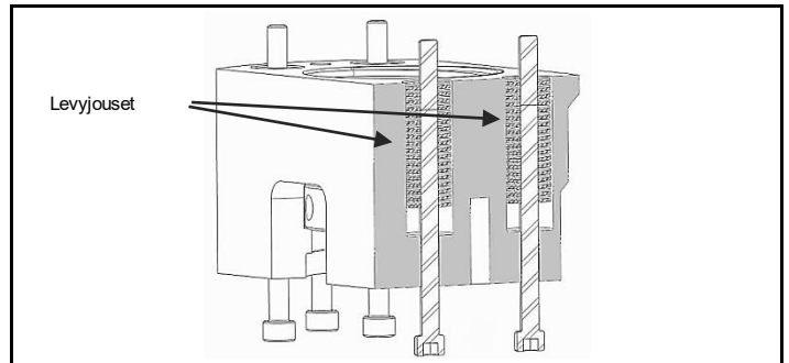
Kuva 4.2 Levyjousien sijainti sillassa
