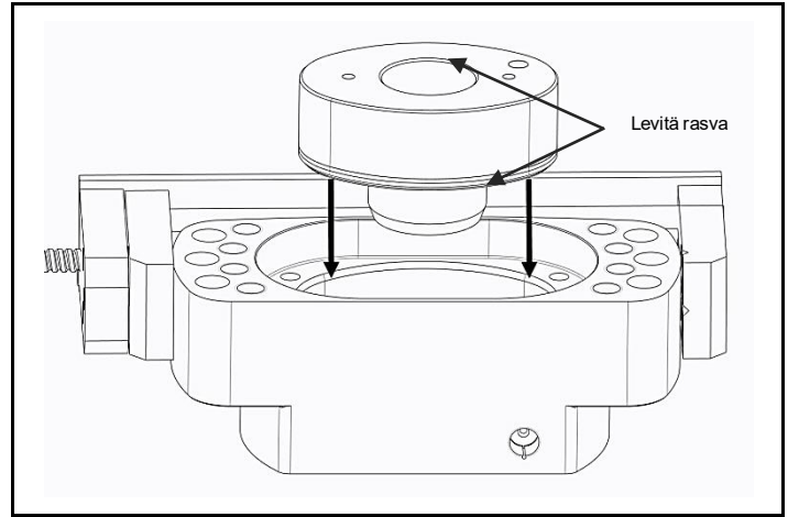
Kuva 4.9 Levitä rasva ja asenna mäntä
