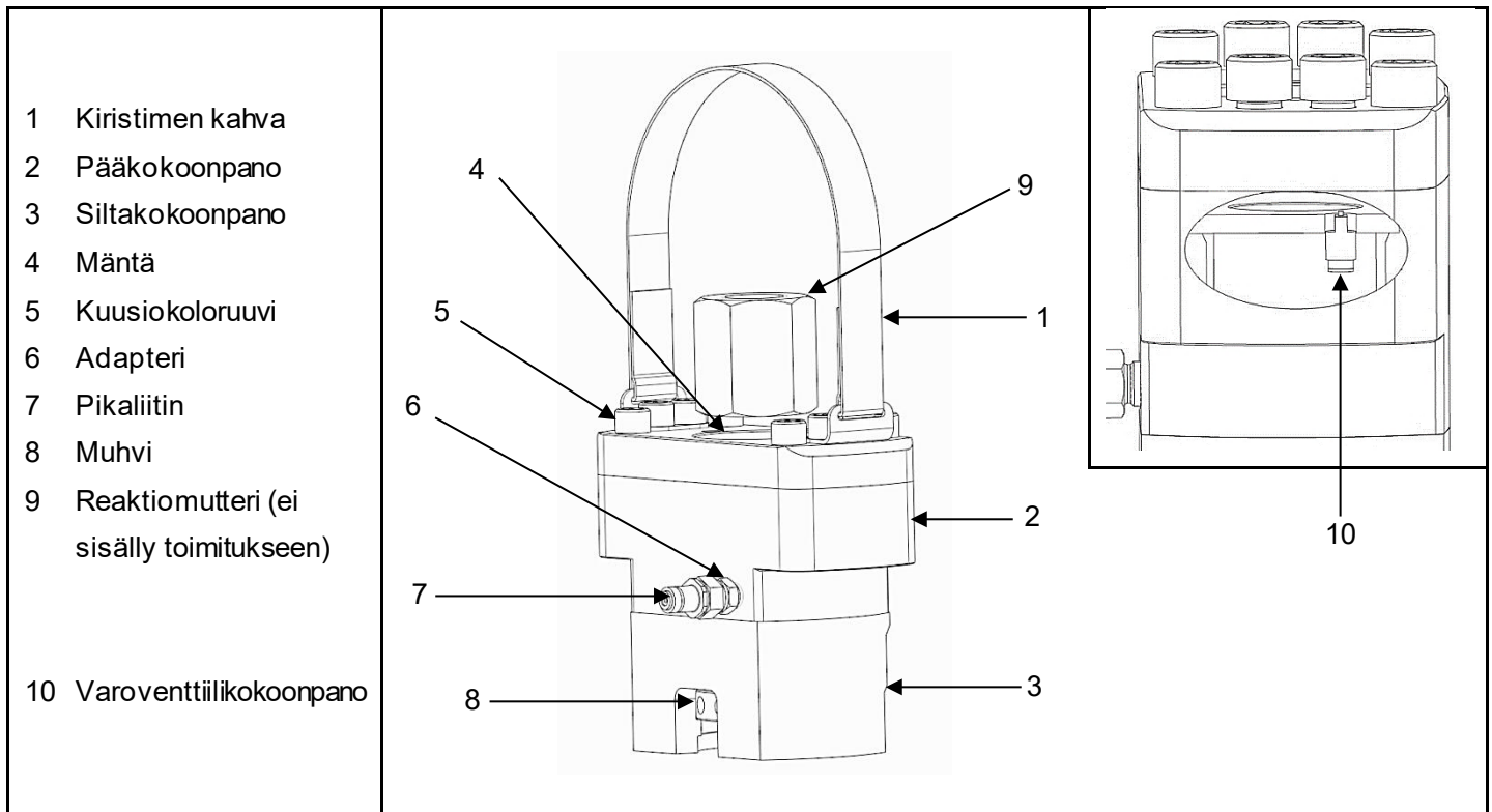
Kuva 1.1 FTE-sarjan elliptisten perustuskiristinten pääominaisuudet ja komponentit
