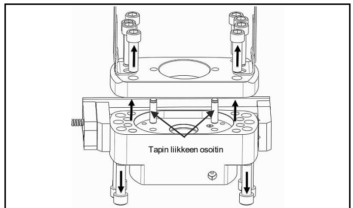
Kuva 4.3 Poista rajoituslevy ja eristä tapin liikkeen osoitin
