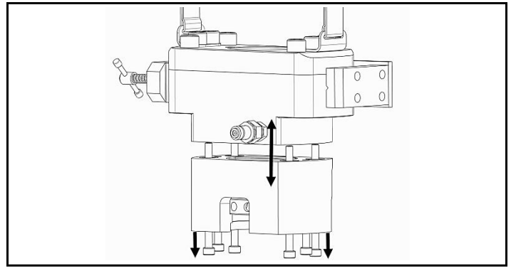
Kuva 4.1 Irrota pääkokoonpano ja siltakokoonpano
