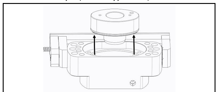
Kuva 4.5 Poista mäntä tiivisteiden puhdistusta ja vaihtoa varten
