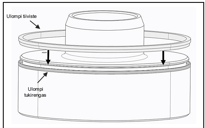
Kuva 4.7 Aseta ulompi tukirengas ja sen jälkeen ulompi tiiviste
