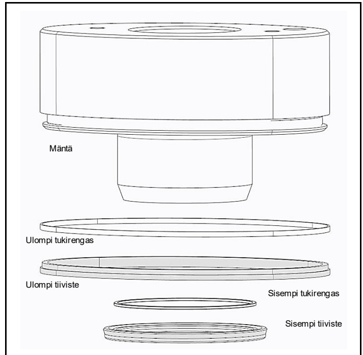
Kuva 4.6 Mäntä, ulompi tukirengas/tiiviste, sisempi tukirengas/tiiviste
