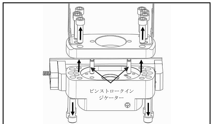
図 4.3 制限プレートの取り外し、およびピンストロークインジケータの分離
