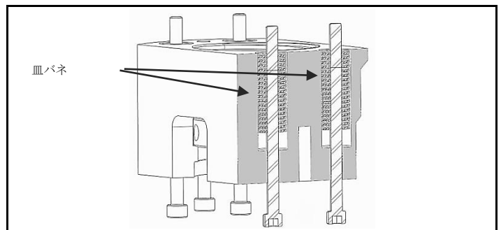
図 4.2 ブリッジ内の皿バネの位置
