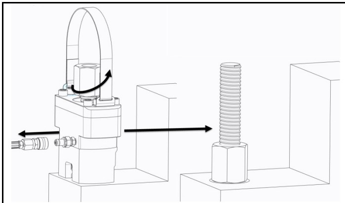
図 2.7 ホースの取り外し、テンショナーの取り外しおよび再配置
