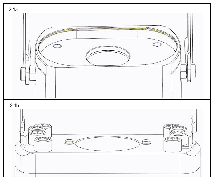
図 2.1a 最大ストロークインジケータ溝
