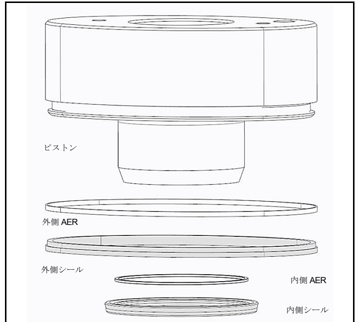
図 4.6 ピストン、外側 AER/シール、内側 AER/シール
