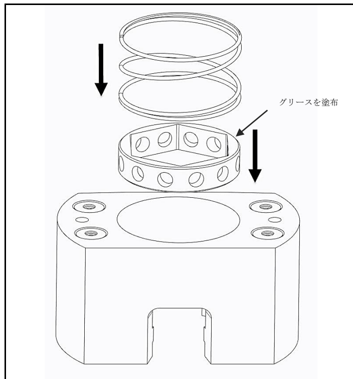
図 4.13 ソケットへのグリース塗布、ソケットの挿入後、圧縮スプリングの挿入
