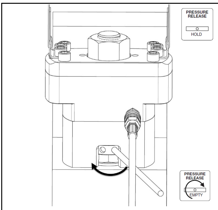
図 2.6 圧力を維持してナットを締め付け
