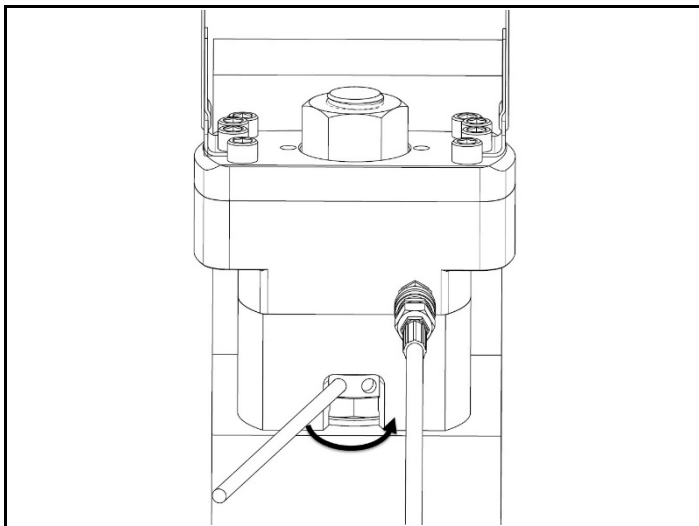
図 3.2 リアクションナットを反時計回りに回す
