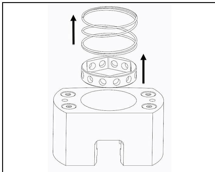
図 4.12 圧縮スプリングとソケットの取り外し
