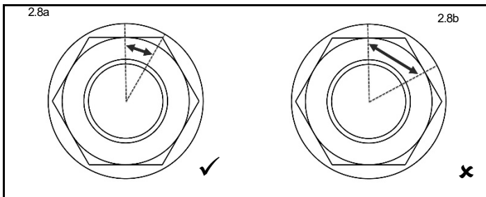
図 2.8a ボルトテンショニング完了
