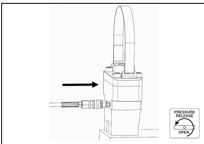
図 2.5 ホースの接続
