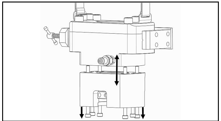
図 4.1 ヘッドアセンブリとブリッジアセンブリの分離
