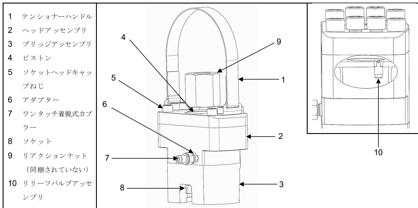
図 1.1 FTE シリーズファウンデーション楕円テンショナーの特長と構成部品
