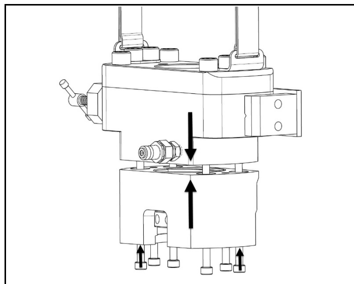
図 4.15 ヘッドアセンブリのブリッジアセンブリへの配置、ソケットヘッドねじでの固定
