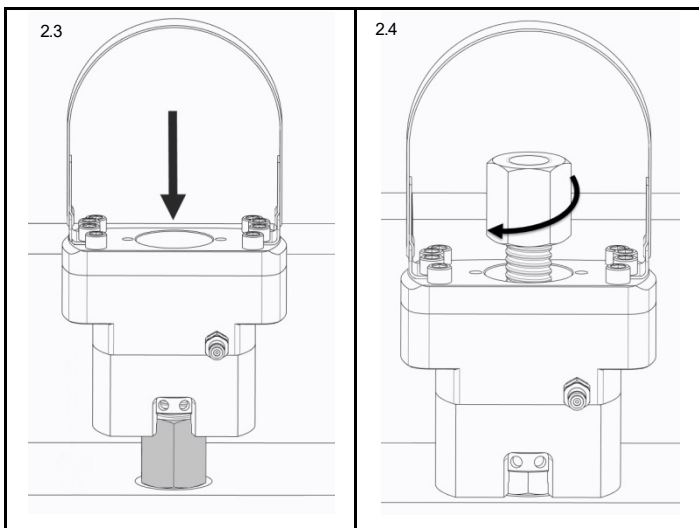
図 2.3 適用対象へのテンショナーの配置
