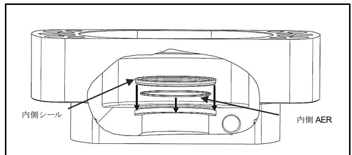
図 4.8 内側シールの挿入後、内側 AER を挿入
