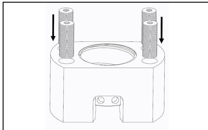
図 4.14 皿バネの挿入 (取り外した場合)
