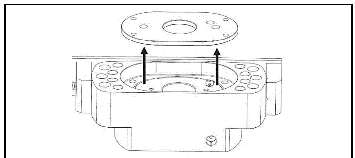
図 4.4 スプリングリテンションプレートの取り外し、およびピンストロークインジケータの分離
