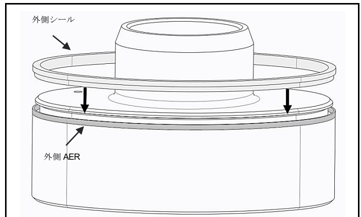
図 4.7 外側 AER の挿入後、外側シールを挿入
