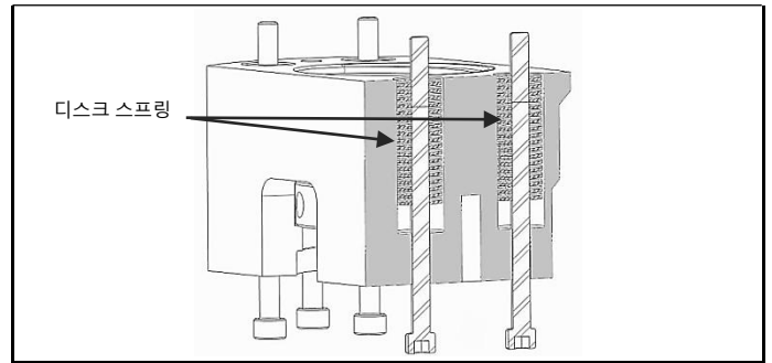
그림 4.2 브리지 내의 디스크 스프링 위치
