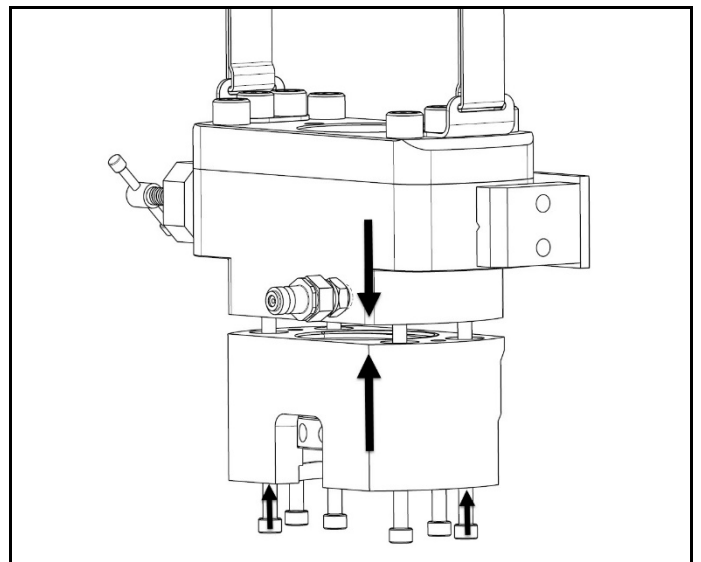
그림 4.15 헤드 어셈블리를 브리지 어셈블리에 배치, 소켓 헤드 나사로 고정
