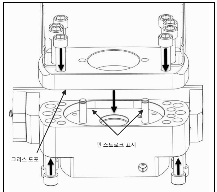
그림 4.11 그리스 도포, 핀 스트로크 표시 삽입, 본체에 제한판 고정
