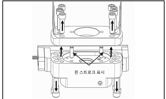
그림 4.3 제한판 제거 및 핀 스트로크 표시 분리
