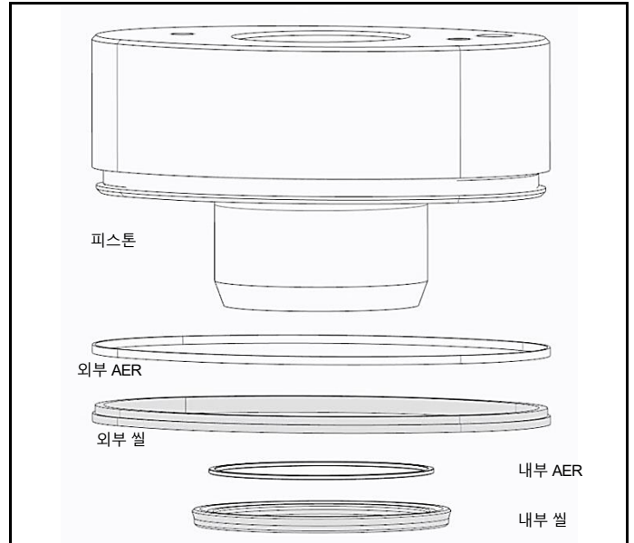
그림 4.6 피스톤, 외부 AER/실, 내부 AER/실
