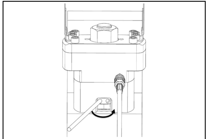
그림 3.2 리액션 너트를 시계 반대 방향으로 돌리기
