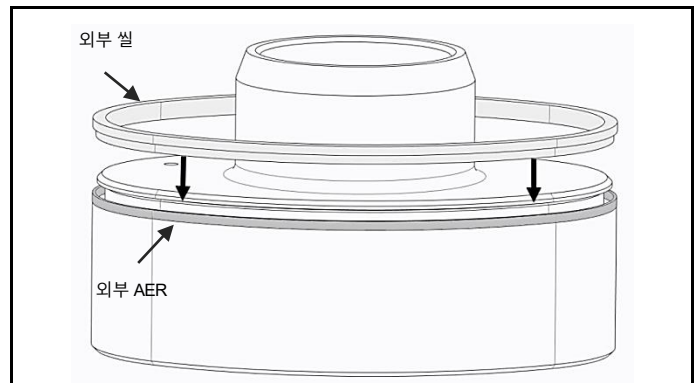
그림 4.7 외부 AER 삽입 후 외부 실 삽입
