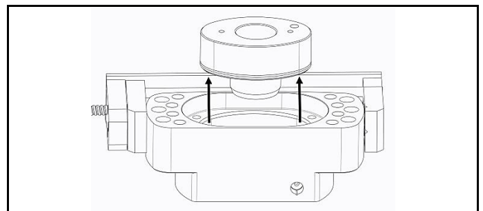
그림 4.5 피스톤을 제거하여 실을 청소하고 교체
