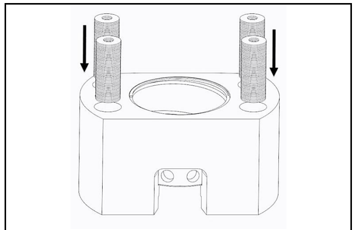
그림 4.14 디스크 스프링 삽입(제거된 경우)
