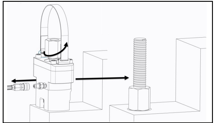
그림 2.7 호스 분리, 텐서너 제거 및 재배치
