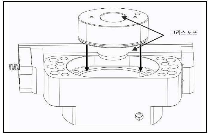
그림 4.9 그리스 도포 및 피스톤 설치
