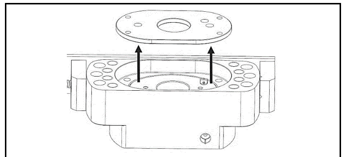
그림 4.4 스프링 고정판 제거 및 핀 스트로크 표시 분리
