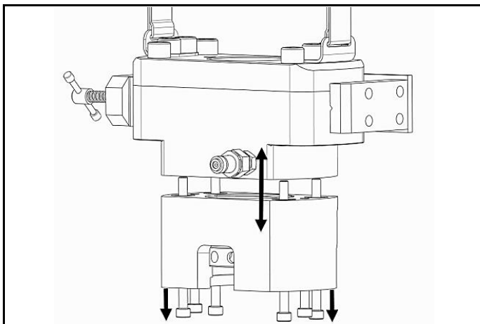
그림 4.1 헤드 어셈블리 및 브리지 어셈블리 분리
