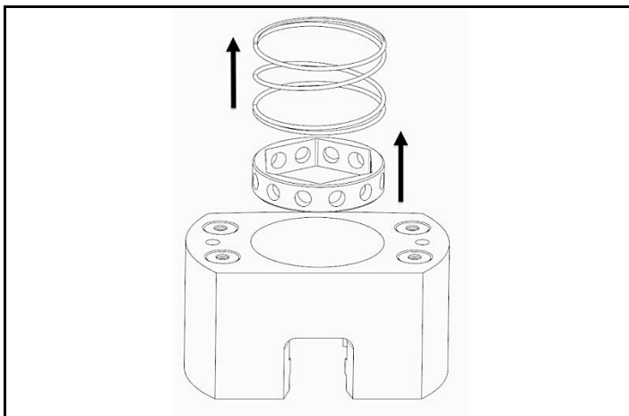
그림 4.12 압축 스프링 및 소켓 제거
