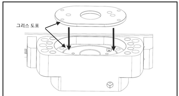
그림 4.10 그리스 도포, 릴리프 밸브 어셈블리 삽입, 스프링 고정판 아래 고정
