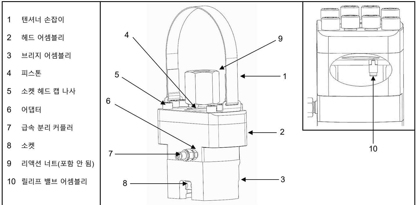
그림 1.1 FTE 시리즈 파운데이션 텐서너(타원형)의 주요 기능 및 구성품
