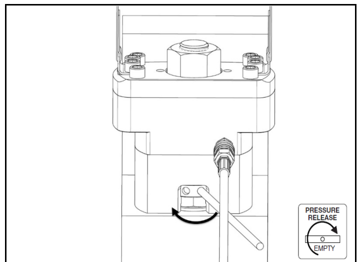
그림 2.6 압력을 유지하여 너트 조이기
