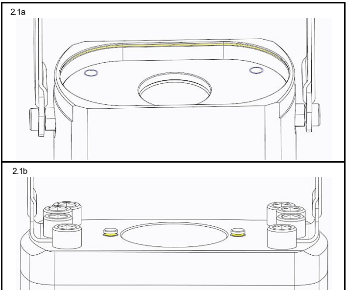
그림 2.1a 최대 스트로크 표시 홈
