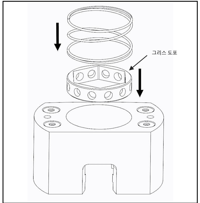
그림 4.13 그리스 도포, 소켓 삽입 후 압축 스프링 삽입
