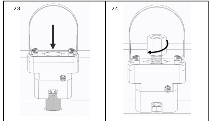
그림 2.3 텐서너를 적용 부분에 배치
