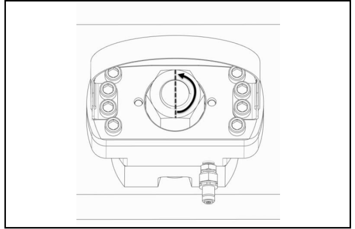
그림 3.1 리액션 너트 조이기 및 1/2 바퀴 뒤로 돌리기
