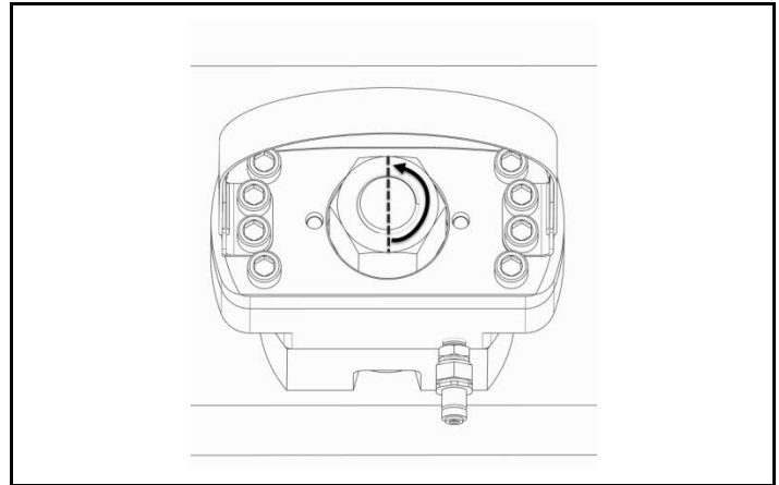
Abb. 3.1 Gegenmutter festziehen und 1/2 Umdrehung zurückdrehen
