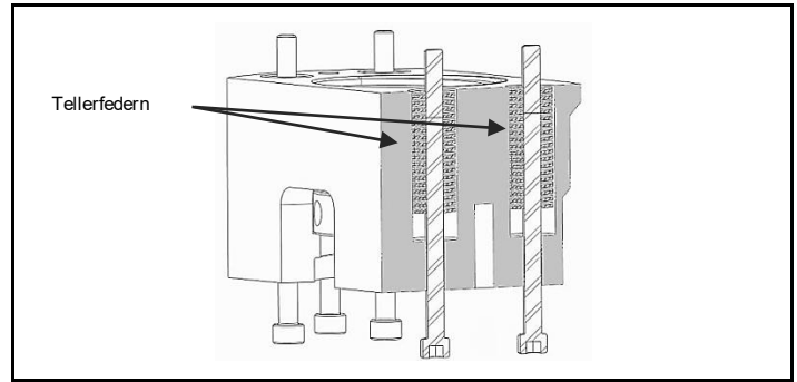
Abb. 4.2 Lage der Tellerfedern in der Brücke
