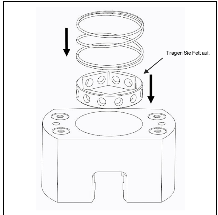
Abb. 4.13 Fett auf die Buchse auftragen und zusammen mit den Druckfedern einsetzen
