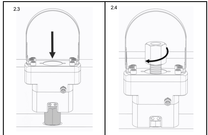
Abb. 2.3 Setzen Sie das Spannwerkzeug auf die Anwendung.
