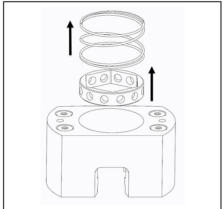
Abb. 4.12 Druckfedern und Buchse entfernen
