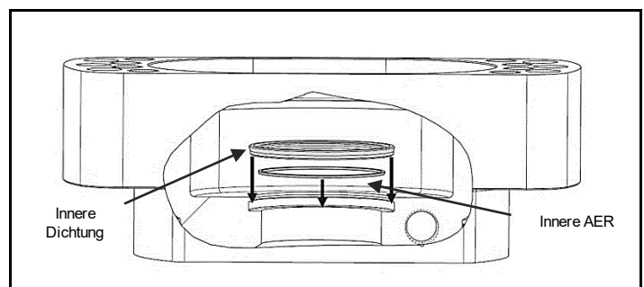
Abb. 4.8 Erst die innere AER und danach die innere Dichtung einsetzen
