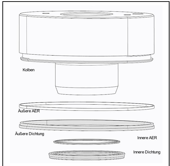
Abb. 4.6. Kolben, äußere AER/Dichtung, innere AER/Dichtung
