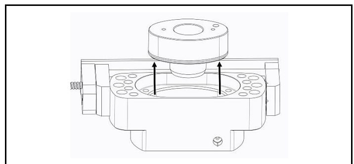
Abb. 4.5 Entfernen des Kolbens, um die Dichtungen zu reinigen und zu ersetzen
