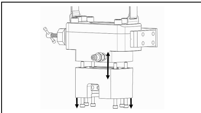
Abb. 4.1 Trennen von Kopfbaugruppe und Brückenbaugruppe
