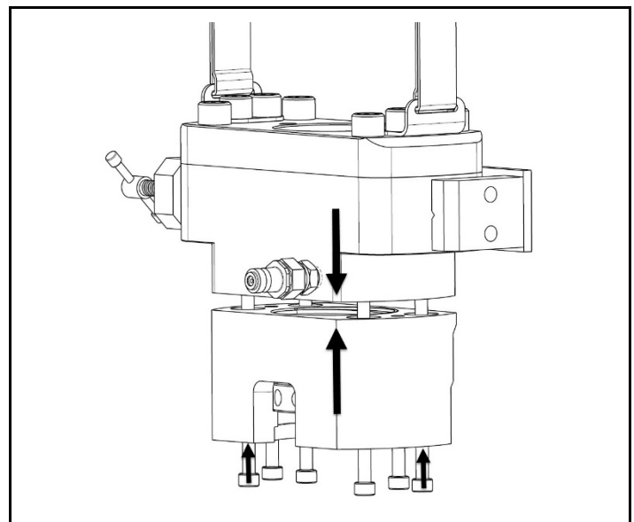
Abb. 4.15 Kopfbaugruppe auf die Brückenbaugruppe setzen und mit den Gewindestiften sichern
