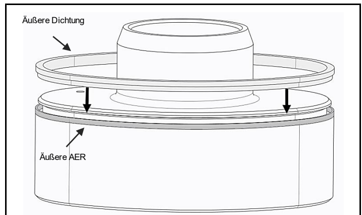
Abb. 4.7 Erst die äußere AER und danach die äußere Dichtung einsetzen
