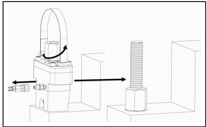
Abb. 2.7 Schlauch lösen, Vorspannwerkzeug entfernen und neu ansetzen
