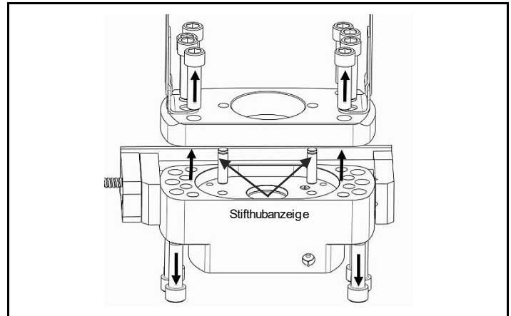
Abb. 4.3 Entfernen der Anschlagplatte, und Ausbau der Stifthubanzeige
