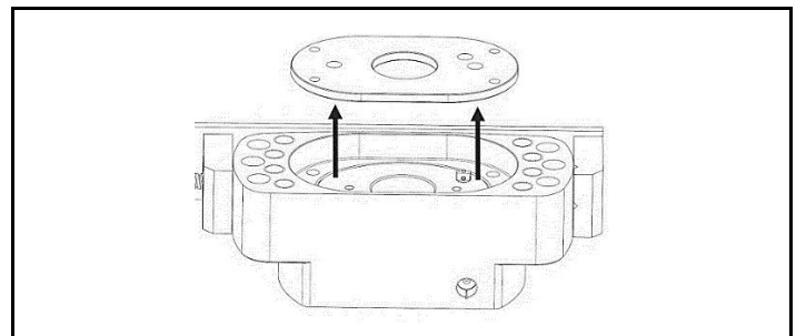
Abb. 4.4 Entfernen der Federhalteplatte, und Ausbau der Stifthubanzeige
