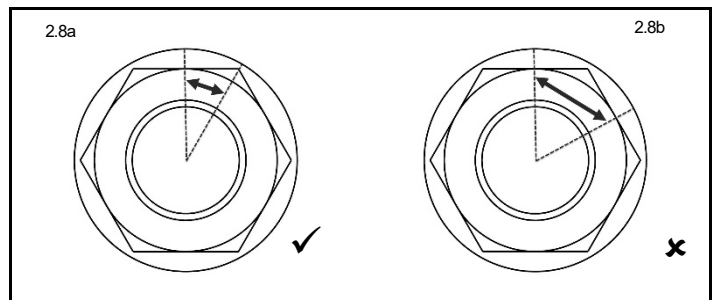
Abb. 2.8a Bolzenspannung vollständig Abb. 2.8b Bolzenspannung unvollständig
