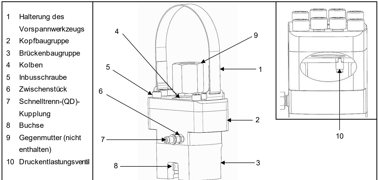
Abb. 1.1 Wichtigste Funktionen und Bauteile des elliptischen hydraulischen Vorspannwerkzeugs der FTE-Serie
