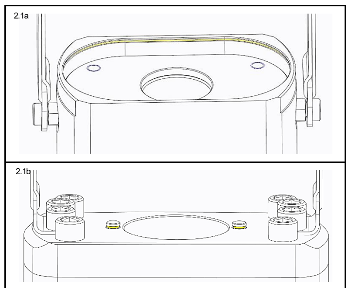
Abb. 2.1a Anzeigenut für maximalen Hub
