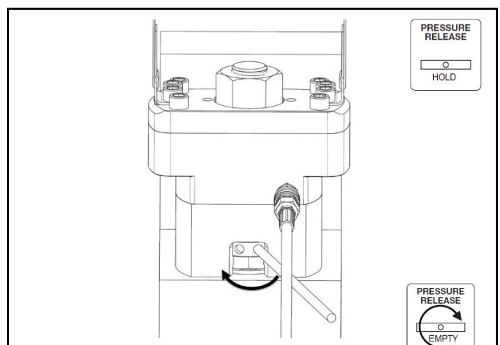
Abb. 2.6 Behalten Sie den Druck bei, um die Mutter festzuziehen.
