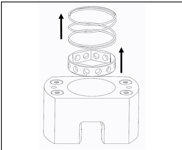
Fig. 4.12 Demontați arcurile de compresie și racordul
