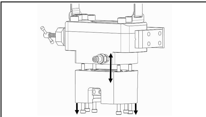
Fig. 4.1 Separarea ansamblului capului și al punții
