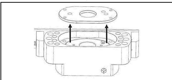
Fig. 4.4 Demontați placa de retenție cu arc și izolați indicatorul de cursă a bolțului
