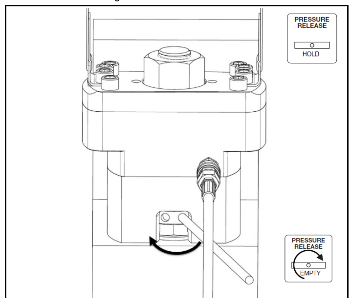
Fig. 2.6 Mențineți presiunea pentru a strânge piulița
