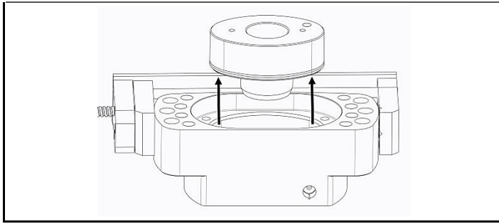
Fig. 4.5 Demontați pistonul pentru a curăța și înlocui garniturile
