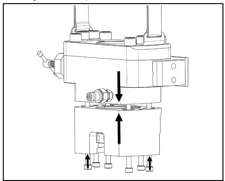
Fig. 4.15 Fixați ansamblul capului pe ansamblul punții, fixați cu șuruburi imbus
