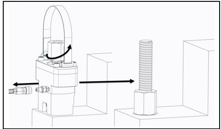
Fig. 2.7 Desfaceți furtunul, demontați și repoziționați dispozitivul de tensionare
