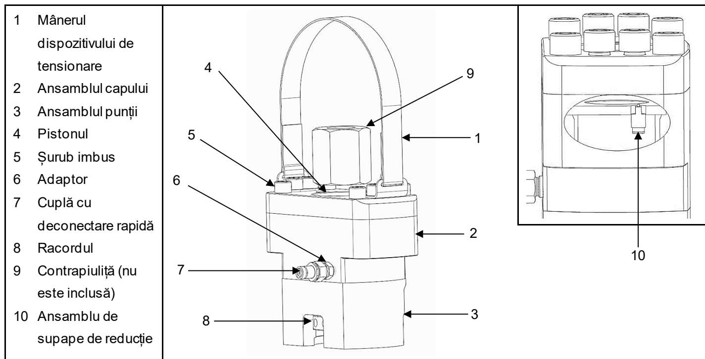
Fig. 1.1 Caracteristicile și componentele principale ale dispozitivelor de tensionare din seria FTE pentru bolțuri de fundație, eliptice
