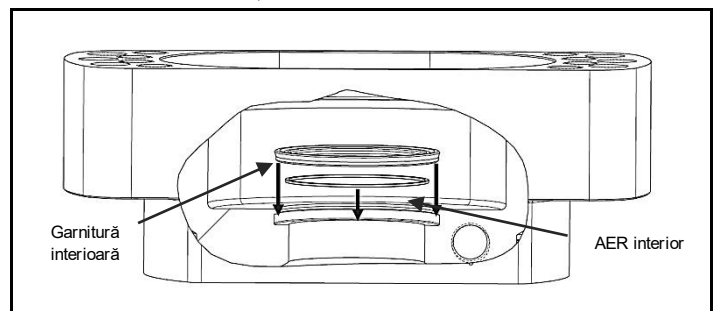
Fig. 4.8 Introduceți AER interior, apoi garnitura interioară
