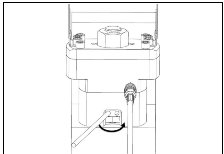
Fig. 3.2 Rotiți contrapiulița în sens antiorar
