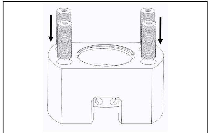
Fig. 4.14 Introduceți arcurile cu disc, dacă au fost scoase
