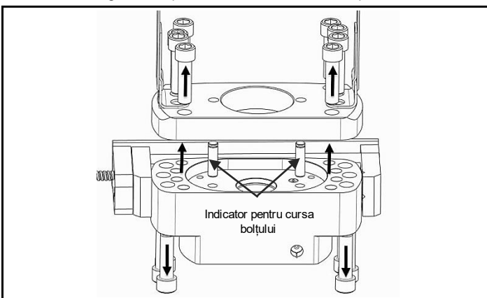
Fig. 4.3 Demontați placa de limitare și izolați indicatorul de cursă a bolțului
