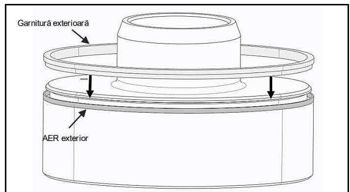
Fig. 4.7 Introduceți AER exterior, apoi garnitura exterioră
