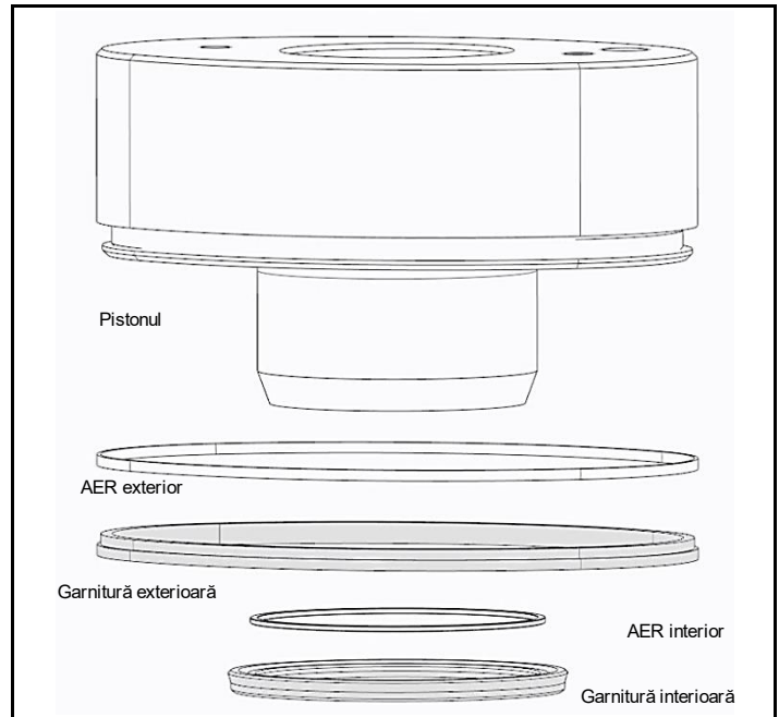
Fig. 4.6 Piston, AER/ garnitură exterior(-oară), AER/ garnitură interior(-oară)
