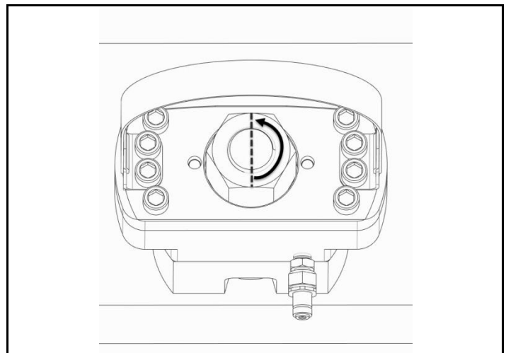
Fig. 3.1 Strângeți contrapiulița și rotiți-o înapoi 1/2 de tură
