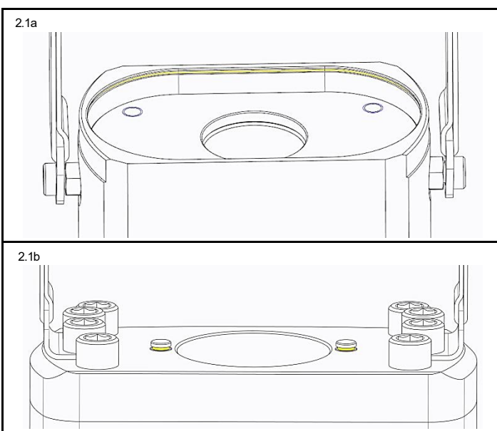
Fig. 2.1a Șanțul indicator pentru cursa maximă
