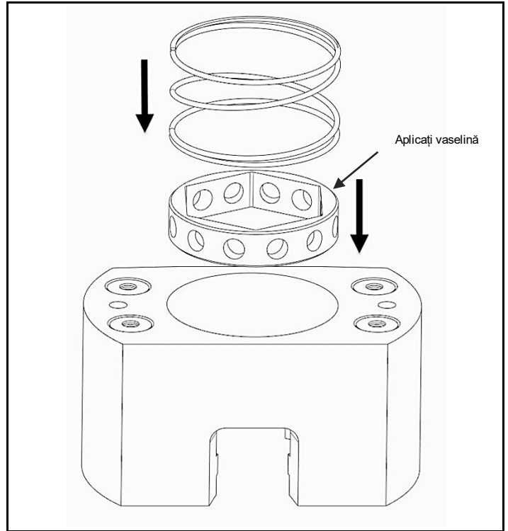
Fig. 4.13 Gresați și introduceți racordul, apoi arcurile de compresie
