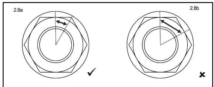
Fig. 2.8a Tensionarea boltului finalizată
