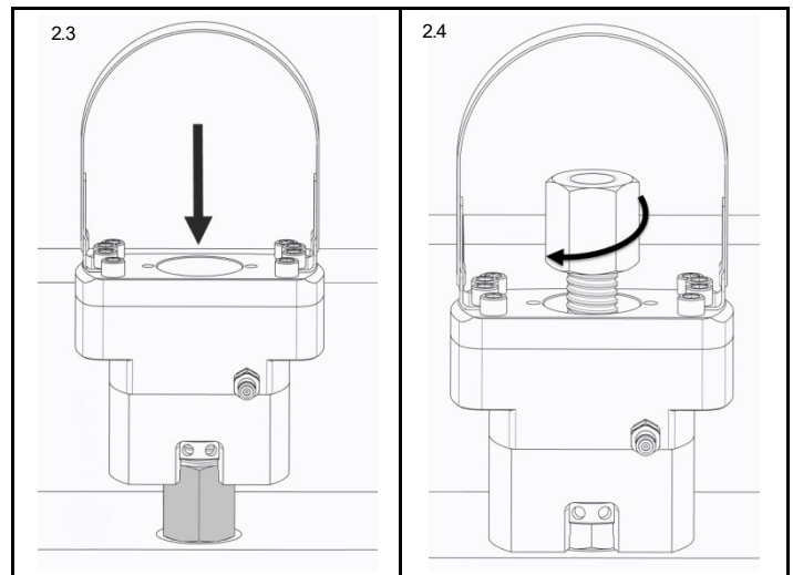
Fig. 2.3 Amplasarea dispozitivului de tensionare pe aplicație
