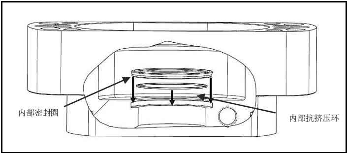
图 4.8 插入内部密封圈，然后插入内部抗挤压环
