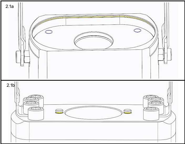
图 2.1a 最大行程指示槽 图 2.1b 行程指示销上指示槽
