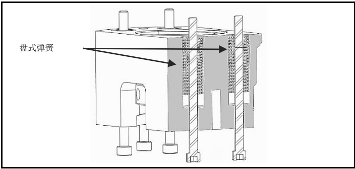
图 4.2 盘式弹簧在座桥总成内的位置
