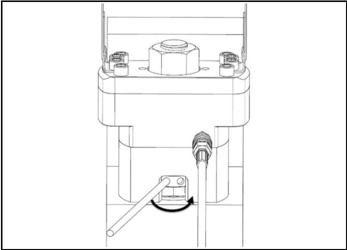
图 3.2 逆时针转动反应螺母
