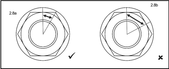
图 2.8a 螺栓旋紧已完成
