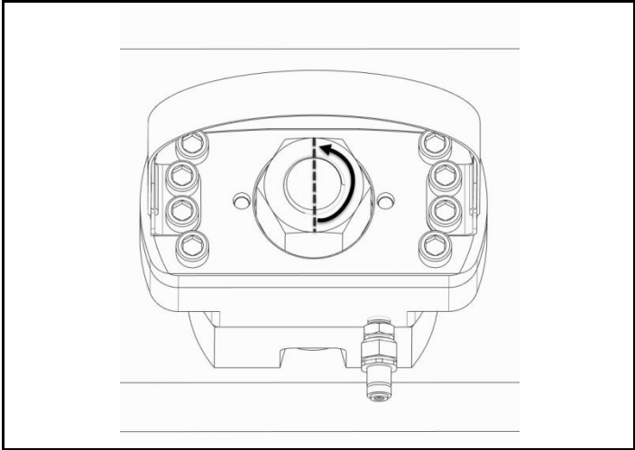
图 3.1 旋紧反应螺母，然后回旋 1/2 圈
