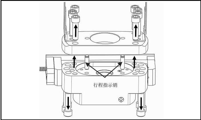
图 4.3 拆下限位板，与行程指示销脱离
