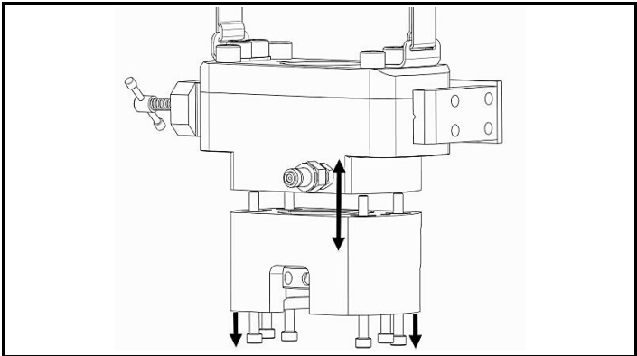
图 4.1 拉伸头总成和座桥总成分离
