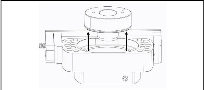
图 4.5 拆下活塞，进行清理和密封件更换
