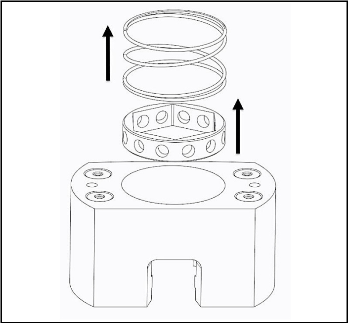
图 4.12 拆下压缩弹簧和套筒头
