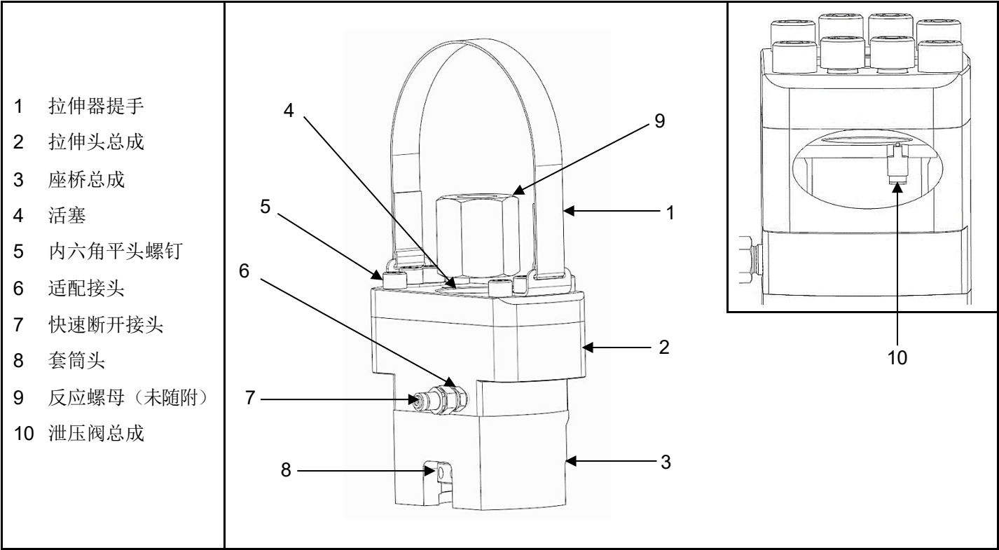
图 1.1 FTE-系列椭圆形基础拉伸器主要特性和部件
