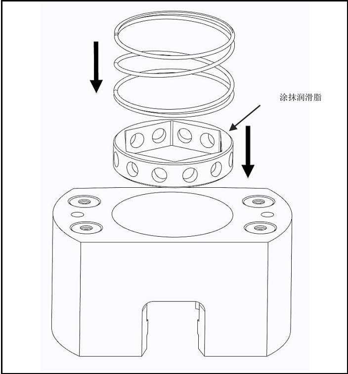
图 4.13 润滑并插入套筒头，然后润滑并装回压缩弹簧。
