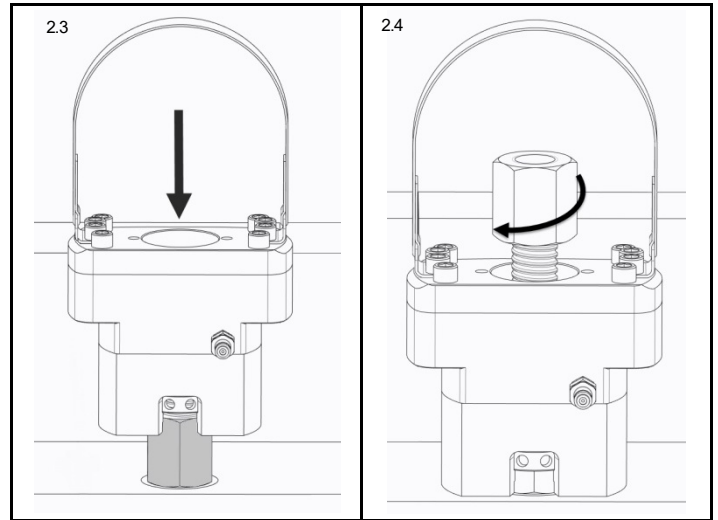
图 2.3 将拉伸器放到目标上
