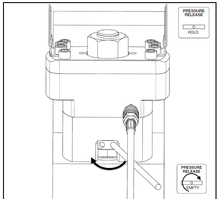
图 2.6 保持压力以旋紧螺母
