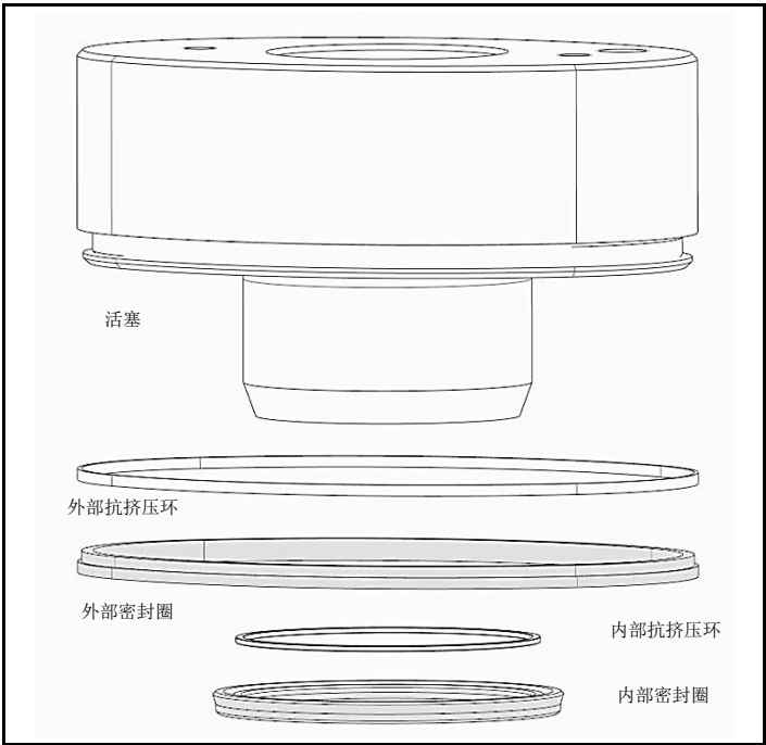
图 4.6 活塞、外部抗挤压环/密封圈、内部抗挤压环/密封圈
