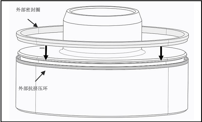
图 4.7 插入外部抗挤压环，然后插入外部密封圈
