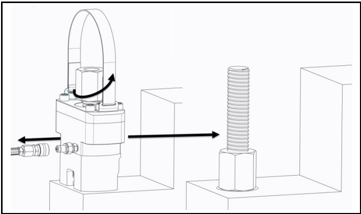
图 2.7 断开软管并重新放置拉伸器
