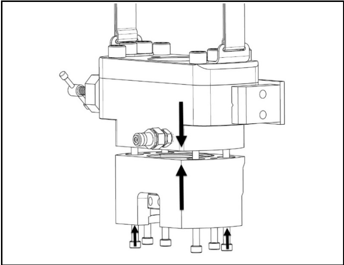
图 4.15 将拉伸头总成放置到座桥总成上，使用内六角平头螺钉固定
