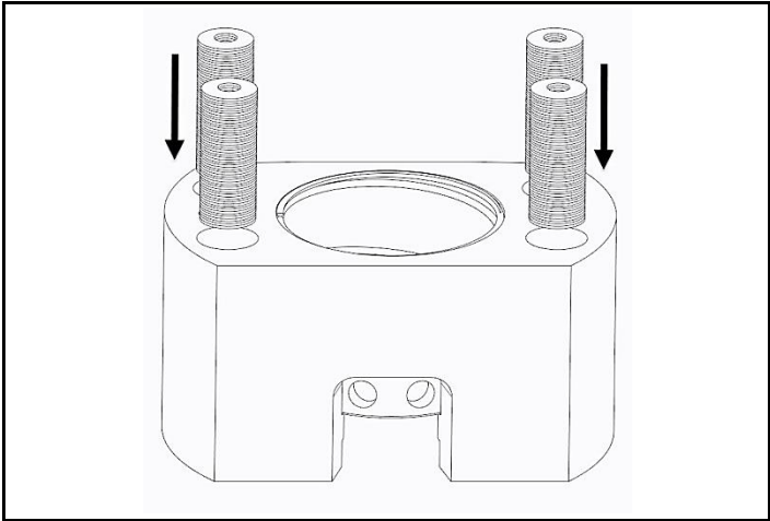
图 4.14 插入盘式弹簧，如果先前被拆下的话
