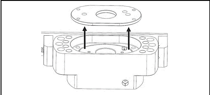
图 4.4 拆下弹簧固定板，与行程指示销脱离
