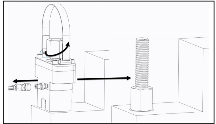
Fig. 2.7 Débrancher le flexible, puis retirer et repositionner le tendeur
