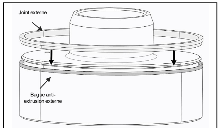
Fig. 4.7 Introduire la bague anti-extrusion externe, suivie du joint externe
