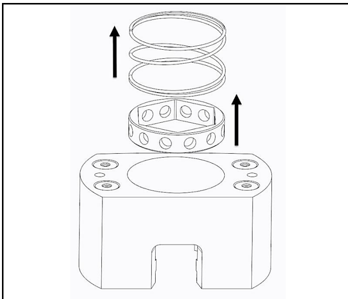
Fig. 4.12 Retirer les ressorts de compression et la douille
