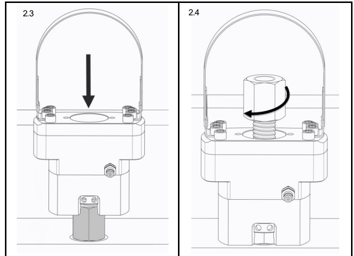
Fig. 2.3 Placer le tendeur sur l'application
