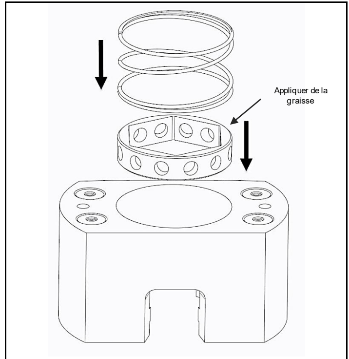
Fig. 4.13 Graisser et introduire la douille, suivie des ressorts de compression
