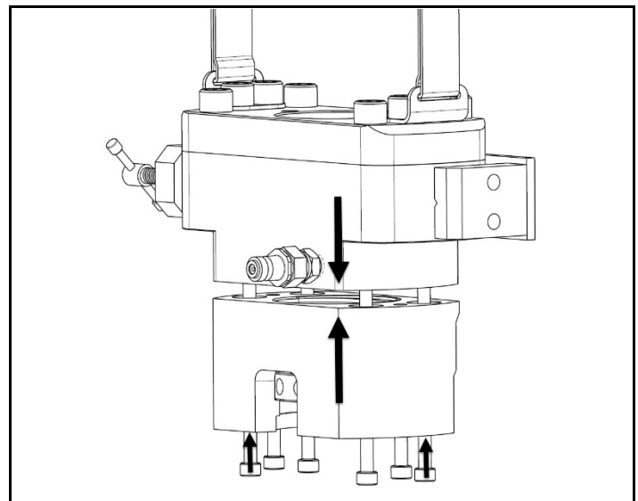
Fig. 4.15 Placer l'ensemble tête sur l'ensemble pont ; fixer avec des vis creuses
