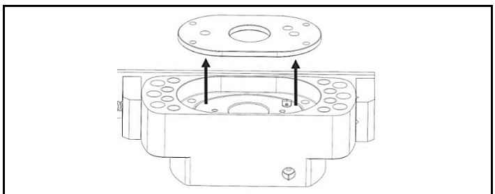
Fig. 4.4 Retirer la plaque de retenue des ressorts et isoler l'indicateur de course à goupille
