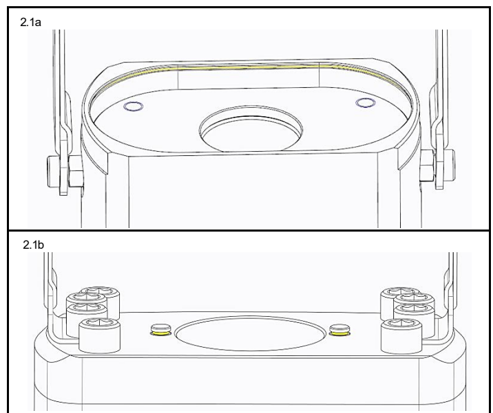
Fig. 2.1a Rainure de course maximale
