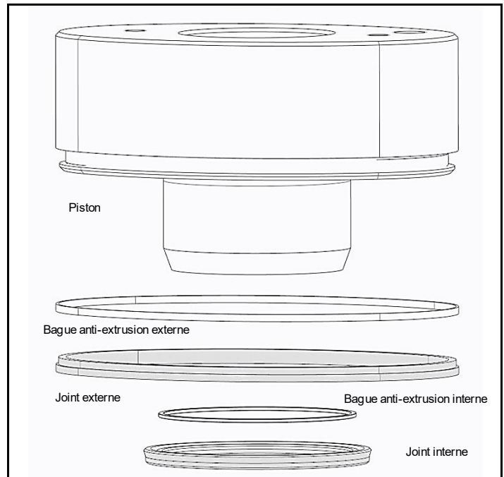
Fig. 4.6 Piston, bague/joint externes, bague/joint internes
