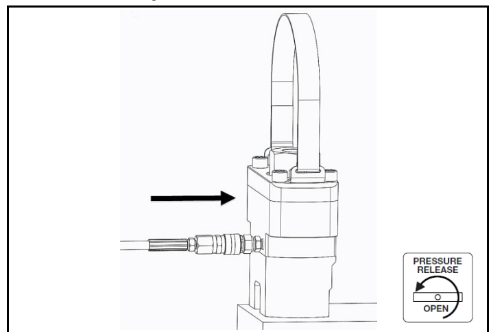
Fig. 2.5 Raccordement du flexible
