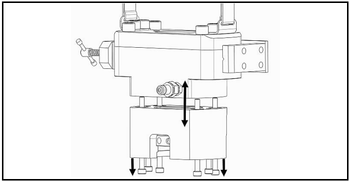
Fig. 4.1 Séparer les ensembles tête et pont
