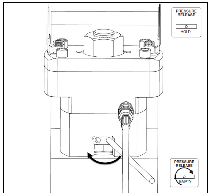
Fig. 2.6 Maintenir la pression pour serrer l'écrou
