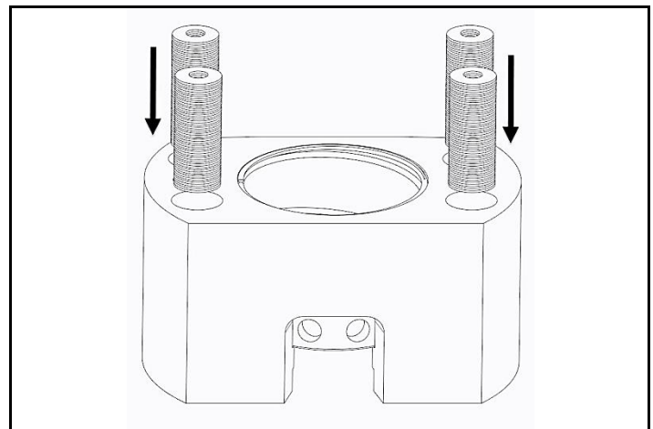
Fig. 4.14 Introduire les ressorts à disques s'ils ont été retirés
