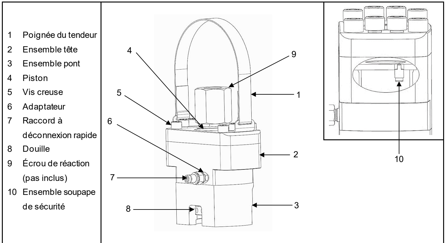
Fig. 1.1 Caractéristiques et composants principaux des tendeurs de boulons de fondation elliptiques de la série FTE
