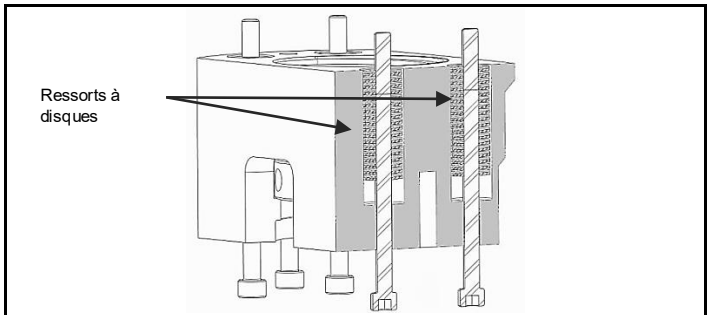
Fig. 4.2 Emplacement des ressorts à disques dans le pont
