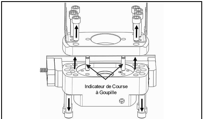
Fig. 4.3 Retirer la plaque de limitation et isoler l'indicateur de course à goupille
