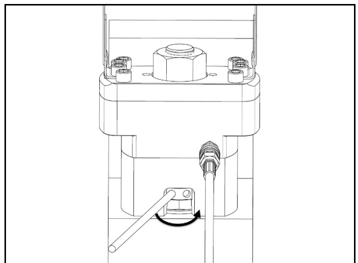
Fig. 3.2 Tourner l'écrou de réaction dans le sens inverse des aiguilles d'une montre
