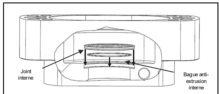
Fig. 4.8 Introduire le joint interne, suivi de la bague anti-extrusion interne
