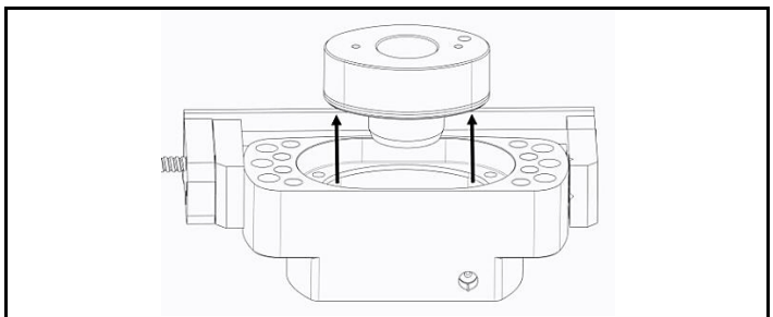
Fig. 4.5 Retirer le piston pour le nettoyage et le remplacement des joints
