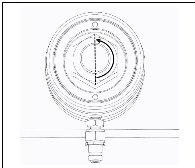
Fig. 3.1 Spænd reaktionsmøtrikken, og drej 1/2 omgang tilbage
