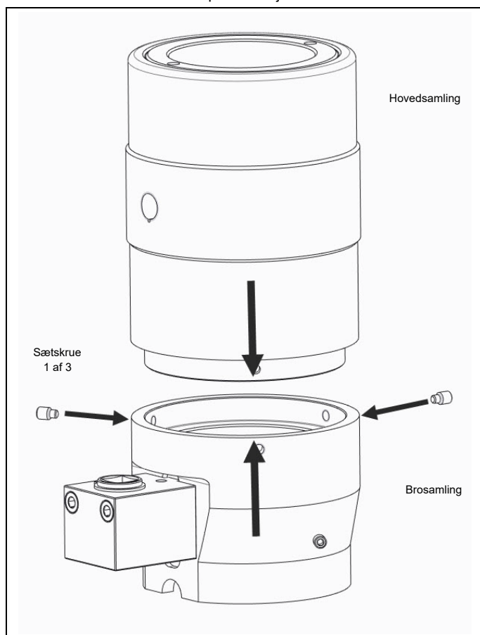
Fig. 4.26 Anbring hovedsamlingen på brosamlingen, sikres med sætskrue
