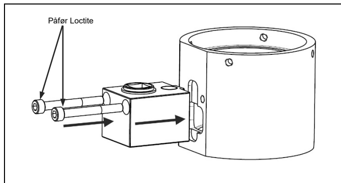
Fig. 4.24 Kom Loctite på maskinskrue, fastgør samlet gearkasse på bro
