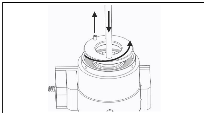
Fig. 4.2 Fjern fjederskive
