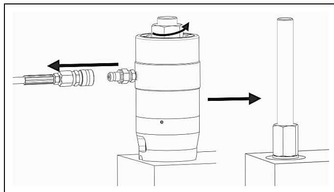
Fig. 2.8 Afkobling af slange, fjern og flyt spænder
