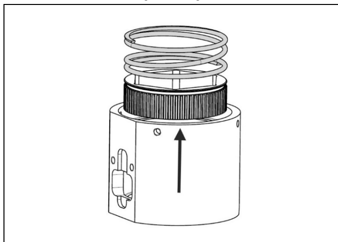
Fig. 4.14 Fjern drivaksel
