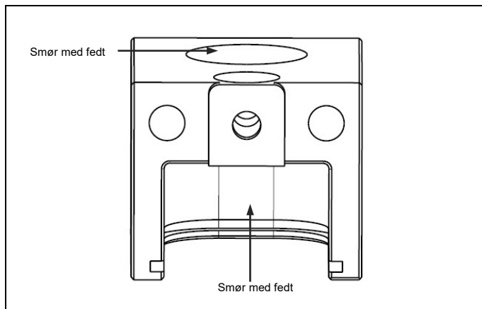
Fig. 4.16 Forbered gearkassehuset
