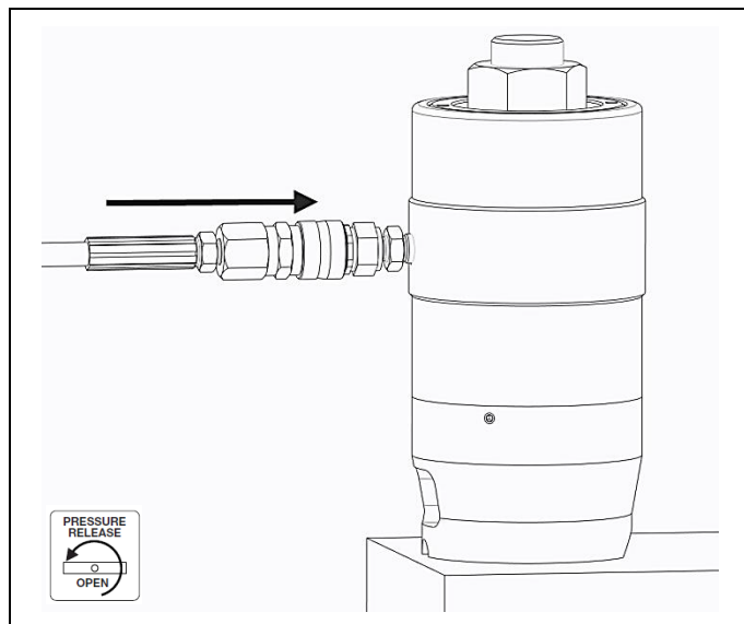
Fig. 2.5 Slangeforbindelse
