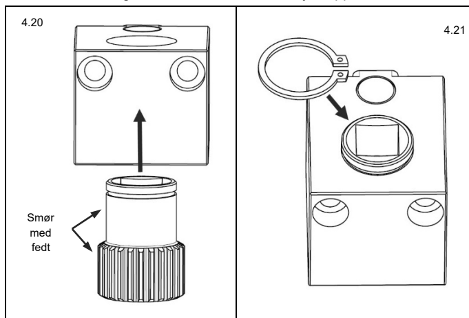
Fig. 4.20 Forbered og installer drivhjul
