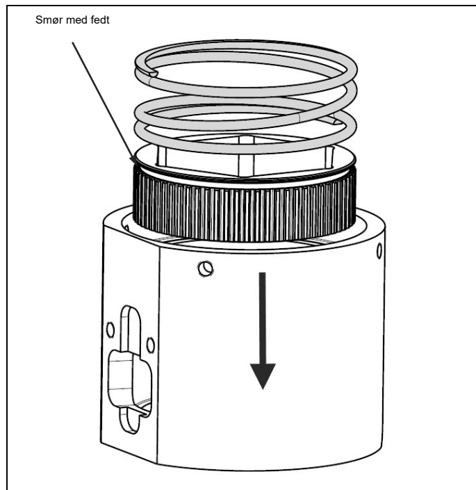
Fig. 4.15 Undersøg, om broens interne dele sidder rigtigt, smør med fedt
