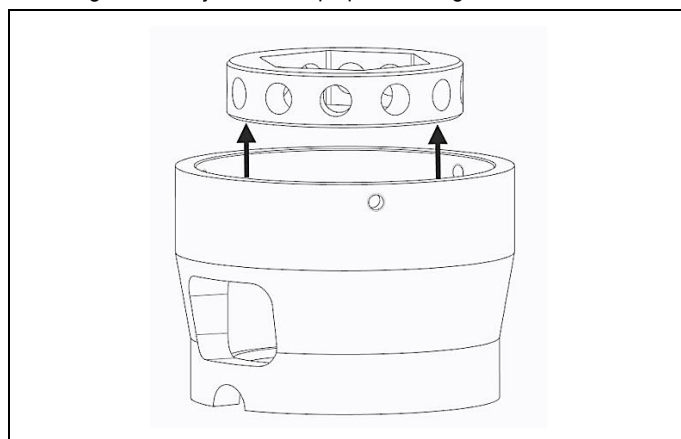
Fig. 4.9 Fjern aksel fra bro
