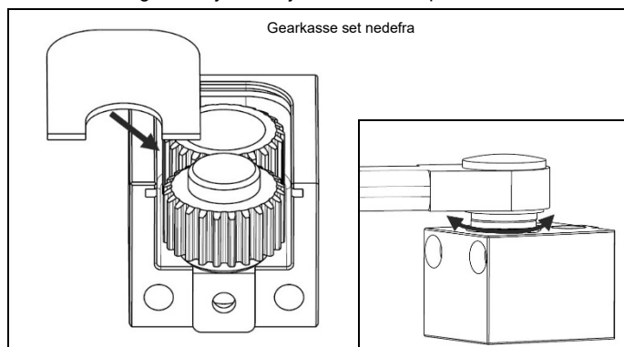
Fig. 4.23 Påsæt gearkassedæksel, tjek om hjulene kører let
