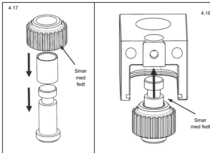
Fig. 4.17 Smør og saml mellemste gear
