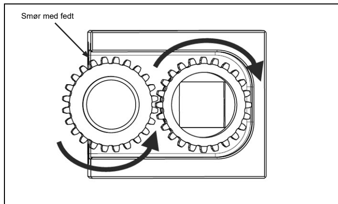
Fig. 4.22 Tjek om hjulene kører let, påfør fedt
