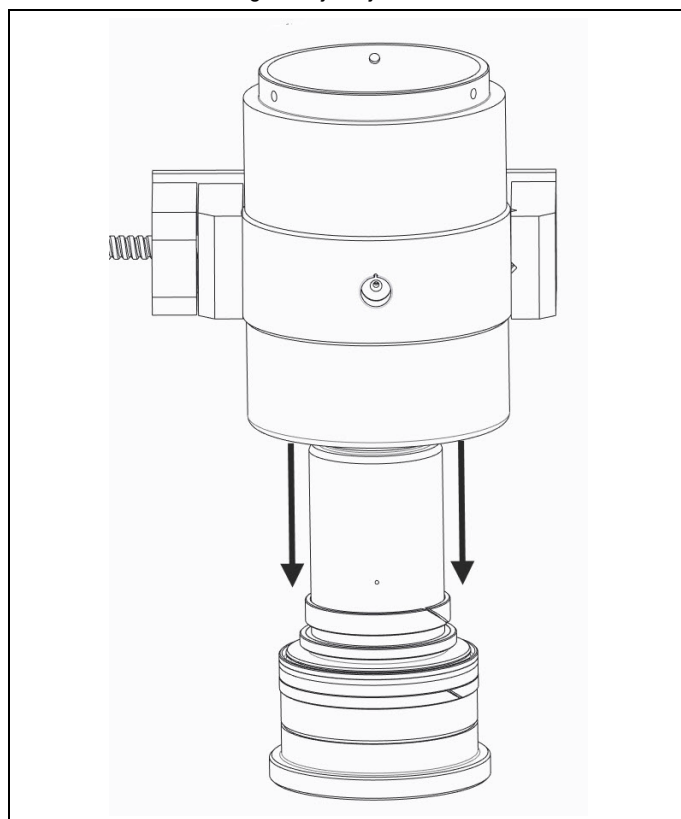
Fig. 4.3 Stempel fjernet fra krop
