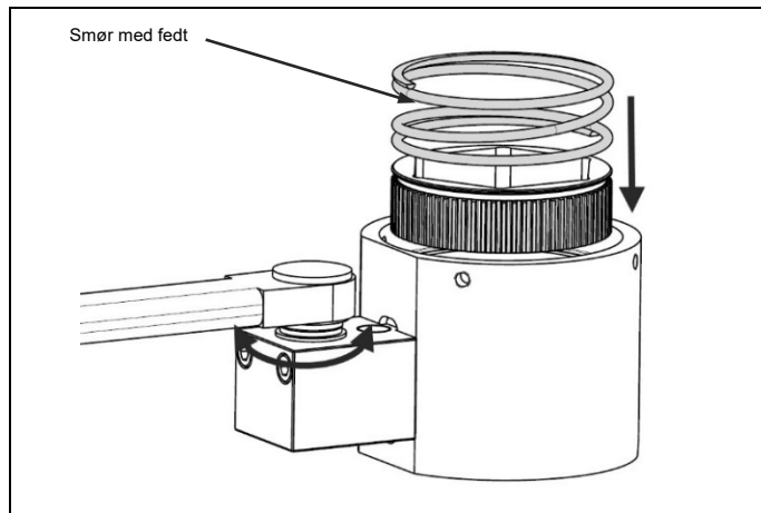
Fig. 4.25 Smør med fedt, og indsæt drivende aksel, efterfulgt af kompressionsfjedre
