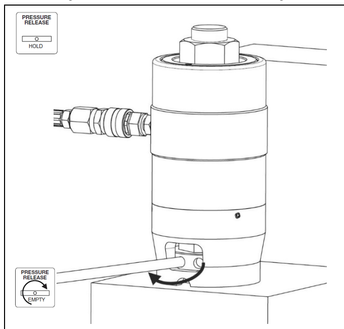
Fig. 2.7 Hold trykket for at spænde møtrikken
