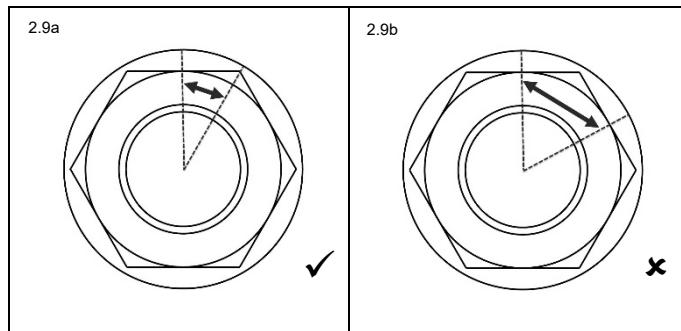
Fig. 2.9a Boltspænding færdig
