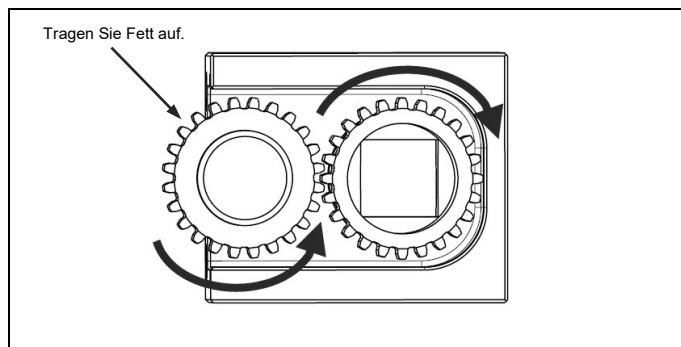
Abb. 4.22 Kontrollieren, ob die eingebauten Zahnräder reibungslos laufen, und Fett auftragen
