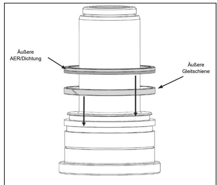
Abb. 4.5 Erst die äußere AER und danach die äußere Dichtung einsetzen
