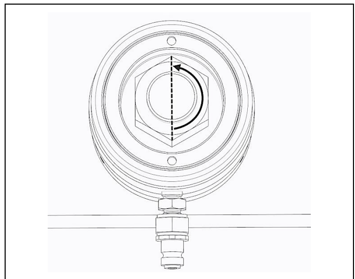
Abb. 3.1 Gegenmutter festziehen und eine 1/2 Umdrehung zurückdrehen
