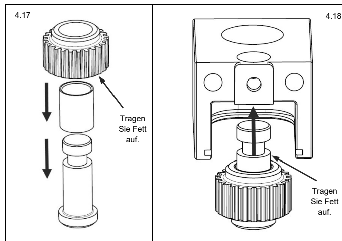
Abb. 4.17 Fett auf das Zwischengetriebe auftragen und montieren
