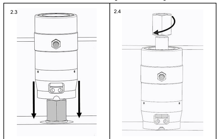
Abb. 2.3 Vorspannwerkzeug auf die Anwendung setzen
