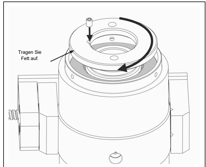
Abb. 4.8 Federteller in seine richtige Position schrauben und mit der Stellschraube sichern
