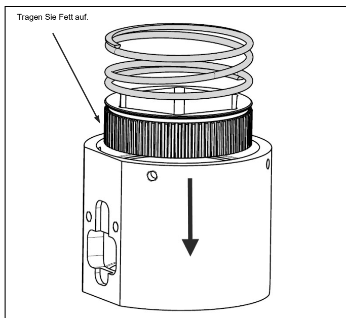
Abb. 4.15 Prüfen, ob die Innenteile der Brücke korrekt zusammenpassen, und Fett auftragen
