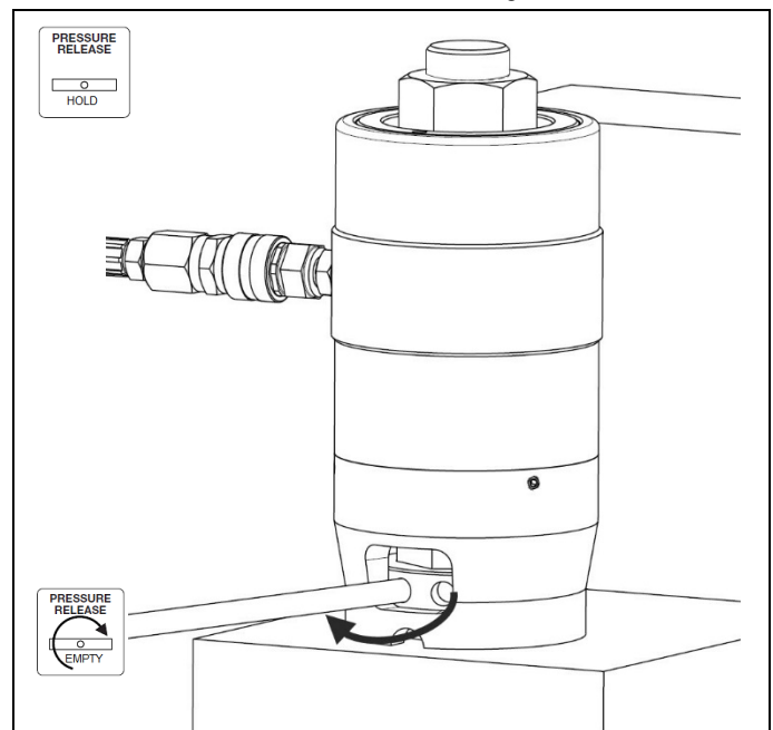
Abb. 2.7. Druck beibehalten, um die Mutter festzuziehen
