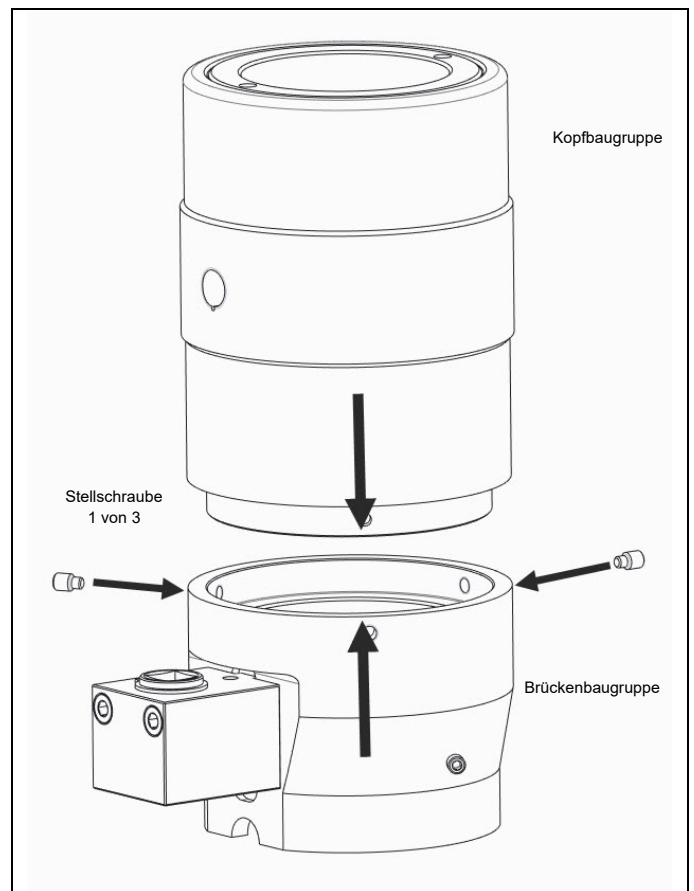
Abb. 4.26 Die Kopfbaugruppe auf die Brückenbaugruppe aufsetzen und mit Gewindestiften sichern
