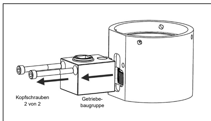
Abb. 4.10 Trennung von Brücken- und Getriebebaugruppe
