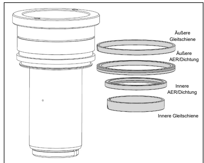
Abb. 4.4 Kolben, äußere AER/Dichtung, innere AER/Dichtung, Gleitschienen
