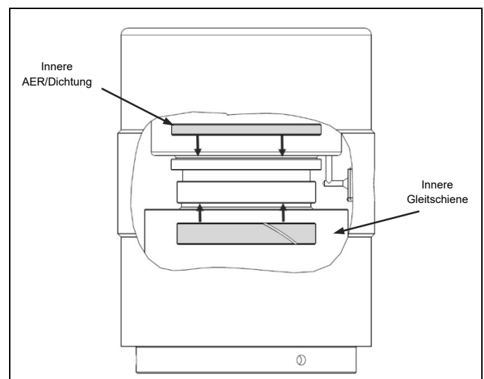
Abb. 4.6 Erst die innere AER und danach die innere Dichtung einsetzen
