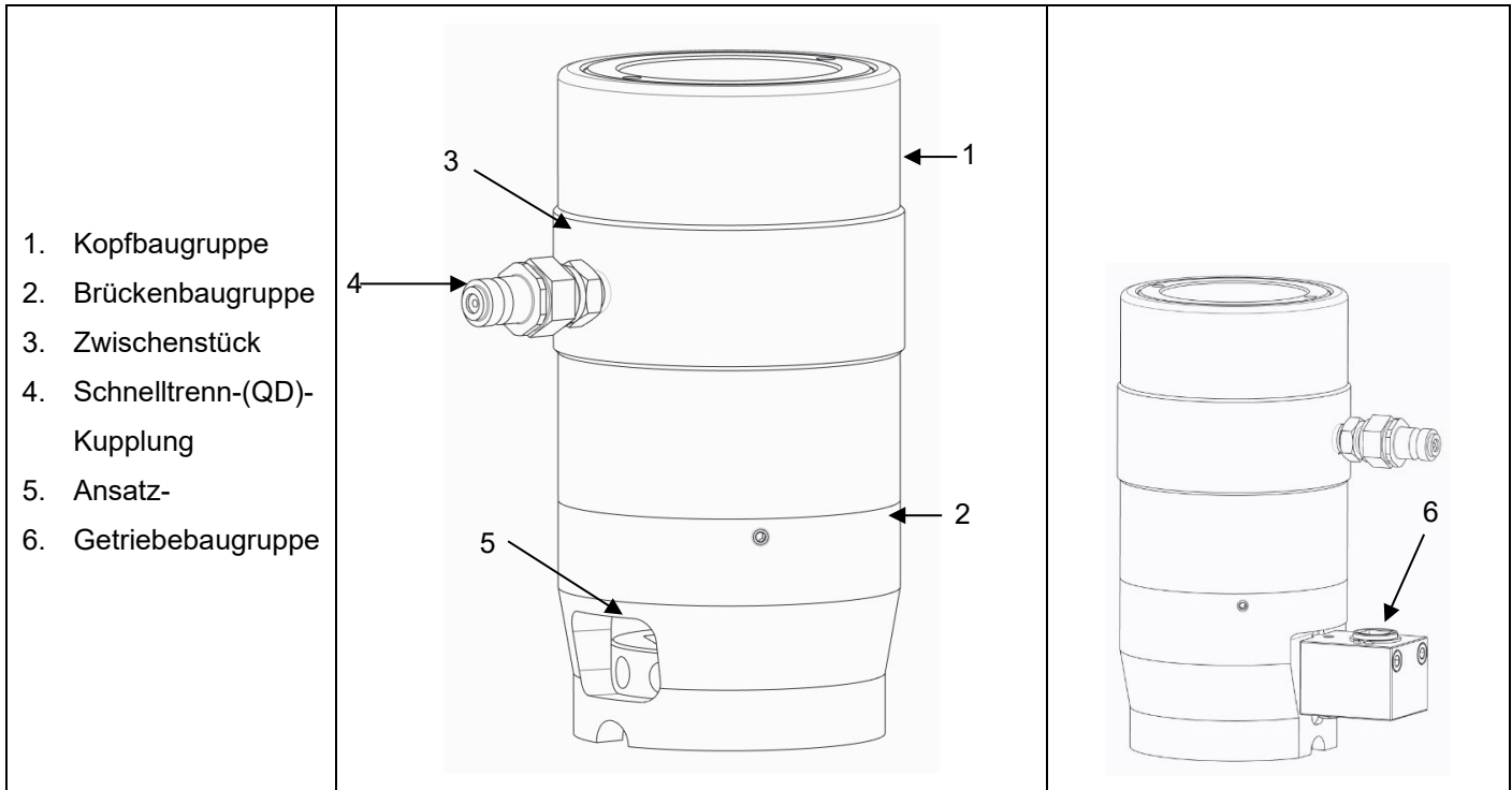
Abb. 1.1. Wichtigste Funktionen und Bauteile der runden hydraulischen Vorspannwerkzeuge der FTR-Serie
