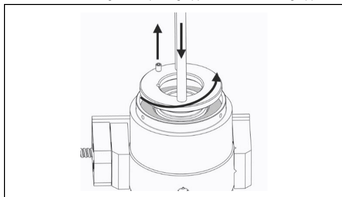
Abb. 4.2 Entfernen des Federtellers
