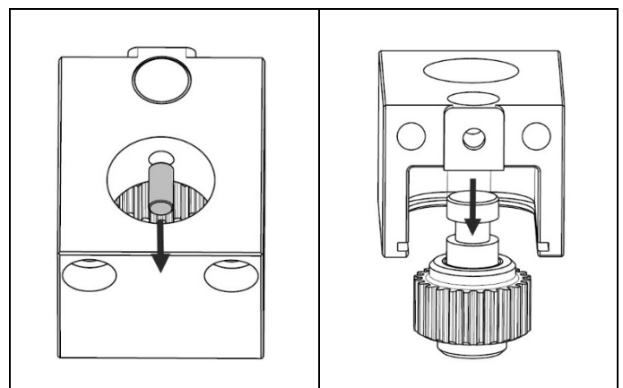
Abb. 4.13 Sicherungsstift entfernen und Zwischengetriebe montieren
