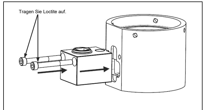
Abb. 4.24 Lactite auf die Kopfschrauben auftragen, das montierte Getriebe an der Brücke sichern
