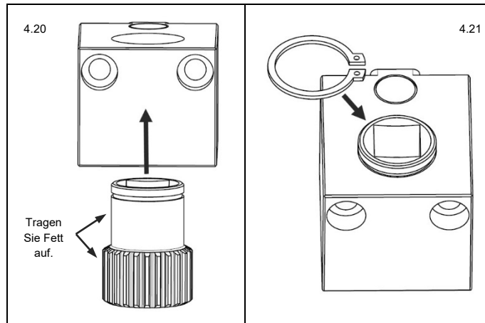
Abb. 4.20 Antriebsrad vorbereiten und montieren
