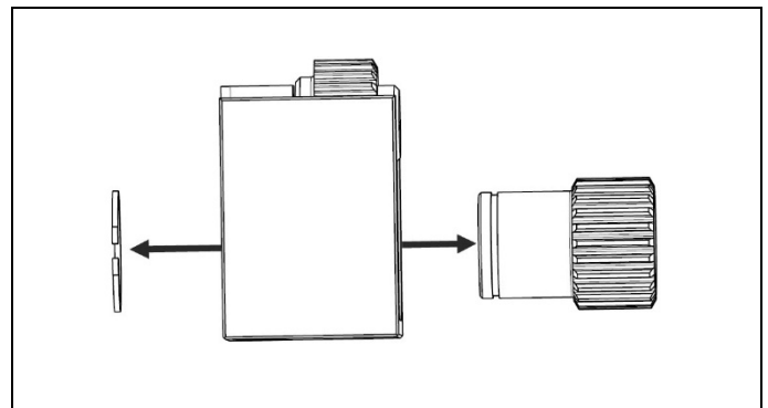
Abb. 4.12 Sicherungsring des Antriebszahnrad und Antriebszahnrad entfernen
