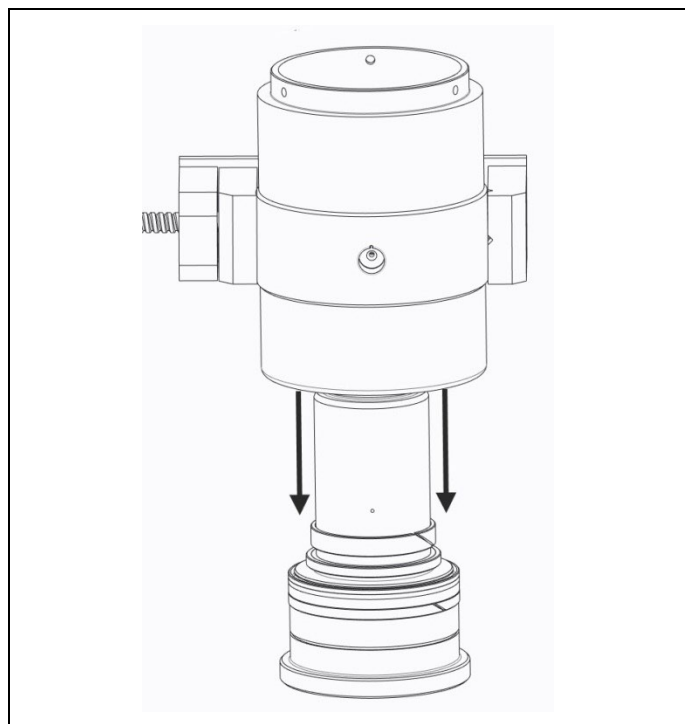
Abb. 4.3 Entfernen des Kolbens vom Körper
