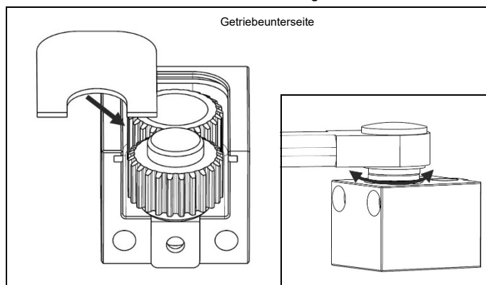
Abb. 4.23 Getriebedeckel aufsetzen, und Getriebe auf Leichtigkeit prüfen
