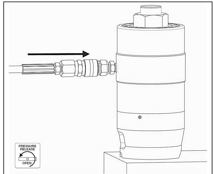
Abb. 2.5 Schlauchanschluss
