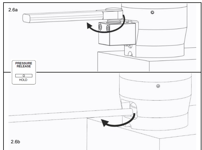
Abb. 2.6a Buchse mit Getriebe festziehen
