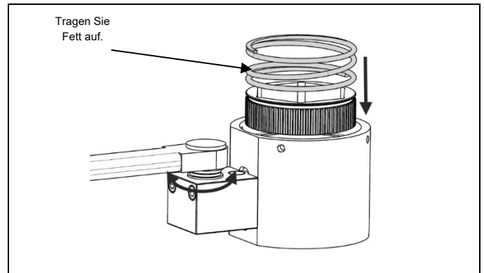
Abb. 4.25 Fett auftragen, und die Getriebebuchse zusammen mit den Druckfedern einsetzen
