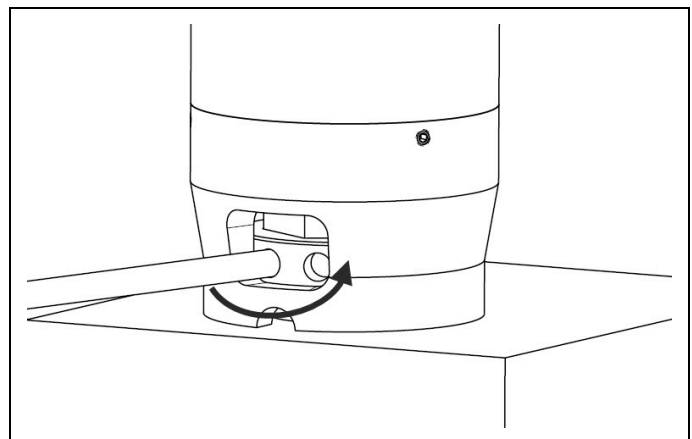
Abb. 3.2 Gegenmutter gegen den Uhrzeigersinn drehen
