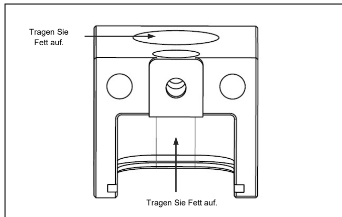
Abb. 4.16 Getriebegehäuse vorbereiten
