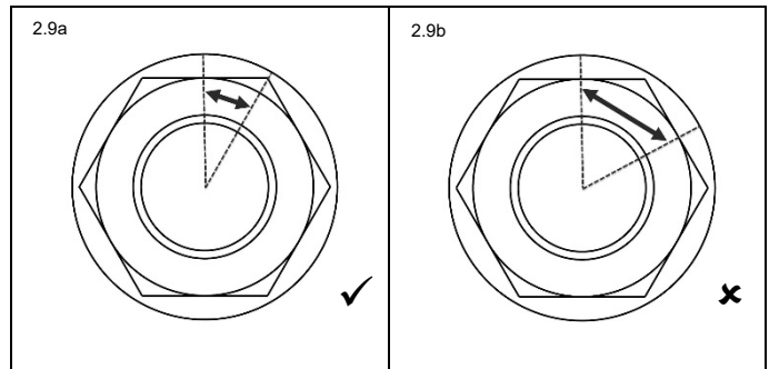
Abb. 2.9a Bolzenspannung vollständig
