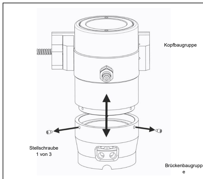
Abb. 4.1 Trennung von Kopfbaugruppe und Brückenbaugruppe
