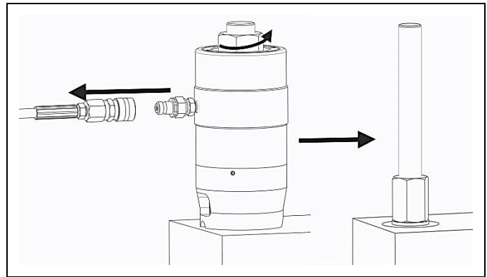
Abb. 2.8 Schlauch lösen, Vorspannwerkzeug entfernen und neu ansetzen
