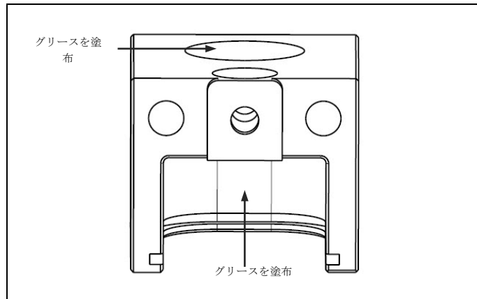
図 4.16 ギアボックスハウジングの準備
