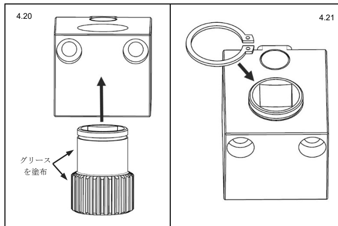
図 4.20 ドライブギアの準備および取り付け
