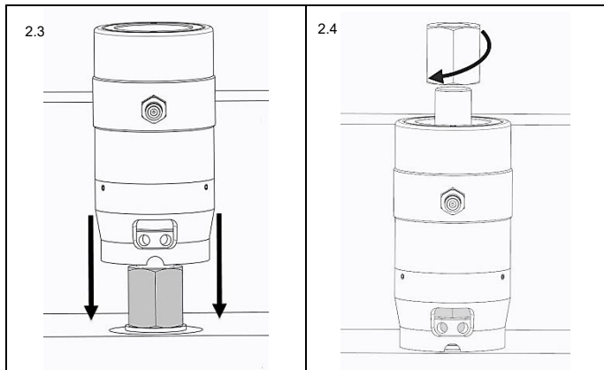
図 2.3 適用対象へのテンショナーの配置
