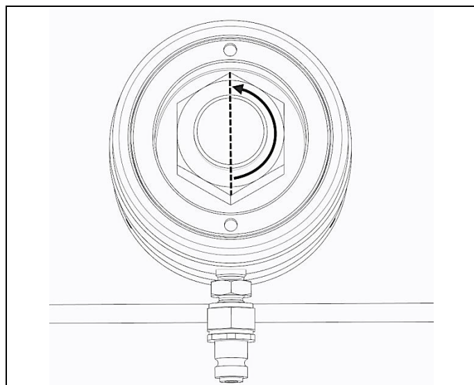
図 3.1 リアクションナットの締め付け、および 1/2 戻した締め付け
