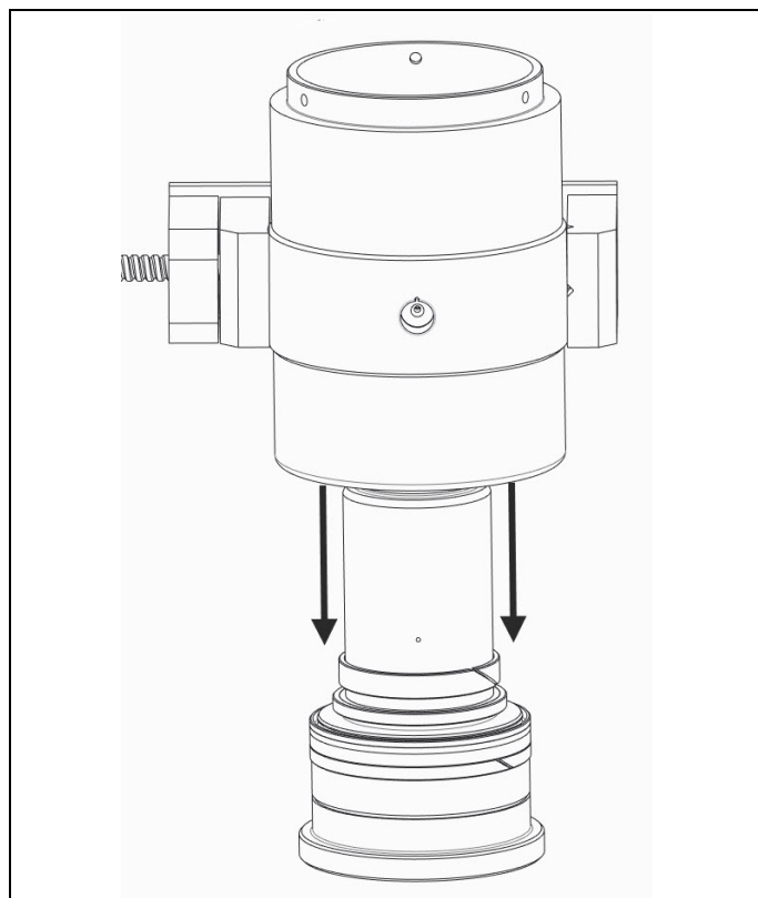
図 4.3 ボディからピストンを取り外した状態
