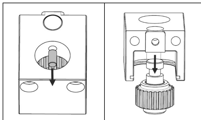
図 4.13 中間ギアアセンブリの取り外しの後、固定ダウエルピンの取り外し
