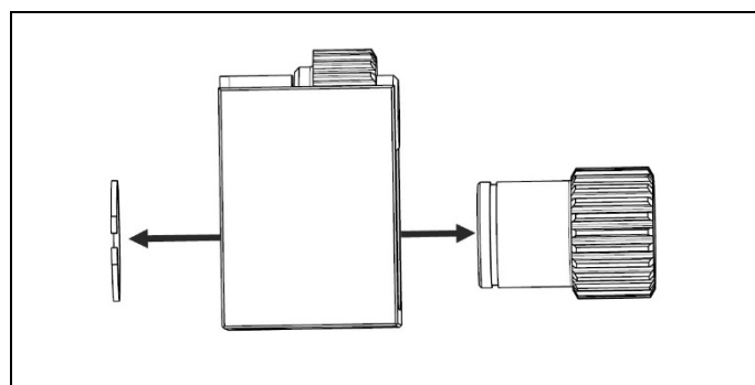
図 4.12 ドライブギアサークリップとドライブギアの取り外し
