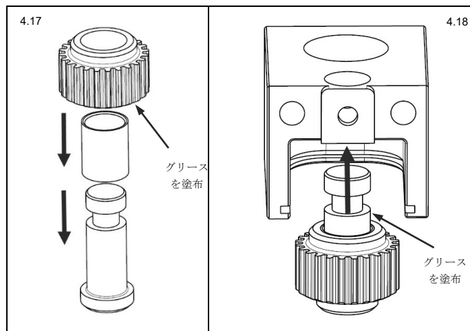
図 4.17 中間ギアの潤滑および組み立て
