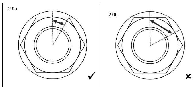
図 2.9a ボルトテンショニング完了
