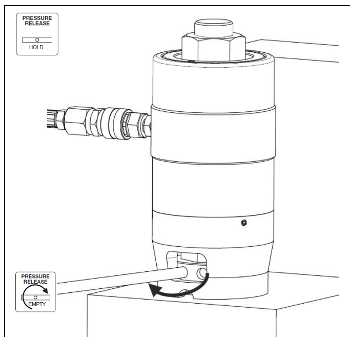
図 2.7 圧力を維持してナットを締め付け
