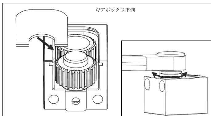
図 4.23 ギアボックスカバーの取り付け、ギアがスムーズに回転するかどうかの点検
