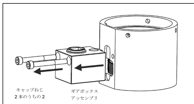
図 4.10 ブリッジアセンブリとギアボックスアセンブリの分離
