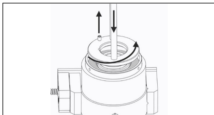
図 4.2 スプリングカラーの取り外し
