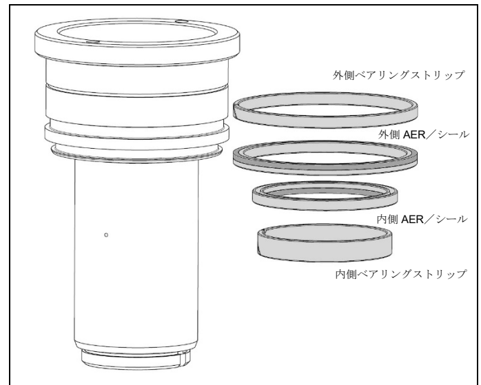
図 4.4 ピストン、外側 AER/シール、内側 AER/シール、ベアリングストリップ
