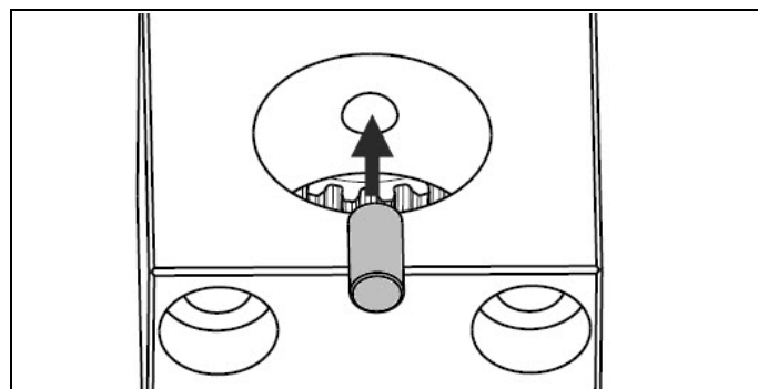
図 4.19 固定ダウエルピンの挿入
