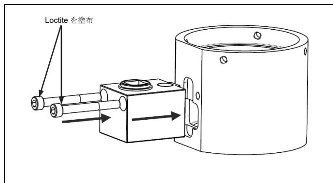
図 4.24 キャップねじへの Loctite の塗布、組み立てられたギアボックスのブリッジへの固定
