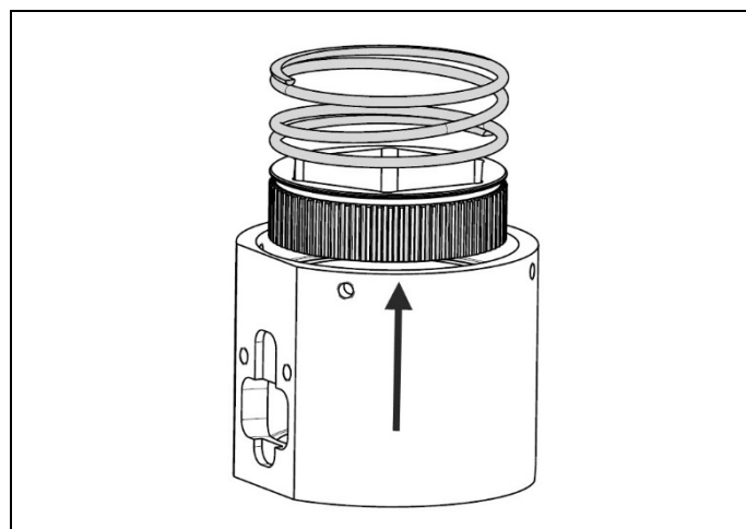
図 4.14 ギアボックスカバーの取り外し
