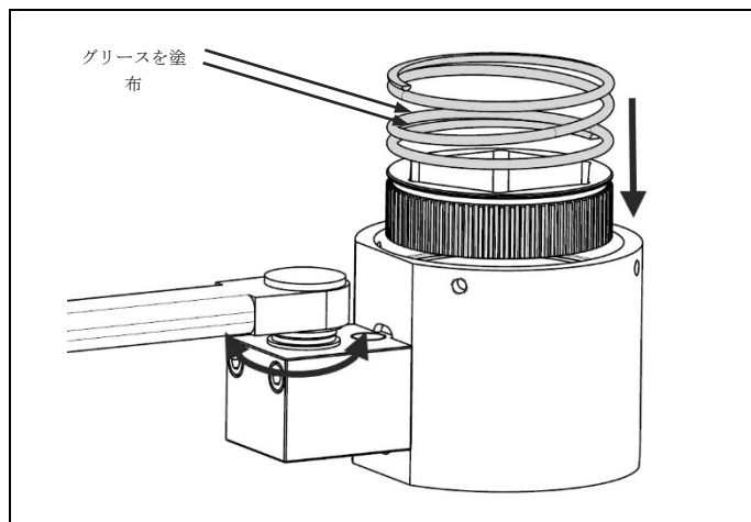
図 4.25 グリースの塗布、ギア付きソケットの挿入後、圧縮スプリングの挿入
