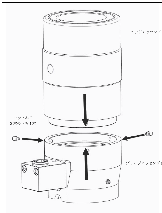
図 4.26 ヘッドアセンブリのブリッジアセンブリへの配置、セットねじでの固定
