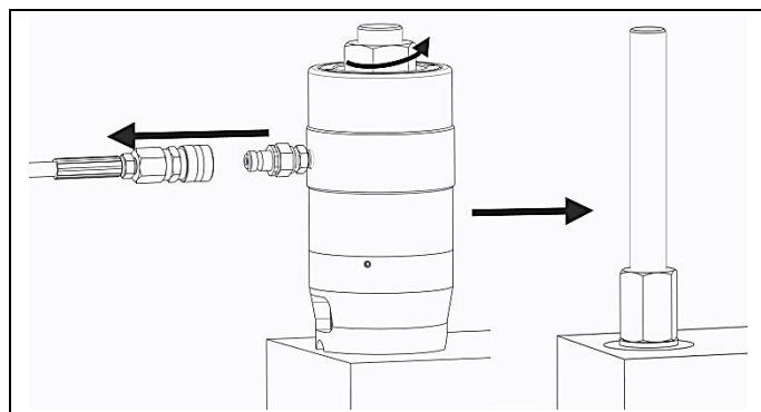
図 2.8 ホースの取り外し、テンショナーの取り外しおよび再配置
