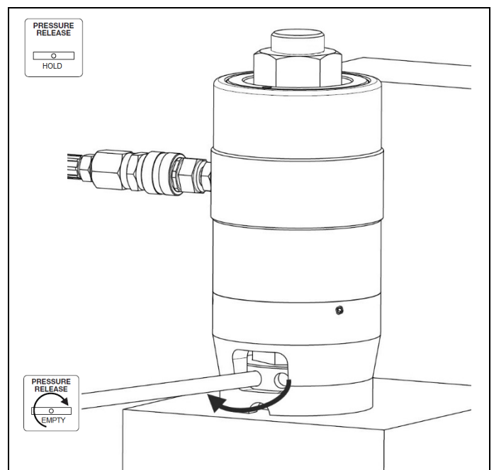
Kuva 2.7 Pidä paine mutterin kiristystä varten
