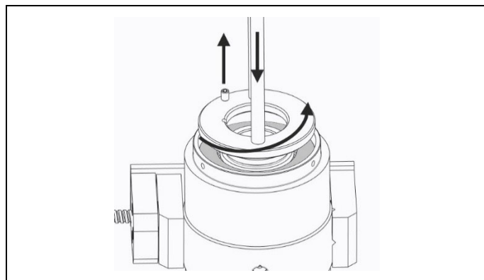
Kuva 4.2 Poista joustorengas
