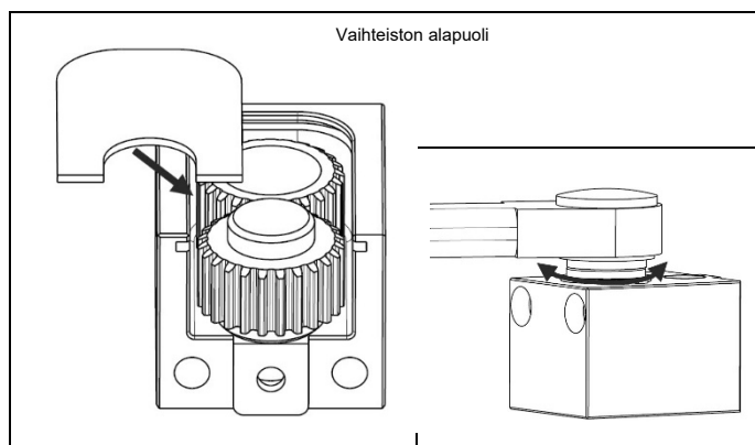
Kuva 4.23 Aseta vaihteiston kansi, tarkista, että pyörät pyörivät tasaisesti
