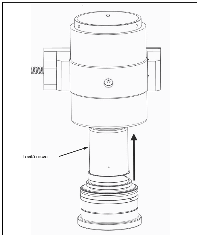
Kuva 4.7 Levitä rasva ja asenna mäntä
