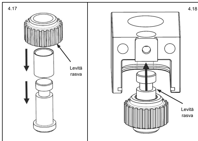
Kuva 4.17 Rasvaa ja asenna välipyörä
