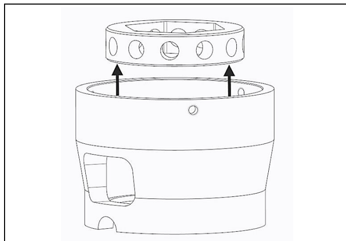
Kuva 4.9 Poista muhvi sillasta
