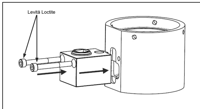
Kuva 4.24 Levitä Loctitea kiinnitysruuveihin, kiinnitä koottu vaihteisto siltaan
