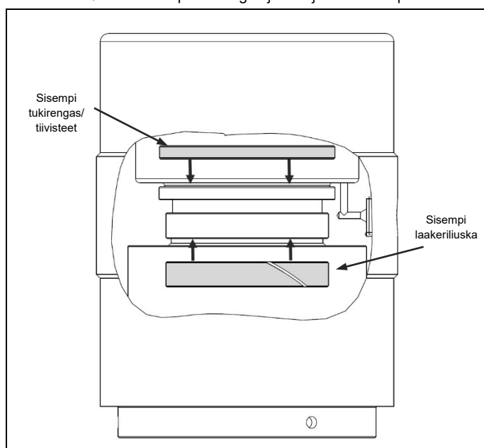
Kuva 4.6 Aseta sisempi tiiviste ja sen jälkeen sisempi tukirengas
