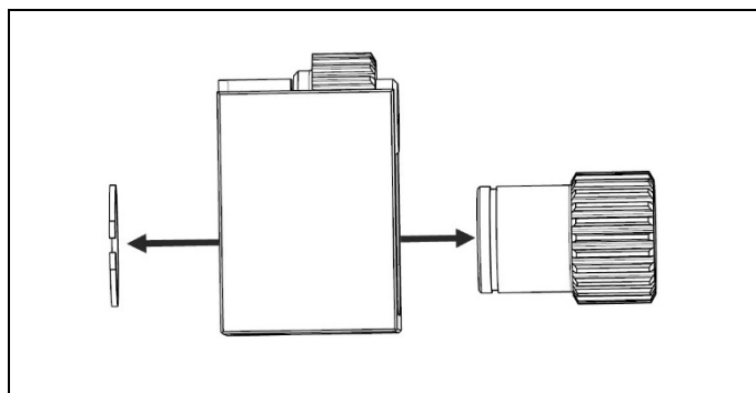
Kuva 4.12 Poista käyttöpyörän lukkorengas ja käyttöpyörä\
