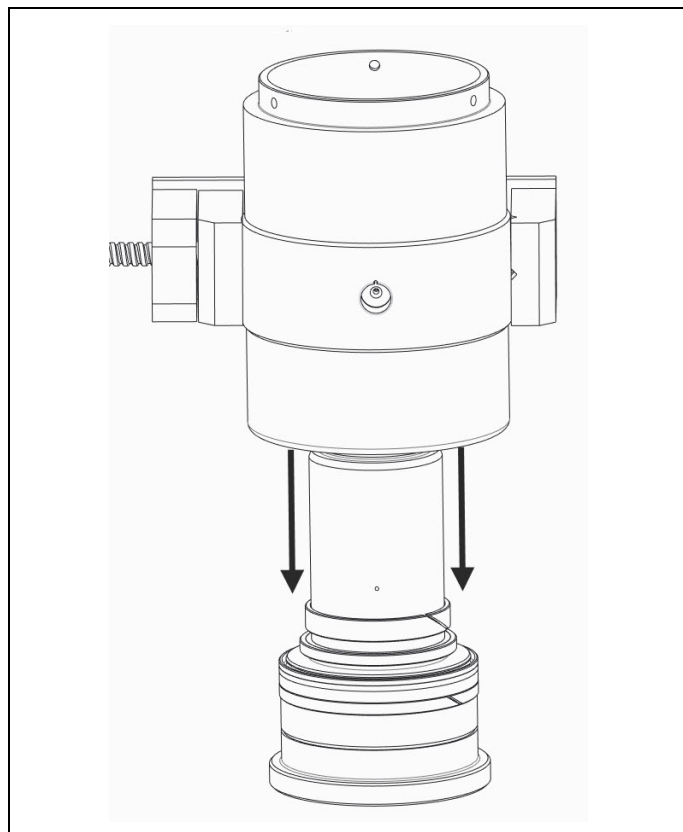
Kuva 4.3 Rungosta poistettu mäntä
