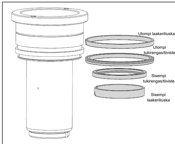
Kuva 4.4 Mäntä, ulompi tukirengas/tiiviste, sisempi tukirengas/tiiviste, laakeriliuskat
