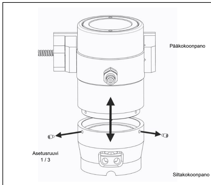
Kuva 4.1 Pääkokoonpanon ja siltakokoonpanon irrottaminen
