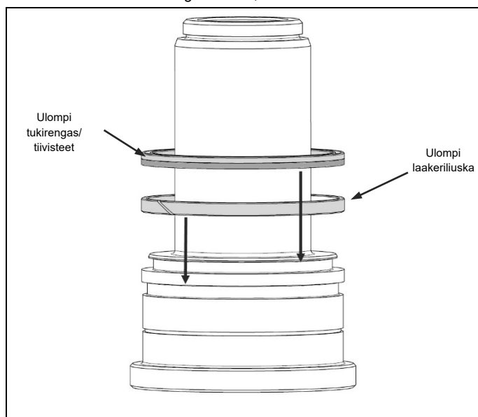
Kuva 4.5 Aseta ulompi tukirengas ja sen jälkeen ulompi tiiviste
