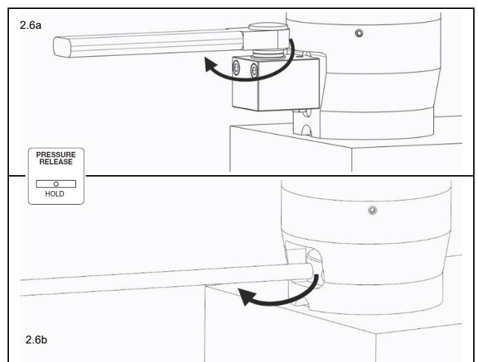
Kuva 2.6a Kiristä muhvia vaihteiston kanssa
