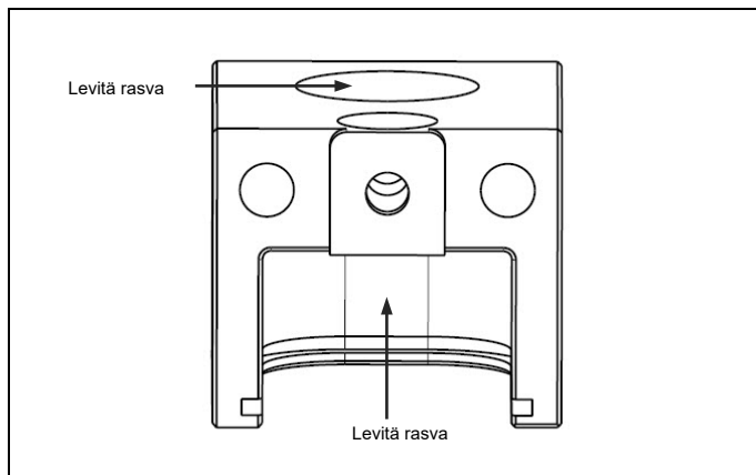
Kuva 4.16 Valmistele vaihteistokotelo
