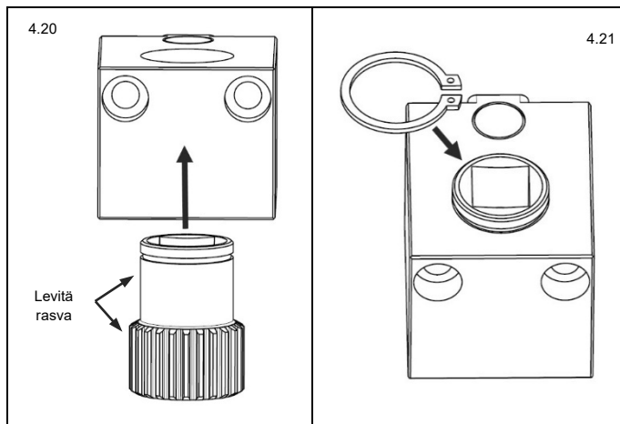
Kuva 4.20 Valmistele ja asenna käyttöpyörä
