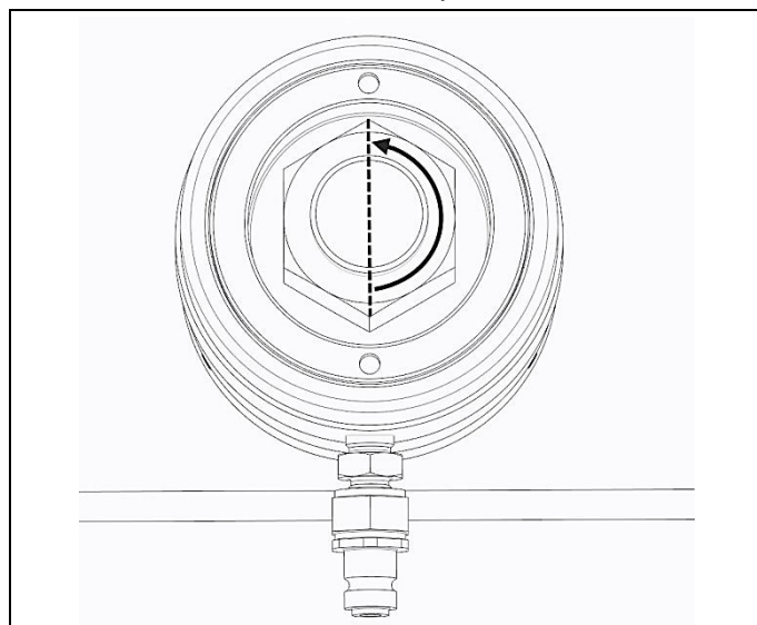
Kuva 3.1 Kiristä reaktiomutteria ja käänä takaisin ½ kierrosta
