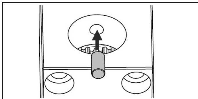
Kuva 4.19 Aseta lieriötappi paikoilleen
