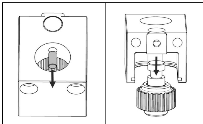
Kuva 4.13 Poista lieriötappi ja sen jälkeen välipyöräkokoonpano
