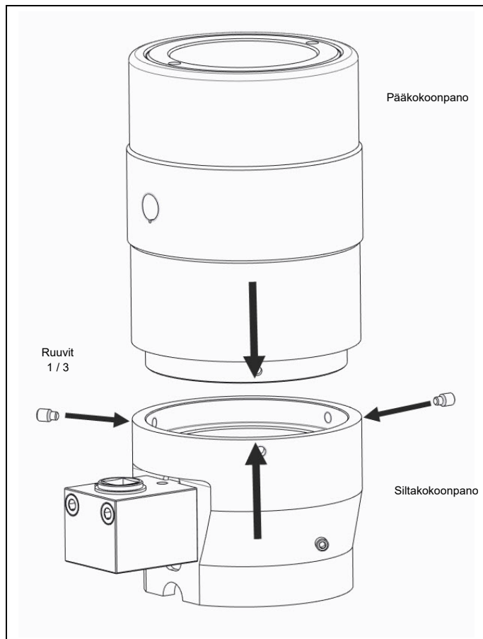
Kuva 4.26 Aseta pääkokoonpano siltakokoonpanon päälle, kiinnitä kiinnitysruuveilla
