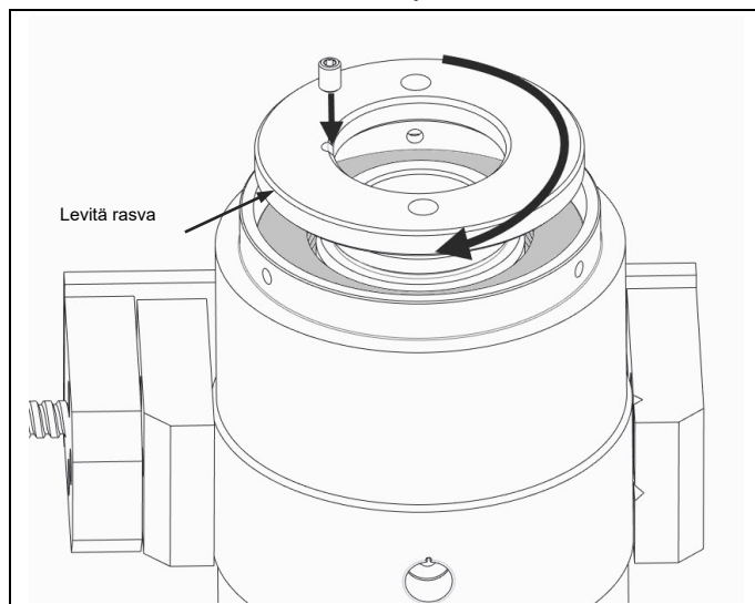
Kuva 4.8 Kierrä joustorengas paikoilleen. Kiinnitä asetusruuvilla
