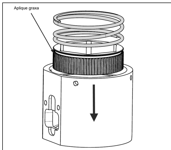
Fig. 4.15 Verifique se as peças internas da ponte se encaixam corretamente, aplique graxa
