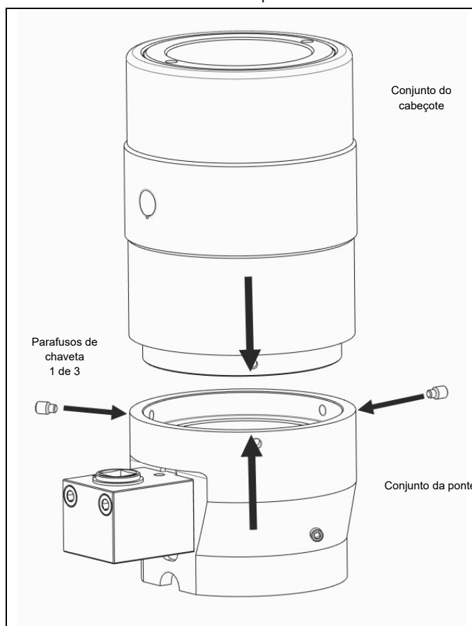
Fig. 4.26 Coloque o conjunto do cabeçote no conjunto da ponte, prenda com parafusos de chaveta
