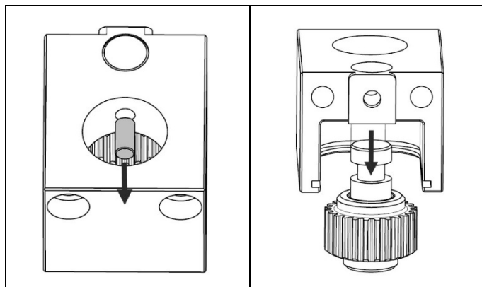
Fig. 4.13 Remova o pino de encaixe seguido pelo conjunto da engrenagem intermediária
