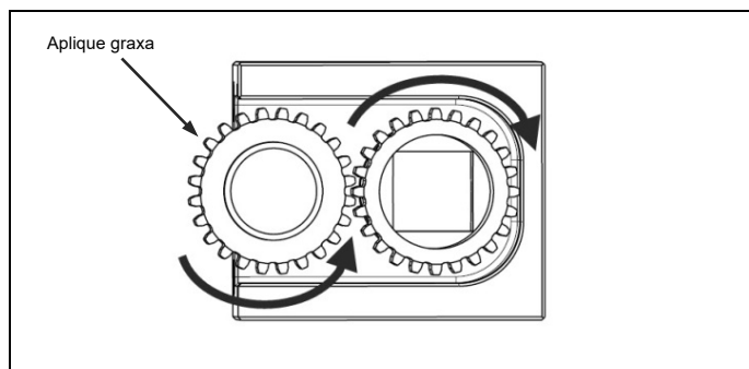
Fig. 4.22 Verifique se as engrenagens encaixadas funcionam sem problemas, aplique graxa
