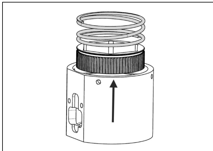
Fig. 4.14 Remova soquete dentada
