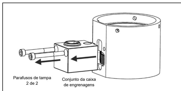
Fig. 4.10 Separação do conjunto montagem da ponte e do conjunto da caixa de engrenagens
