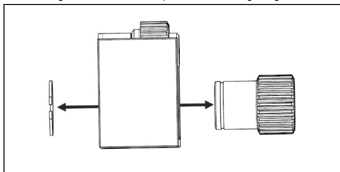
Fig. 4.12 Remova o anel de trava da engrenagem acionadora e a engrenagem acionadora
