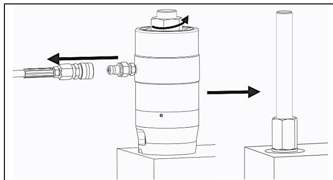
Fig. 2.8 Remova a mangueira, retire e reposicione o tensionador
