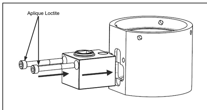
Fig. 4.24 Aplique Loctite nos parafusos de tampa, prenda a caixa de engrenagens montada na ponte
