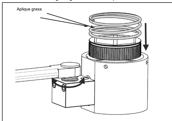
Fig. 4.25 Aplique graxa, insira o soquete dentado, seguido por molas de compressão
