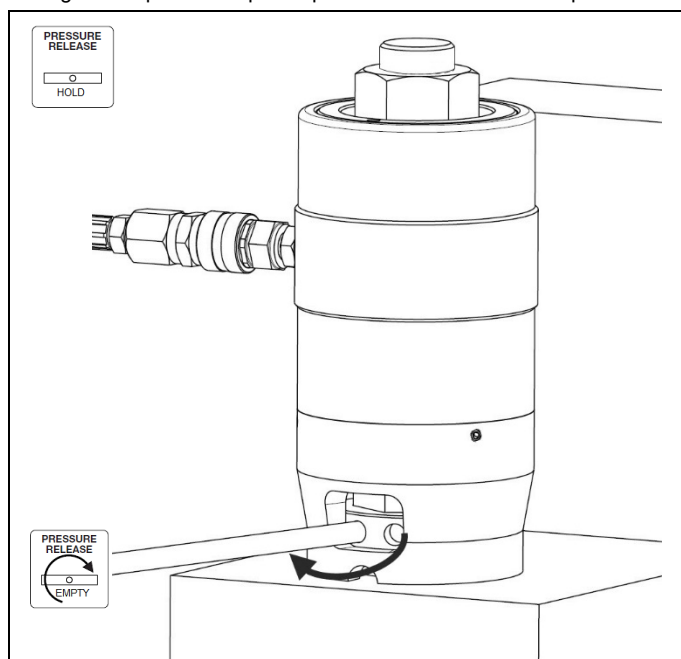
Fig. 2.7 Mantenha a pressão para apertar a porca
