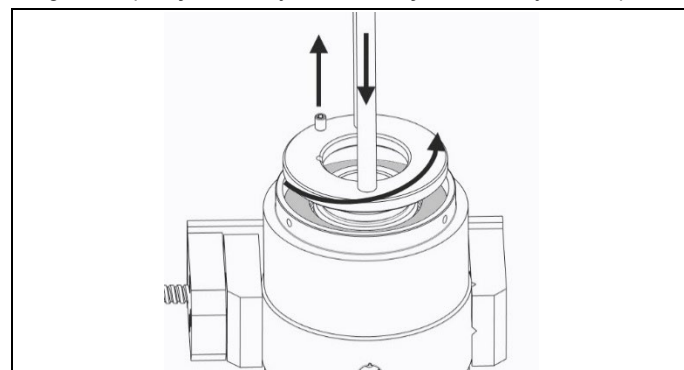
Fig. 4.2 Remova o colar da mola
