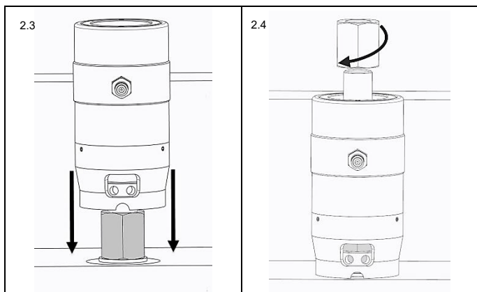
Fig. 2.3 Coloque o tensionador na aplicação
