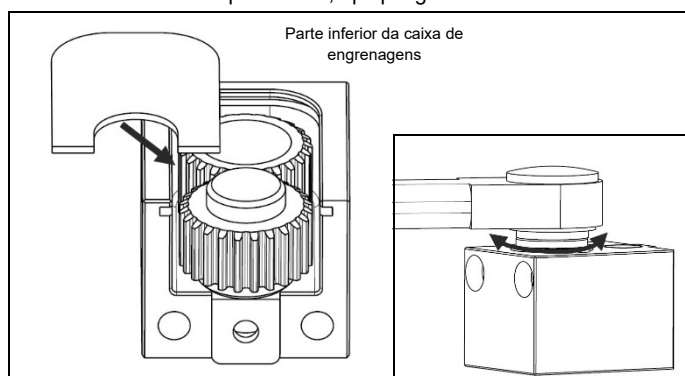
Fig. 4.23 Coloque a tampa da caixa de engrenagens, verifique se as engrenagens funcionam sem problemas
