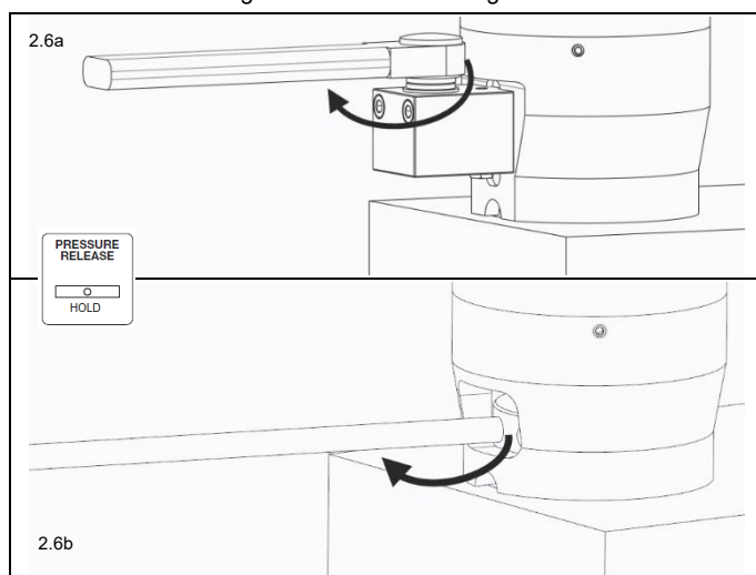
Fig. 2.6a Aperte o soquete aplicado com a caixa de engrenagens
