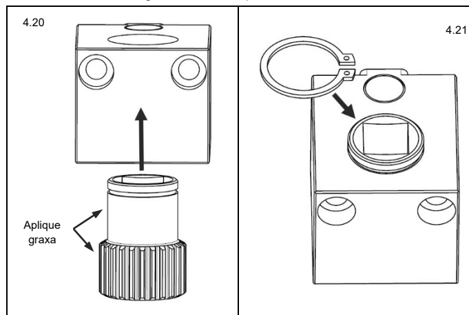
Fig. 4.20 Prepare e instale a transmissão acionadora
