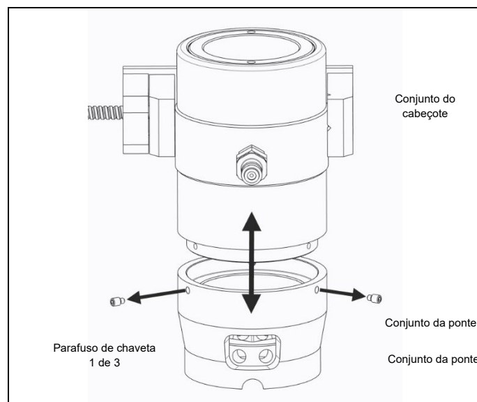
Fig. 4.1 Separação do conjunto do cabeçote e do conjunto da ponte
