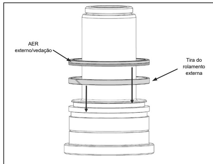
Fig. 4.5 Inserção AER externo, seguida pela vedação externa
