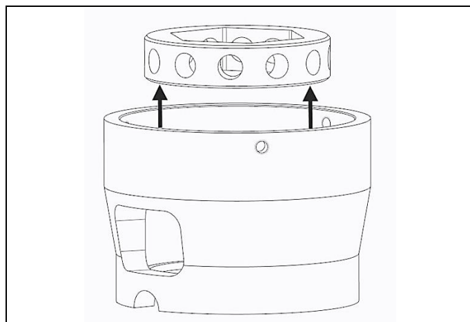
Fig. 4.9 Remova o soquete da ponte
