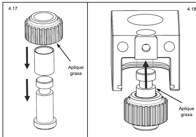
Fig. 4.17 Lubrifique e monte a engrenagem intermediária
