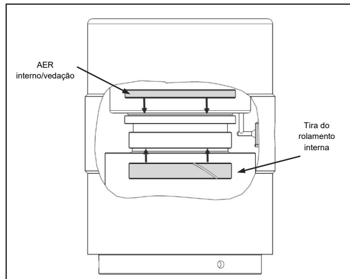
Fig. 4.6 Inserção AER interno, seguida pela AER interno
