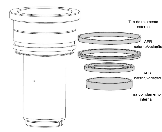
Fig. 4.4 Pistão, AER externo/vedação, AER interno/vedação, tiras do rolamento
