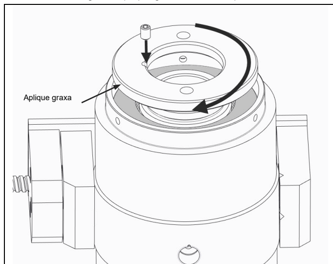
Fig. 4.8 Aparafuse o colar da mola no lugar. Prenda com parafuso de chaveta
