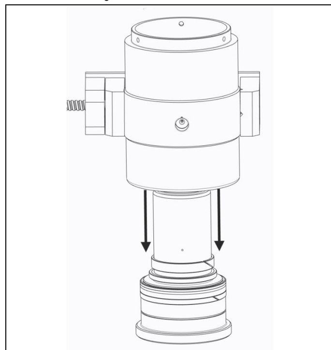
Fig. 4.3 Pistão removido do corpo
