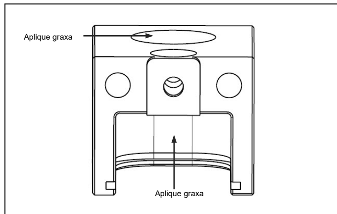
Fig. 4.16 Prepare o compartimento da caixa de engrenagens
