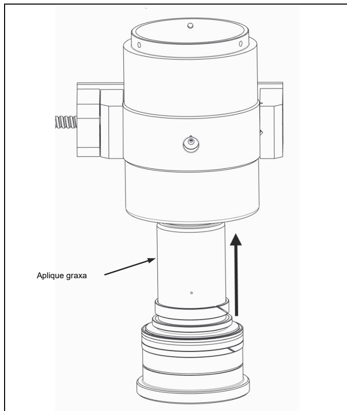
Fig. 4.7 Aplique graxa e instale o pistão
