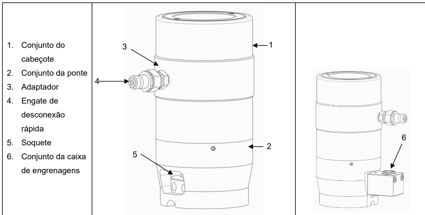
Fig. 1.1 Principais características e componentes do Tensionador redondo de fundação da Série FTR
