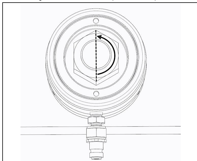
Fig. 3.1 Aperte a porca de reação e gire 1/2 volta
