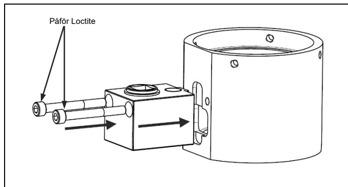
Fig. 4.24 Påför Loctite på skruvarna, fäst monterad växellåda på bryggan
