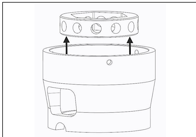
Fig. 4.9 Ta bort hylsan från bryggan
