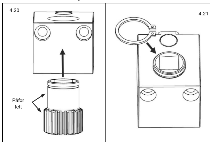
Fig. 4.20 Förbered och installera drivväxeln
