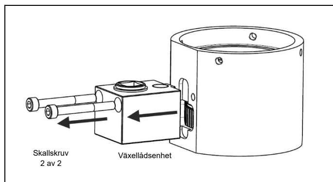
Fig. 4.10 Separering av bryggenhet och växellådsenhet
