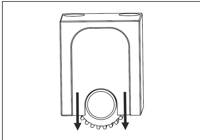
Fig. 4.11 Ta bort växellådans hölje
