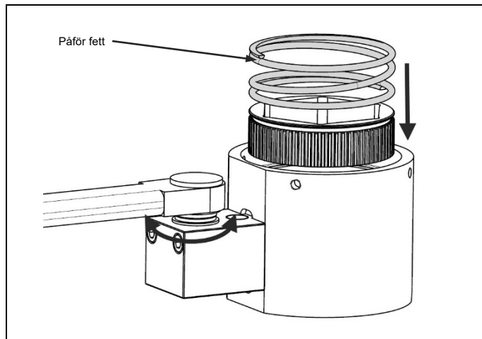
Fig. 4.25 Påför fett, sätt dit växelhylsan följt av kompressionsfjädrarna
