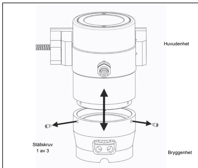
Fig. 4.1 Separering av huvudenhet och bryggenhet
