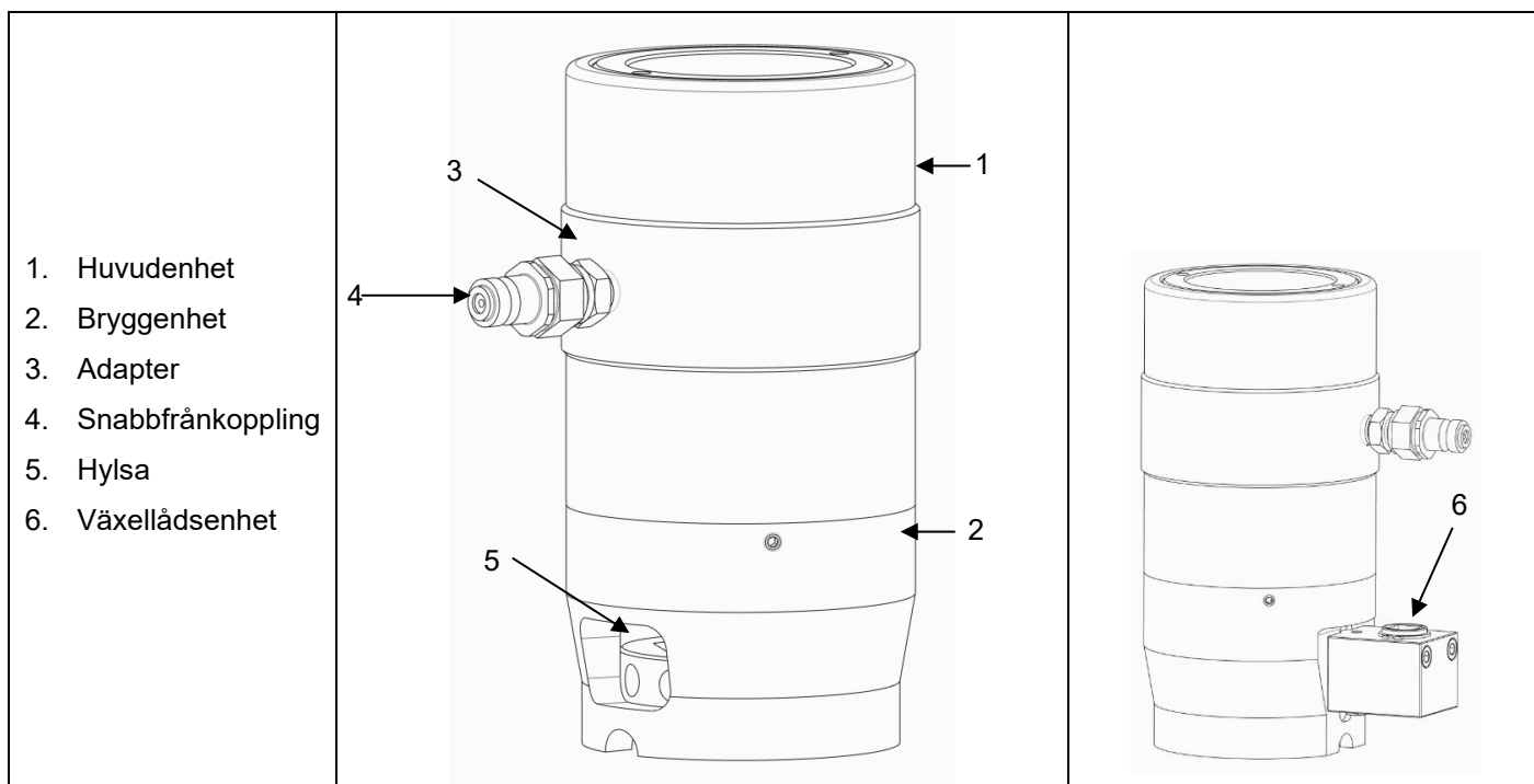
Fig. 1.1 Allmänna funktioner och komponenter i FTR-seriens runda fundamentsträckare
