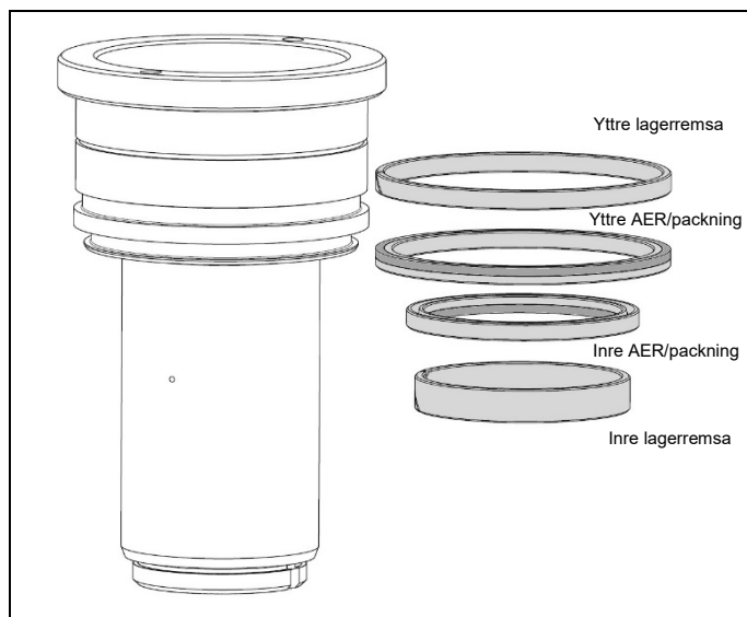
Fig. 4.4 Kolv, yttre AER/packning, inre AER/packning, lagerremsor
