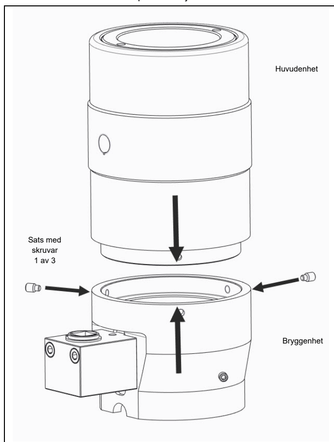
Fig. 4.26 Placera huvudenheten på bryggenheten, fäst med ställskruvar
