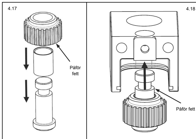
Fig. 4.17 Smörj och montera mellanväxeln
