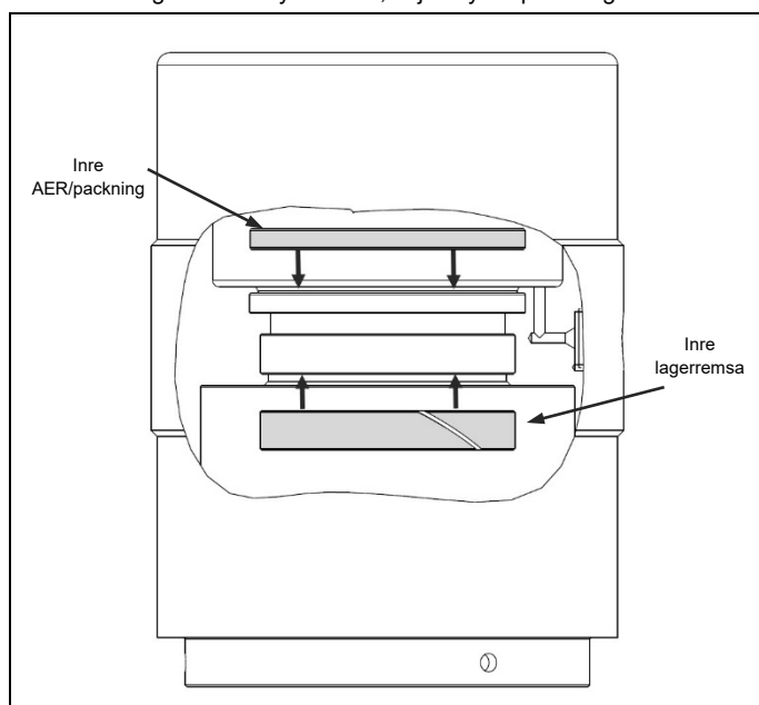
Fig. 4.6 Sätt i inre packning följt av inre AER
