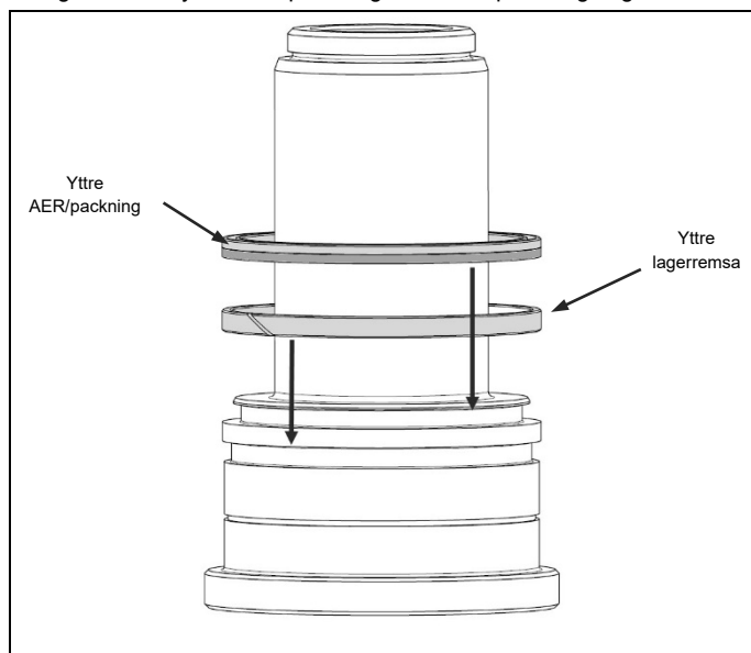
Fig. 4.5 Sätt i yttre AER, följt av yttre packningen
