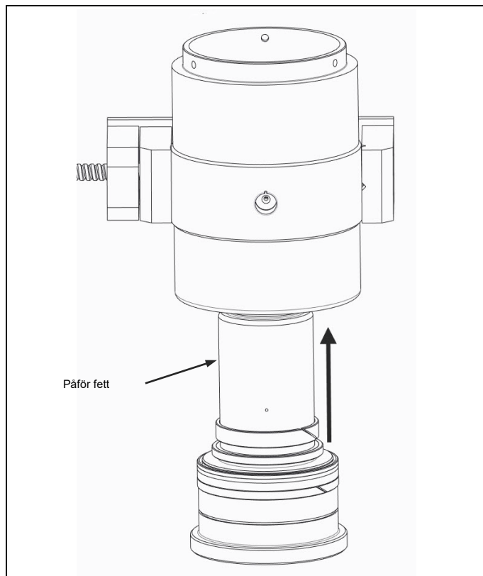
Fig. 4.7 Påför fett och montera kolven
