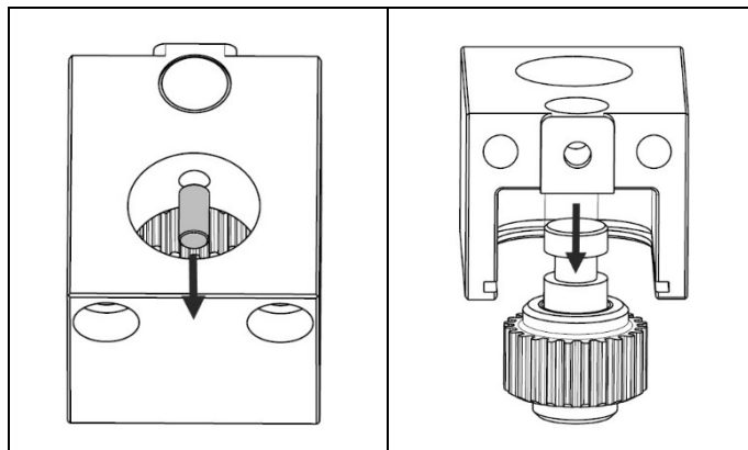
Fig. 4.13 Ta bort fäststiftet följt av mellanväxelenheten
