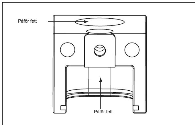
Fig. 4.16 Förbered växellådshuset
