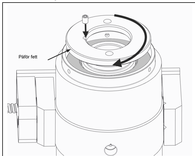
Fig. 4.8 Skruva fast fjäderkragen Fäst med ställskruv
