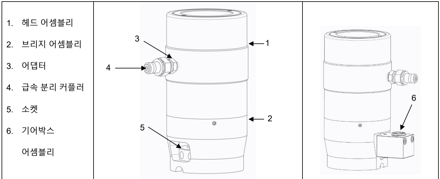
그림 1.1 FTR 시리즈 파운데이션 텐서너(원형)의 주요 기능 및 구성품
