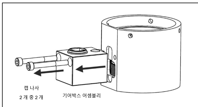
그림 4.10 브리지 어셈블리 및 기어박스 어셈블리의 분리
