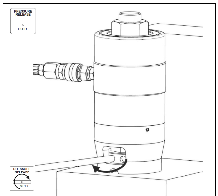
그림 2.7 압력을 유지하여 너트 조이기
