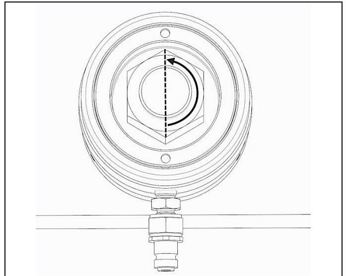
그림 3.1 리액션 너트 조이기 및 1/2 바퀴 뒤로 돌리기
