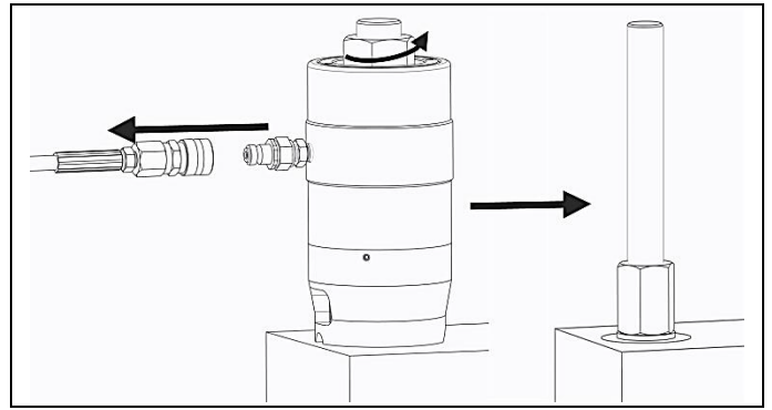
그림 2.8 호스 분리, 텐서너 제거 및 재배치
