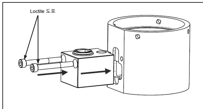
그림 4.24 캡 나사에 Loctite 도포, 조립된 기어박스를 브리지에 고정
