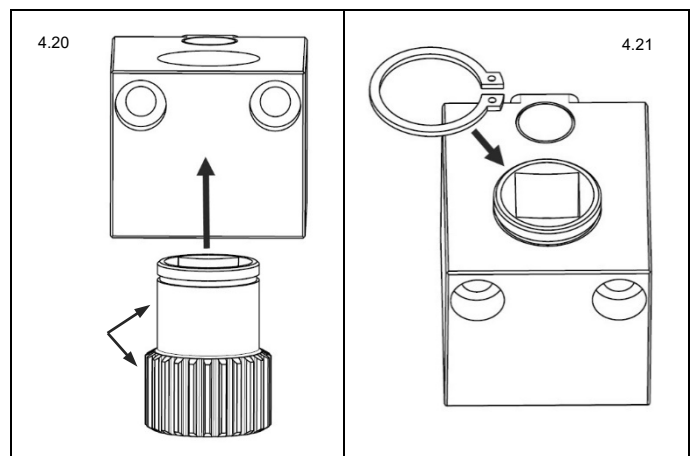
그림 4.20 드라이브 기어 준비 및 설치
