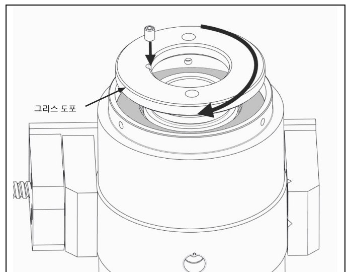
그림 4.8 스프링 칼라를 제자리에 고정. 고정 나사로 고정
