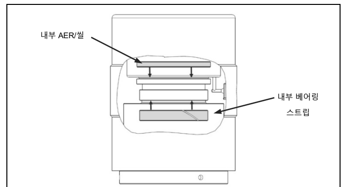
그림 4.6 내부 실 삽입 후 내부 AER 삽입
