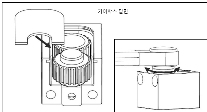
그림 4.23 기어박스 커버 장착, 기어가 원활하게 움직이는지 점검
