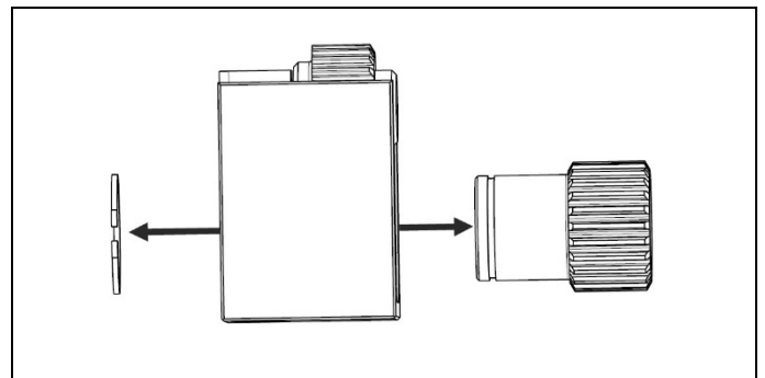
그림 4.12 드라이브 기어 서클립과 드라이브 기어 제거
