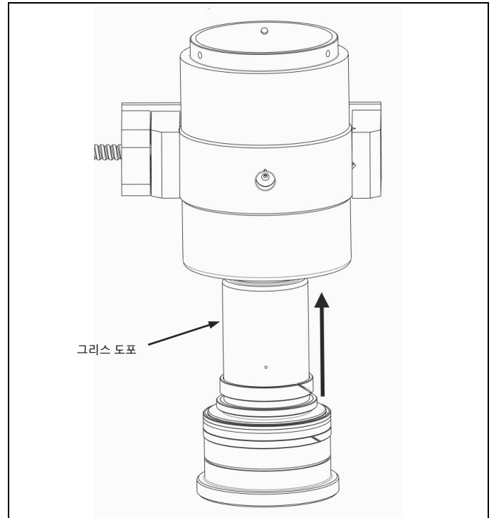
그림 4.7 그리스 도포 및 피스톤 설치
