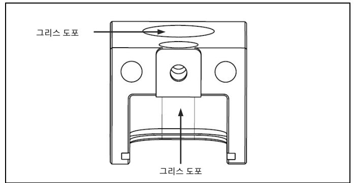
그림 4.16 기어박스 하우징 준비
