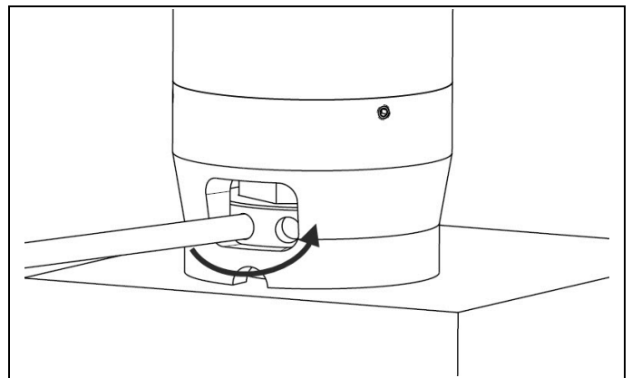
그림 3.2 리액션 너트를 시계 반대 방향으로 돌리기
