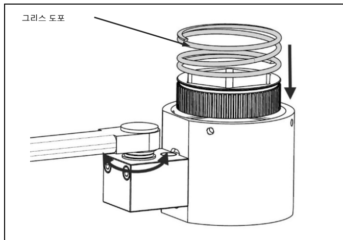
그림 4.25 그리스 도포, 기어드 소켓 삽입 후 압축 스프링 삽입
