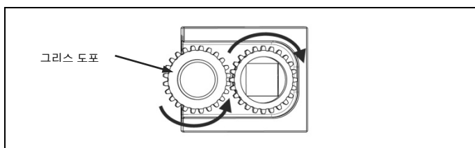
그림 4.22 장착된 기어가 원활하게 움직이는지 점검, 그리스 도포
