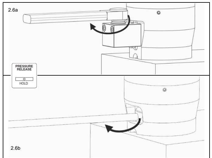
그림 2.6a 기어박스로 적용 소켓 조이기
