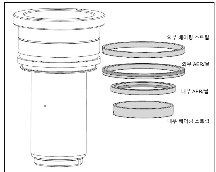
그림 4.4 피스톤, 외부 AER/실, 내부 AER/실, 베어링 스트립
