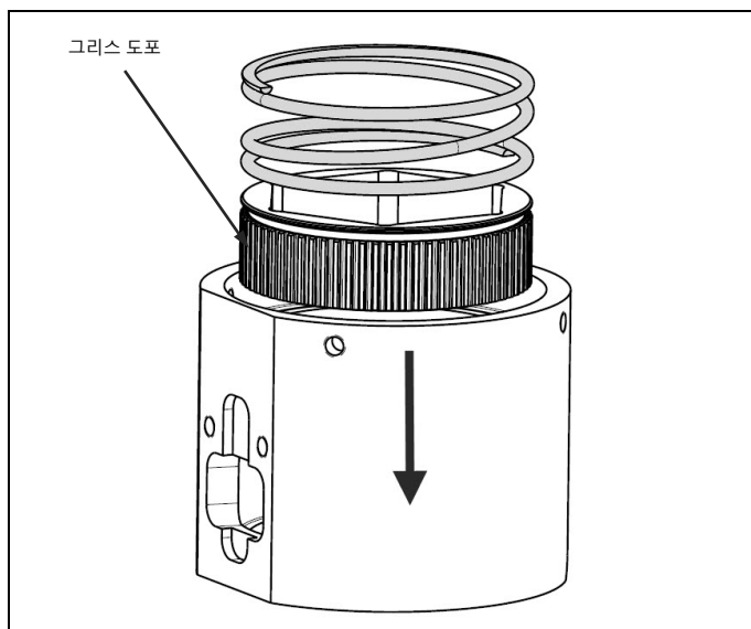
그림 4.15 브리지 내부 부품이 올바르게 맞춰졌는지 점검. 그리스 도포
