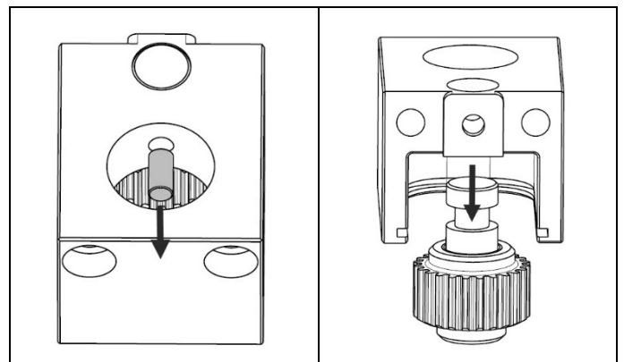
그림 4.13 고정 다웰 핀을 제거한 후 중간 기어 어셈블리 제거
