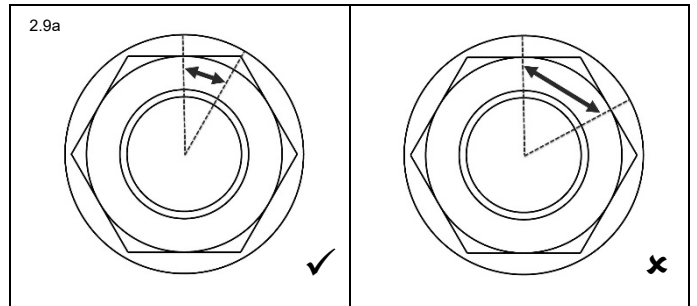
그림 2.9a 볼트 텐서닝 완성
