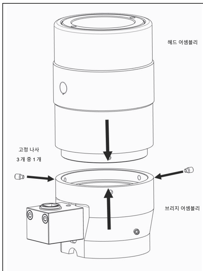
그림 4.26 헤드 어셈블리를 브리지 어셈블리에 배치, 고정 나사로 고정
