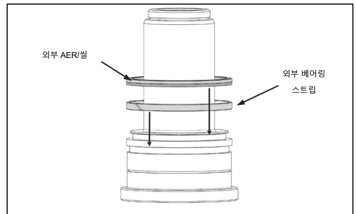
그림 4.5 외부 AER 삽입 후 외부 실 삽입
