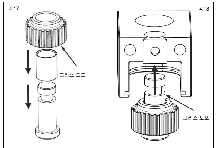
그림 4.17 중간 기어 윤활 및 조립
