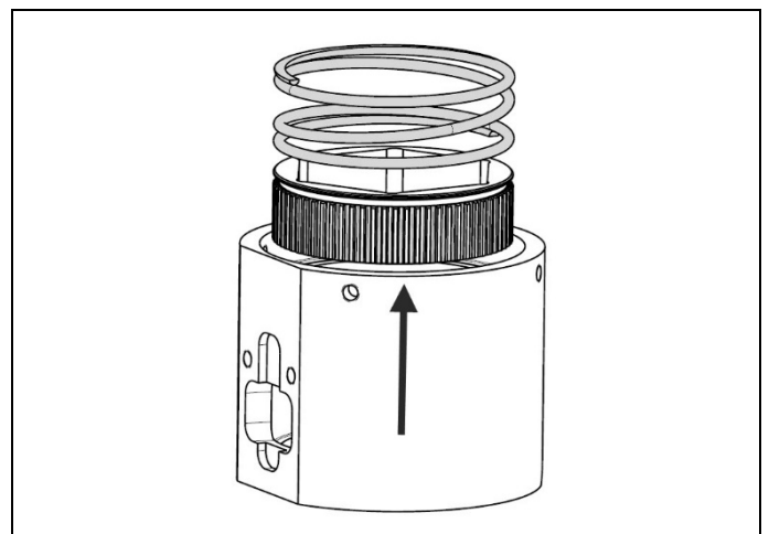
그림 4.14 기어드 소켓 제거
