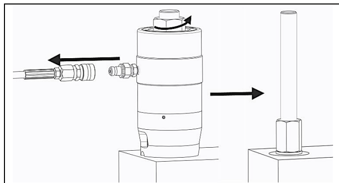
Obr. 2.8 Odpojení a hadice a přemístění napínáku
