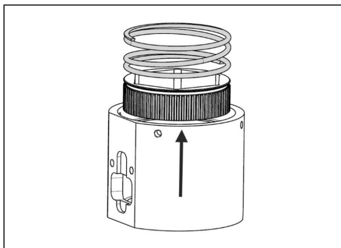
Obr. 4.14 Vyjmutí ozubené nástrčky
