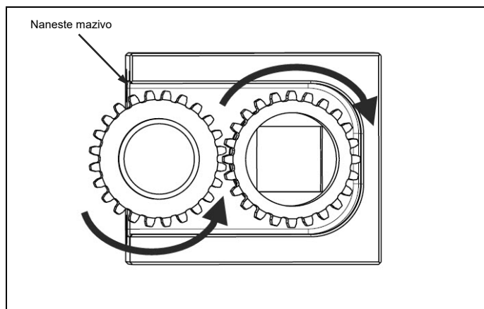
Obr. 4.22 Kontrola hladkého chodu soukolí a nanesení maziva
