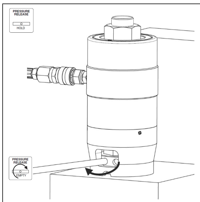
Obr. 2.6b Utažení nástrčky pomocí speciálního klíče
