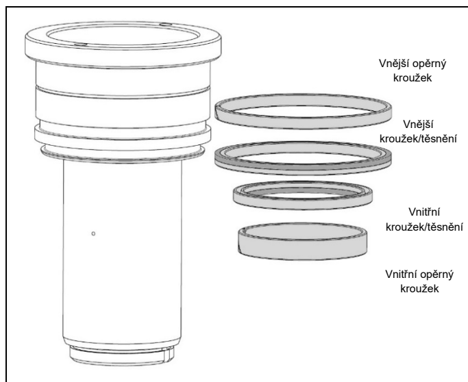
Obr. 4.4 Píst, vnější kroužek/těsnění, vnitřní kroužek/těsnění, opěrné kroužky
