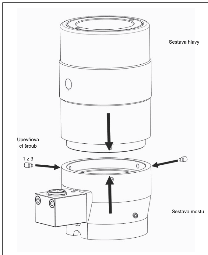
Obr. 4.26 Umístění sestavy hlavy na sestavu mostu a jejich spojení pomocí upevňovacích šroubů
