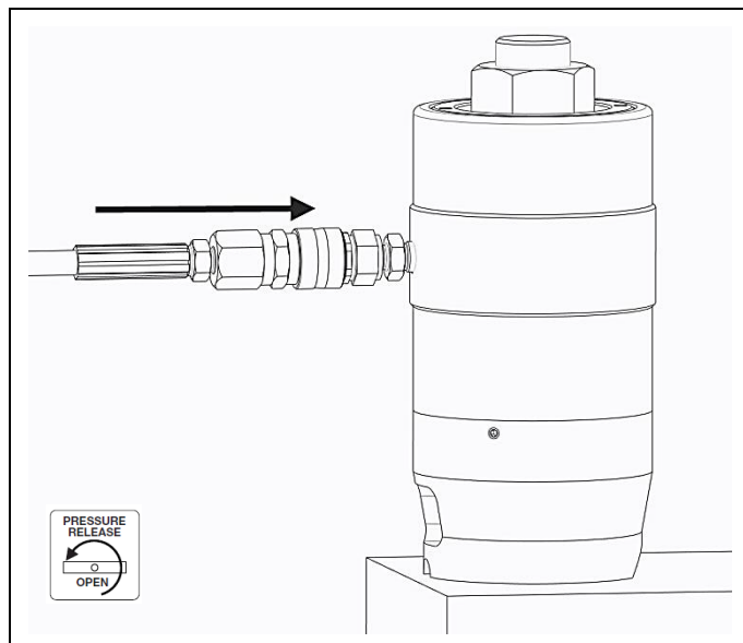
Obr. 2.5 Připojení hadice
