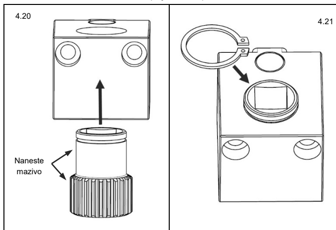
Obr. 4.20 Příprava a montáž pastorku
