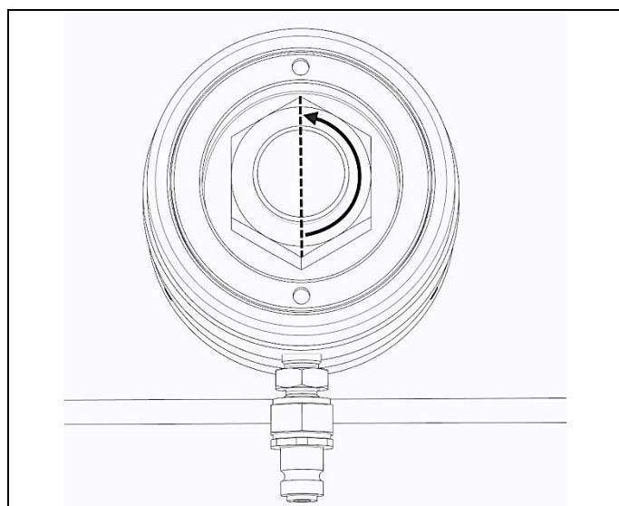
Obr. 3.1 Utažení reakční matice a následné uvolnění o 1/2 otáčky zpět
