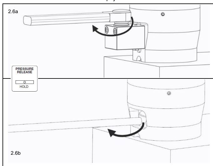
Obr. 2.6a Utažení nástrčky pomocí soukolí
