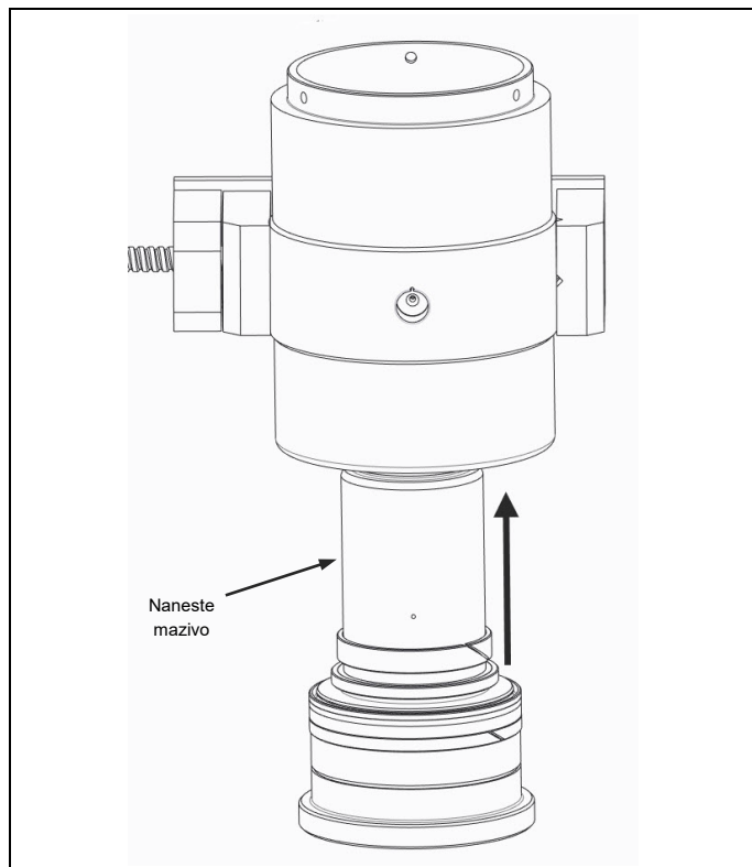
Obr. 4.7 Nanesení maziva a instalace pístu
