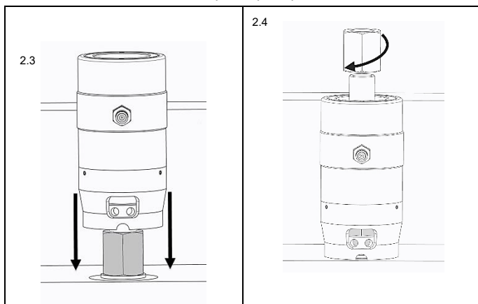
Obr. 2.3 Umístění napínáku na šroub
