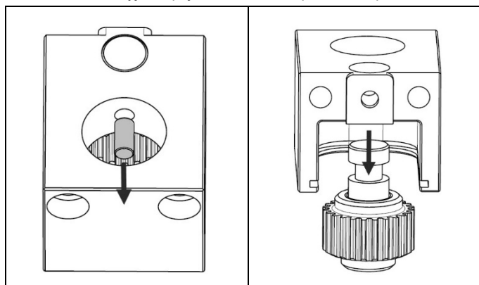
Obr. 4.13 Vyjmutí pojistného pozičního kolíku a sestavy mezilehlého kola
