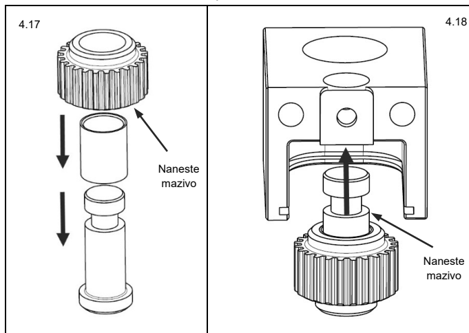
Obr. 4.17 Namazání a sestavení mezilehlého kola
