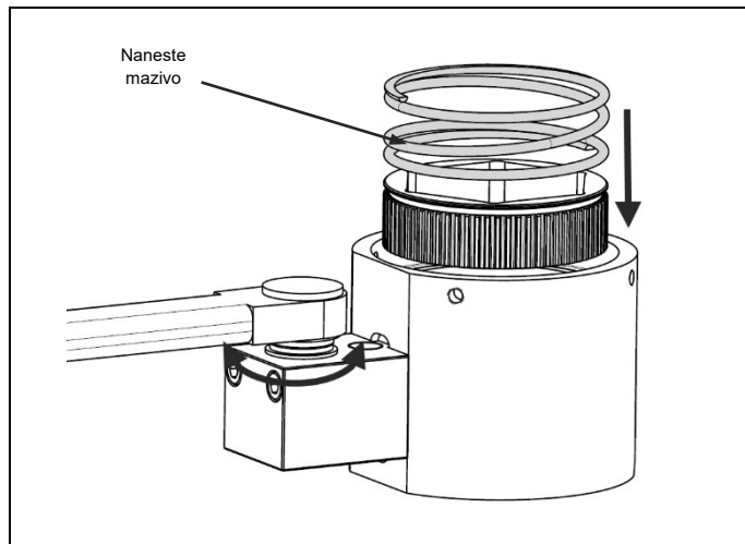
Obr. 4.25 Nanesení maziva, vložení ozubené nástrčky a následně tlačné pružiny
