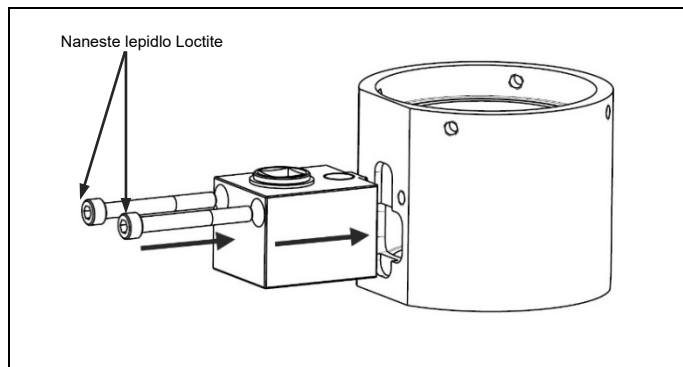
Obr. 4.24 Nanesení lepidla Loctite na upevňovací šrouby a připevnění sestavy skříně soukolí k mostu
