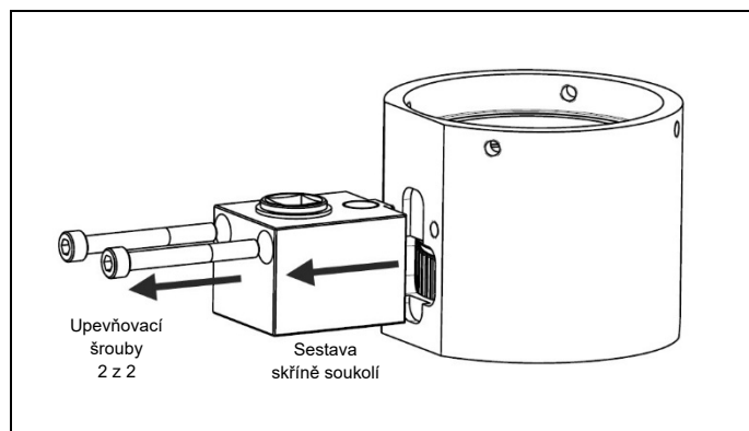
Obr. 4.10 Oddělení sestavy mostu a sestavy skříňě soukolí
