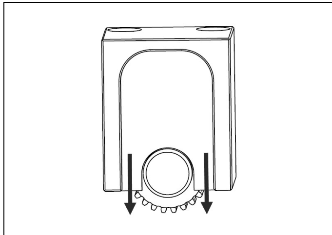
Obr. 4.11 Vyjmutí krytu skříňě soukolí
